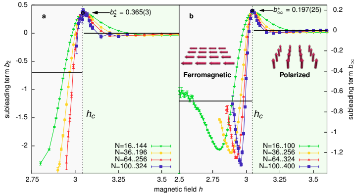
Fig. 75 Terme sous-dominant constant b_q dans le scaling de l'entropie de participation S_q (pour q = 2 et q = \infty ) pour le modèle d'Ising 2d en champ transverse. La valeur de cette constante (dans la limite thermodynamique) est universelle et permet de distinguer les phases ferromagnétique, paramagnétique (polarisée) et le point critique h_c où cette constante prend une valeur universelle non triviale b_q^* .
