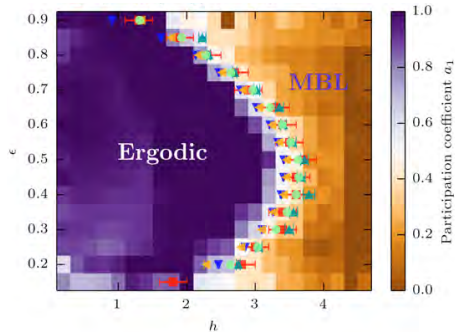
Fig. 77 Diagramme de phase densité d'énergie versus intensité du désordre pour une chaîne d'Heisenberg en champ aléatoire, obtenu à partir de divers indicateurs de taille finie [Lutz15]. La courbure de la ligne de transition séparant la phase ergodique (ETH) de la phase localisée (MBL) indique l'existence d'un seuil de mobilité à N corps dans ce modèle.
