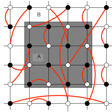
Fig. 71 L'entropie S_{VB} est définie pour un état liens de valence comme le nombre de singulets (7 sur cet exemple) traversant la frontière entre A et B (multiplié par \ln(2) ). Seuls des pavages singulets bipartites sont considérés ici.
