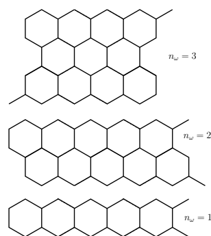
Fig. 59 Réseaux de polyacènes à n_w cycles benzéniques.
