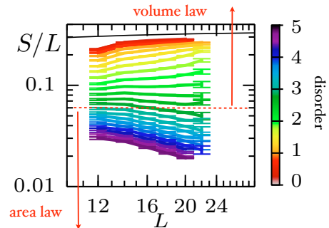
Fig. 76 Entropie d'intrication par site à mi-chaîne d'états propres du milieu du spectre d'une chaîne d'Heisenberg de taille finie L en champ aléatoire. Alors qu'à faible désordre les états du milieu du spectre suivent une loi de volume, les états dans la phase MBL (obtenue à désordre suffisamment grand) suivent une loi des aires.
