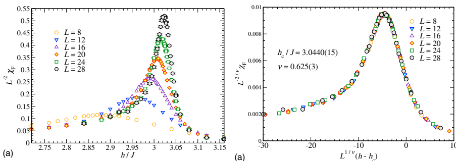
Fig. 73 Fidélité de susceptibilité \chi_F pour le modèle d’Ising 2d en champ transverse h en fonction de la taille linéaire L de l’échantillon. Le pic de la susceptibilité (panneau de gauche) signale la transition à h_c \simeq 3.04 . Une analyse d’échelle (panneau de droite) permet d’obtenir un recouvrement parfait des données, donnant accès à la classe d’universalité de la transition.
