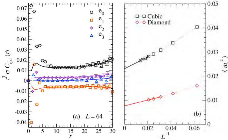
Fig. 69 La fonction |\Psi_{\text{NNVB}}\rangle présente sur les réseaux bipartites 3d à la fois un ordre antiferromagnétique à longue portée (panneau de droite, où le paramètre d'ordre tend vers une valeur finie à la limite thermodynamique) et de l'ordre dipolaire dans la fonction de corrélation dimère-dimère (panneau de gauche où l'on note la similitude totale avec la Fig. 32).
