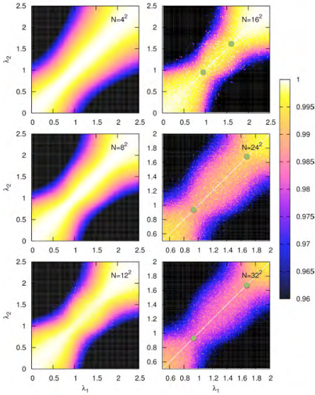
Fig. 72 Fidélité du modèle d’Heisenberg sur le réseau CaVO entre deux fondamentaux ayant des valeurs de couplage \lambda_1 et \lambda_2 . Les minima dans la fidélité révèlent les deux transitions de phase quantiques dans ce modèle (notées par des points verts pour les systèmes de plus grande taille).
