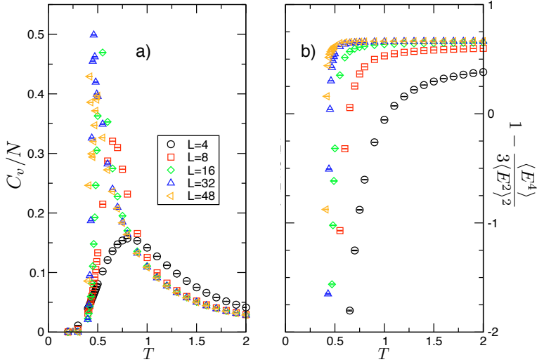
Fig. 28 En fonction de la température, pour différentes tailles de systèmes et v = 1 : a) Chaleur spécifique par site. b) Cumulant de Binder de l'énergie 1 - \langle E^4 \rangle / (3\langle E^2 \rangle^2) .
