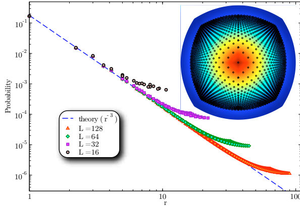
Fig. 70 Probabilité P(r) de présence d'un lien de valence entre deux spins situés à la distance r , pour le modèle d'Heisenberg antiferromagnétique en deux dimensions. L'encart figure la représentation spatiale de P(r) qui est isotrope.
