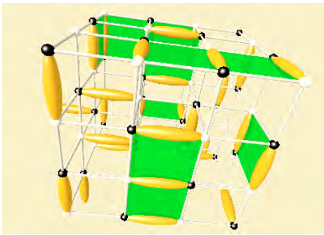
Fig. 38 Illustration du modèle de dimères en interactions sur le réseau cubique. Chaque plaquette colorée en vert possède deux dimères parallèles et contribue +v à l'énergie.
