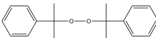
Figure 2: Structure chimique du peroxyde de dicumyle.
