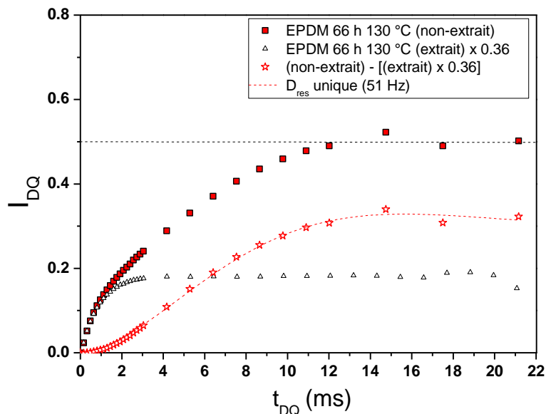
Figure 30 : Courbe de montée des cohérences DQ\ ^1H obtenue pour la matrice réticulée, non-chargée, thermo-oxydée pendant 66 h à 130 °C et non-extraite après vieillissement (■). La courbe correspondant au même échantillon, mais extrait cette fois, a été multipliée par un facteur d'échelle ( \beta = 0.36 ) ( \Delta ) puis soustraite de la courbe I_{DQ}(t_{DQ}) du matériau non-extrait.
