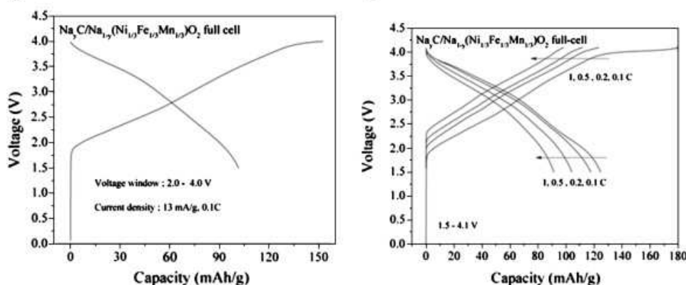
Figure 1.14. Performances de cellules Na-ion complètes \text{Na}_y\text{C} // \text{Na}_{1-y}(\text{Ni}_{1/3}\text{Fe}_{1/3}\text{Mn}_{1/3})\text{O}_2 ; ( \sim 0 < y < 0,7 (charge)) [56].
