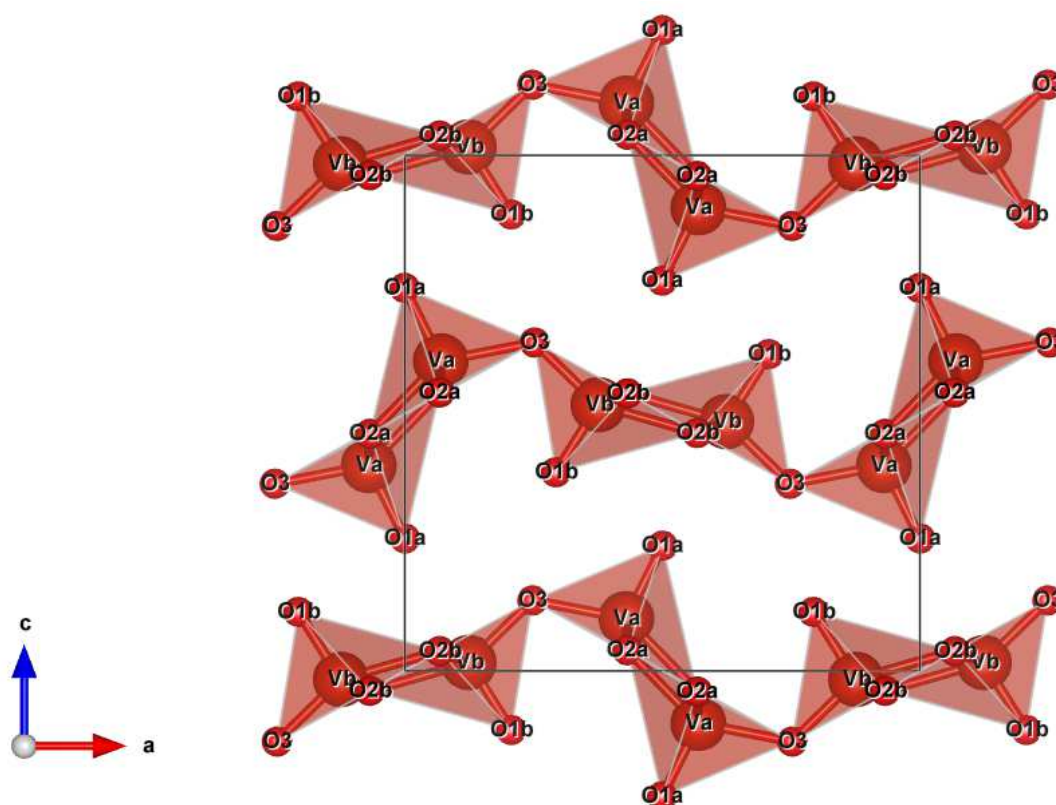
Figure 2.12. Projection dans le plan ac de la structure de \gamma -V 2 O 5 (structure orthorhombique de groupe d'espace Pnma , a = 9,9461 Å, b = 3,5852 Å et c = 10,0423 Å).
