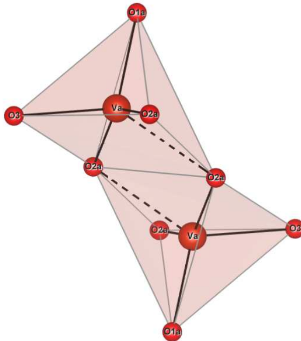
Figure 4.22. Unité principale des chaînes de V 2 O 5 dans \gamma -Na 0,97 V 2 O 5 montrant les différentes liaisons (V-O). Les contacts inter-catéennes ("ladder steps") sont indiqués par des lignes brisées.
