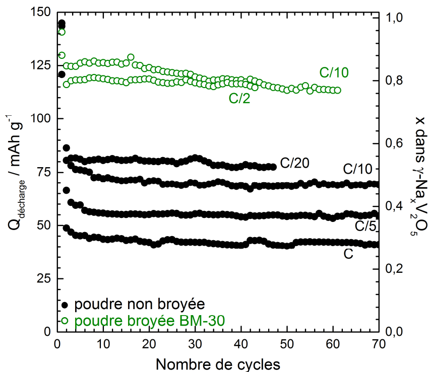
Figure 4. Evolution de la capacité spécifique en fonction du nombre de cycles de \gamma\text{'-V}_2\text{O}_5 et \gamma\text{'-V}_2\text{O}_5 - BM30. Température ambiante. Fenêtre de potentiel 1,75 - 4 V. Electrolyte 1M \text{NaClO}_4/\text{PC} .
