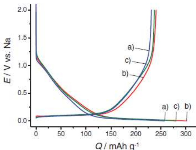
Figure 1.10. Profils de charge-décharge de carbone dur. 1M \text{NaClO}_4 dans a) EC, b) PC, c) BC butylene carbonate ( 25 \text{ mA g}^{-1} ) [44].
