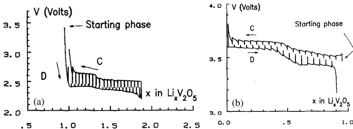
Figure 2.9. Courbes galvanostatiques de \gamma\text{-Li}_{0,95}\text{V}_2\text{O}_5 réalisées de façon intermittente avec (a) départ en réduction et (b) départ en oxydation [12].
