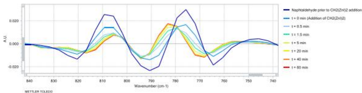
Figure 4 : Spectres IR en temps réel (conditions A) Région de la 2 ème dérivée [ 840\text{-}740\text{cm}^{-1} ]
