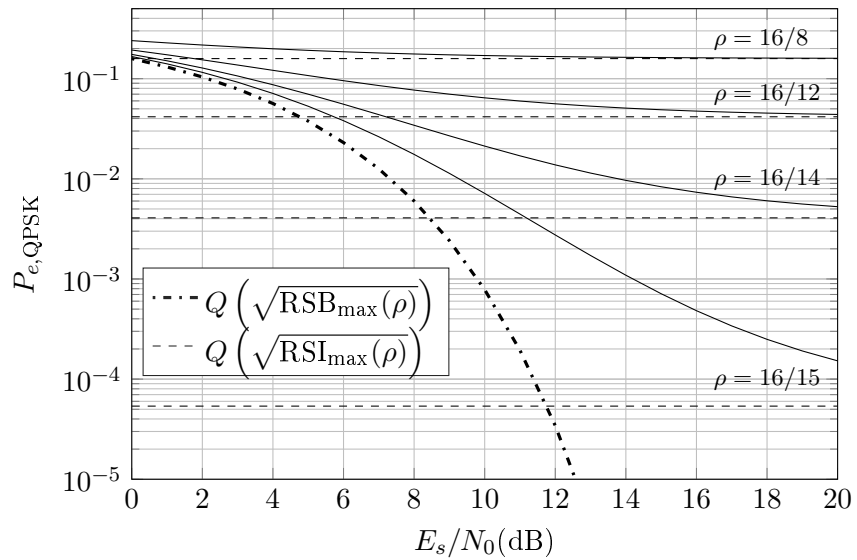
FIGURE 3.11 – Évolution de la probabilité d’erreur en fonction du rapport E_s/N_0 du système multiporteuse linéaire FTN optimal avec une constellation QPSK, et en supposant l’interférence gaussienne.
