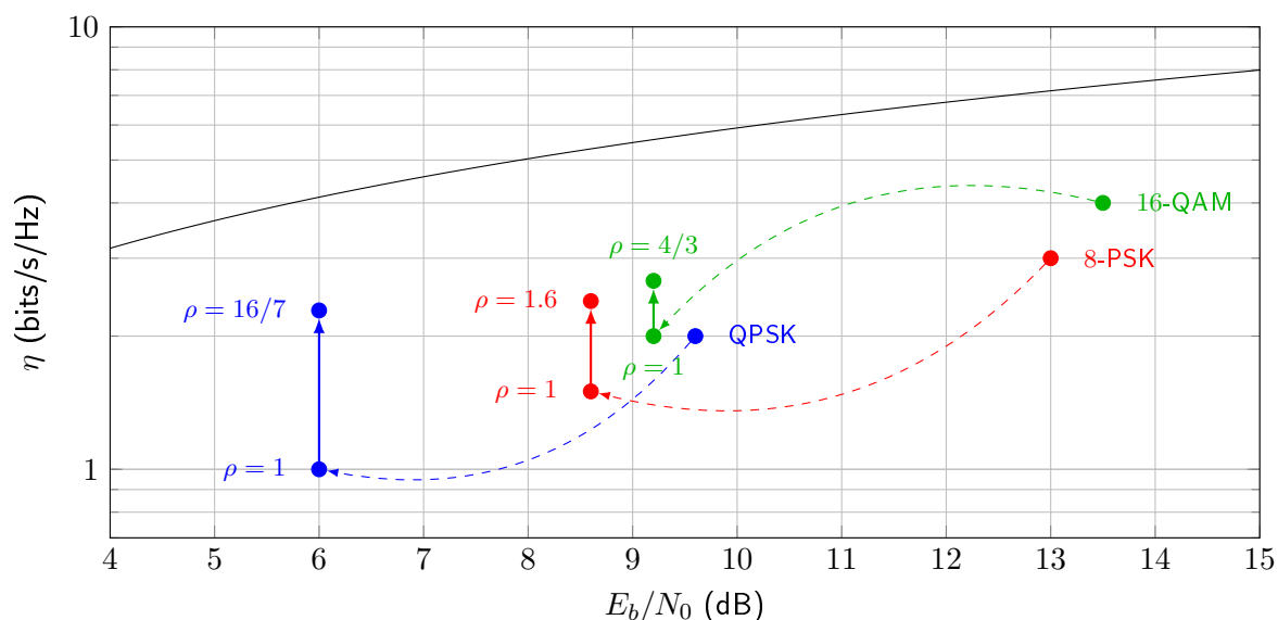
FIGURE 4.5 – Impact sur l'efficacité spectrale du système multiporteuse FTN turbo à annulation souple de l'interférence sur canal à BABG pour un TEB cible de 10^{-5} . Pour chaque constellation, trois points sont donnés. Le premier (identifié par le nom de la constellation) représente la performance du système orthogonal non-codé, le deuxième (identifié par \rho = 1 ) représente la performance du système orthogonal codé utilisant un code convolutif (7, 5), et le dernier (identifié par la valeur maximale de densité permettant la convergence du système turbo) représente la performance du système FTN turbo à annulation souple de l'interférence utilisant le code (7, 5).
