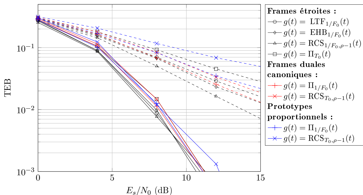
FIGURE 4.10 – Impact des prototypes d'émission et de réception sur les performances du système FTN turbo à suppression souple de l'interférence pour \rho = 1.6 , M = 4096 sous-porteuses, et en présence d'un canal COST 207 TUx6 en situation de faible mobilité ( v_{\max} = 3 km/h). Les courbes en tirets représentent la première itération du turbo-égaliseur, celles en trait plein la dixième.
