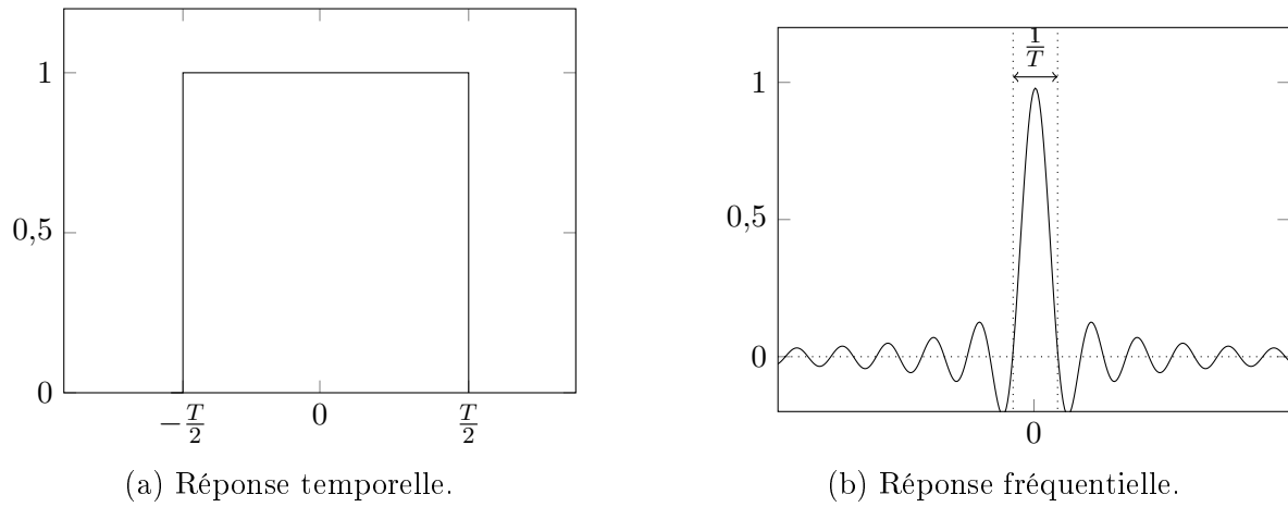
FIGURE 1.10 – Réponses temporelle et fréquentielle normalisées du prototype rectangulaire de largeur T : \Pi_T(t) .
