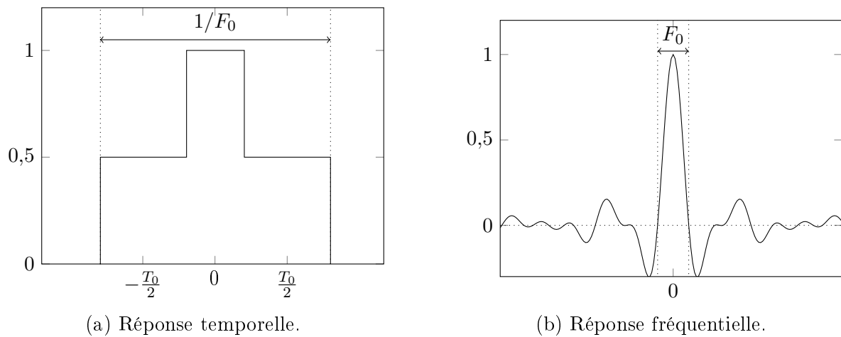
FIGURE 1.11 – Réponses temporelle et fréquentielle normalisées du prototype de la frame duale canaonique pour la frame de Gabor \mathbf{g} , de prototype g(t) = \Pi_{1/F_0}(t) et de densité \rho = 1.6 : S_{\mathbf{g}}^{-1}g(t) .
