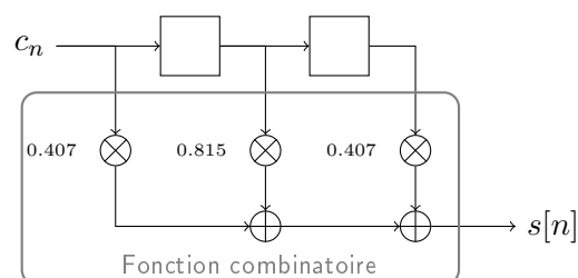
(c) Registres à décalage et fonction combinatoire.
