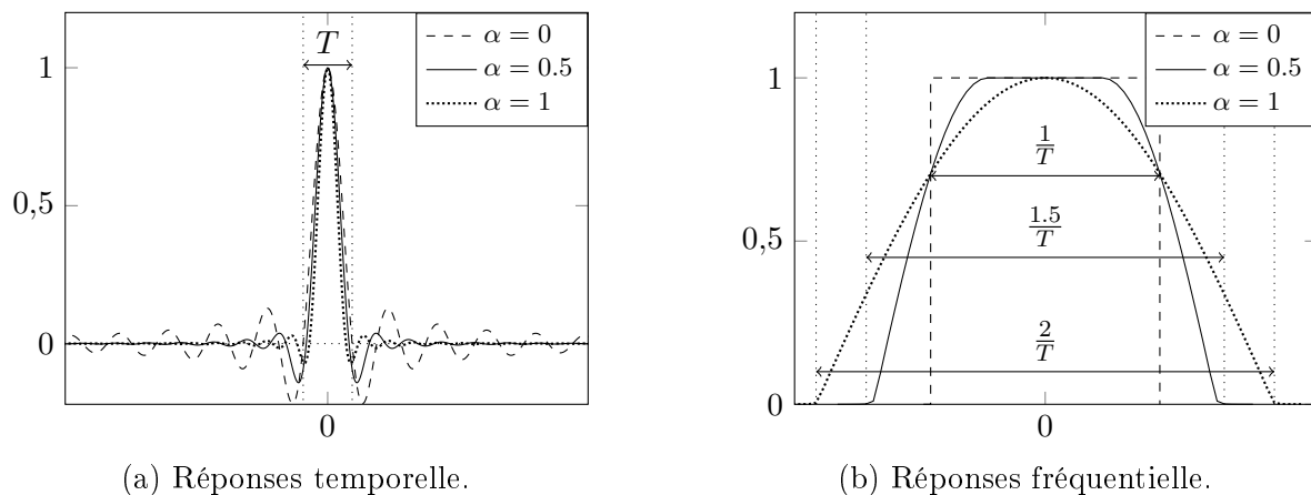
FIGURE 1.12 – Exemple de réponses temporelles et fréquentielles normalisées du prototype en racine de cosinus surélevé de support fréquentiel [-(1+\alpha)/(2T); (1+\alpha)/(2T)] : \text{RCS}_{T,\alpha}(t) .
