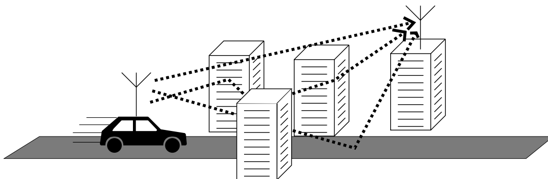
FIGURE 1.4 – Illustration d’une communication radiomobile : propagation multitrajet (plusieurs chemins de propagation entre l’émetteur et le récepteur) et effet Doppler (l’émetteur et/ou le récepteur sont mobiles).
