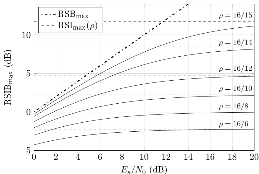
FIGURE 3.4 – Évolution du RSIB maximal avec le rapport E_s/N_0 . On remarque que lorsque ce dernier tend vers 0, RSIB_{\max} tend vers RSB_{\max} . À l'inverse, RSIB_{\max} tend rapidement vers l'asymptote horizontale RSI_{\max} lorsque E_s/N_0 augmente.
