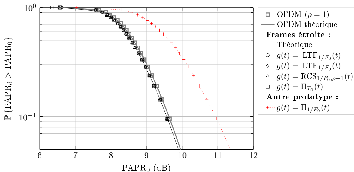
FIGURE 5.1 – Comparaison des fonctions de répartition complémentaires du PAPR discret pour différents prototypes, M = 1024 sous-porteuses et une densité \rho = 16/14 . Les courbes théoriques sont données par (5.11). On remarque la similitude du comportement en PAPR des prototypes utilisant des frames étroites, lequel est ici légèrement meilleur qu'en OFDM.
