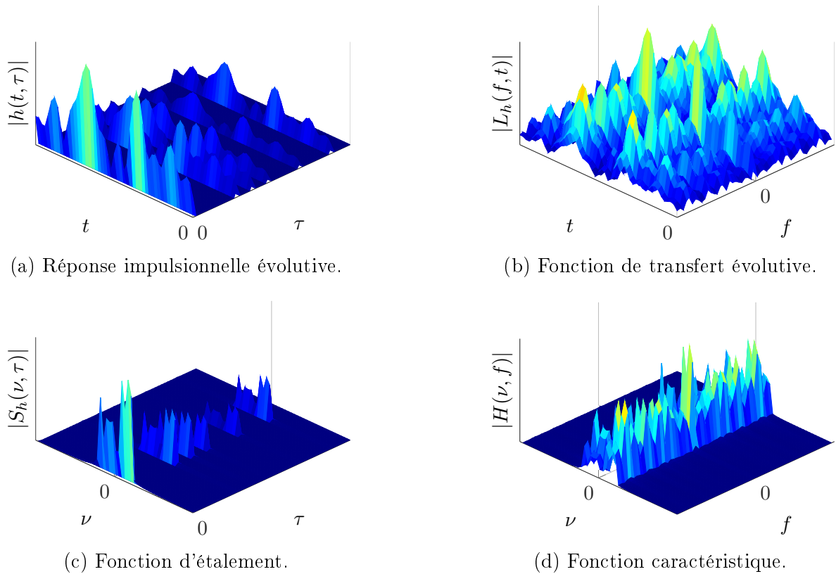
FIGURE 1.8 – Exemple de canal LTV correspondant à l'association des canaux des figures 1.6 et 1.7.
