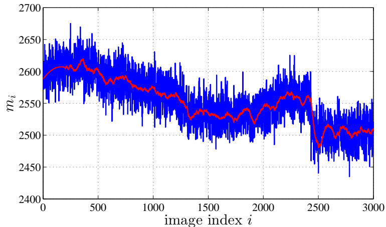
Figure 8.7: Exemple réel de la variation de la valeur moyenne avec un changement brusque à l'indice 2434.
