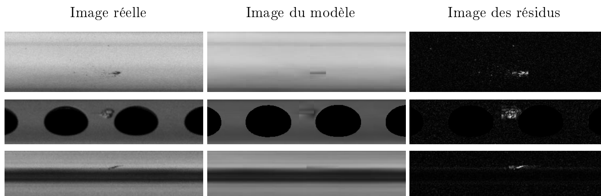
Figure 8.5: Images de roues contenant différents défauts, avec l'image du modèle de l'arrière-plan, et l'image résiduelle
