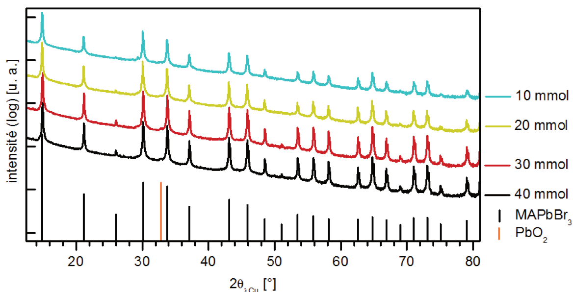
Figure 3.9. Diffractogrammes des nanocristaux hybrides \text{MAPbBr}_3 synthétisés à partir de 10, 20, 30 mmol (expériences de contrôle) ou 40 mmol de \text{PbBr}_2 .
