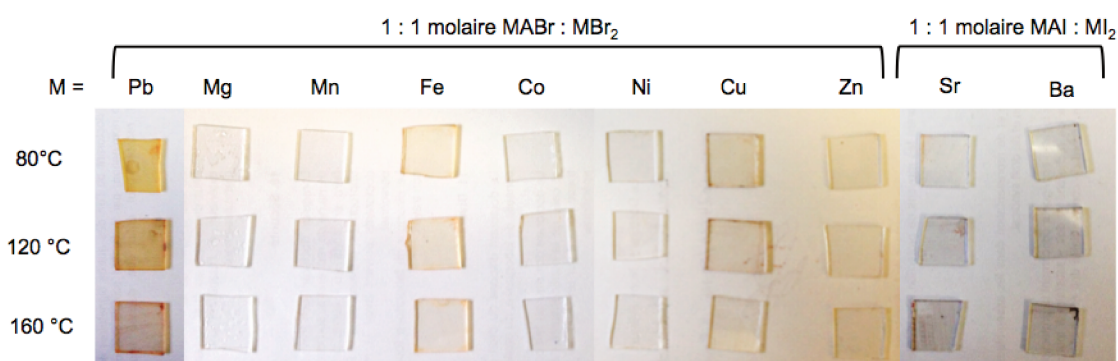
Figure 3.3. Photographie des films hybrides \text{MAPbBr}_3 et sans plomb déposés sur un substrat de verre à partir d'une solution de précurseurs \text{MAX} : \text{MX}_2 avec un ratio molaire 1 : 1 ( \text{M}^{2+} = \text{Pb}^{2+} ; \text{Mn}^{2+} ; \text{Fe}^{2+} ; \text{Co}^{2+} ; \text{Ni}^{2+} ; \text{Cu}^{2+} ; \text{Zn}^{2+} ; \text{Mg}^{2+} et \text{X}^- = \text{Br}^- ; \text{I}^- ).
