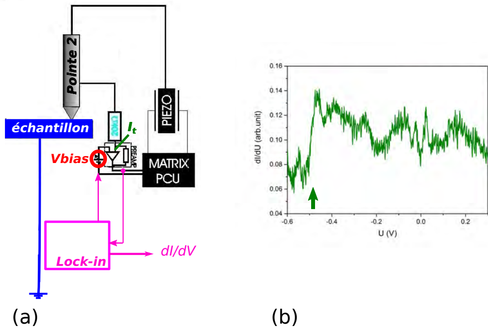
FIGURE 4.10 – En (a), schéma du lock-in ajouté au montage électronique du chapitre précédent. En (b), courbe dI/dV réalisée sur la surface d'or nous permettant d'estimer la position énergétique de l'état de surface (flèche verte).
