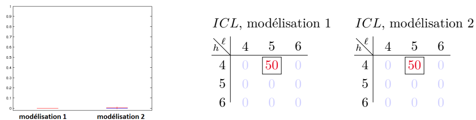
Figure 4.3 – Erreur de classification croisée sur 50 matrices (à gauche) et répartition du nombre de classes en ligne et en colonne sélectionné par la procédure Bi-KM1 (à droite) selon le type de modélisation.
