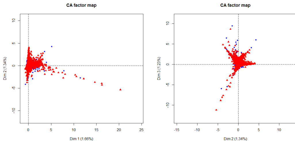
Figure 5.5 – Représentation simultanée des deux nuages profils lignes (médicaments symbolisés par des points) et profils colonnes (effets indésirables symbolisés par des triangles) dans le premier plan factoriel (à gauche) et deuxième plan factoriel (à droite) de l'AFC.
