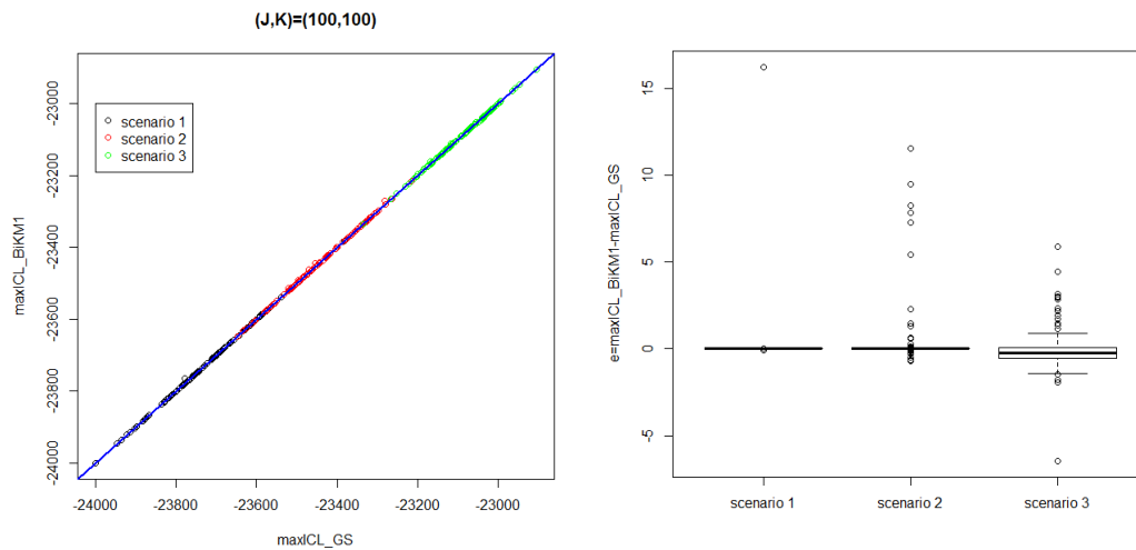
Figure 4.17 – Comparaison des valeurs maximales d' ICL renvoyées par la procédure GS (en abscisse) et par la procédure Bi-KM1 (en ordonnée) et boxplot des différences des valeurs renvoyées par les procédures suivant 3 scénarios pour la taille d'échantillon : (100, 100) .
