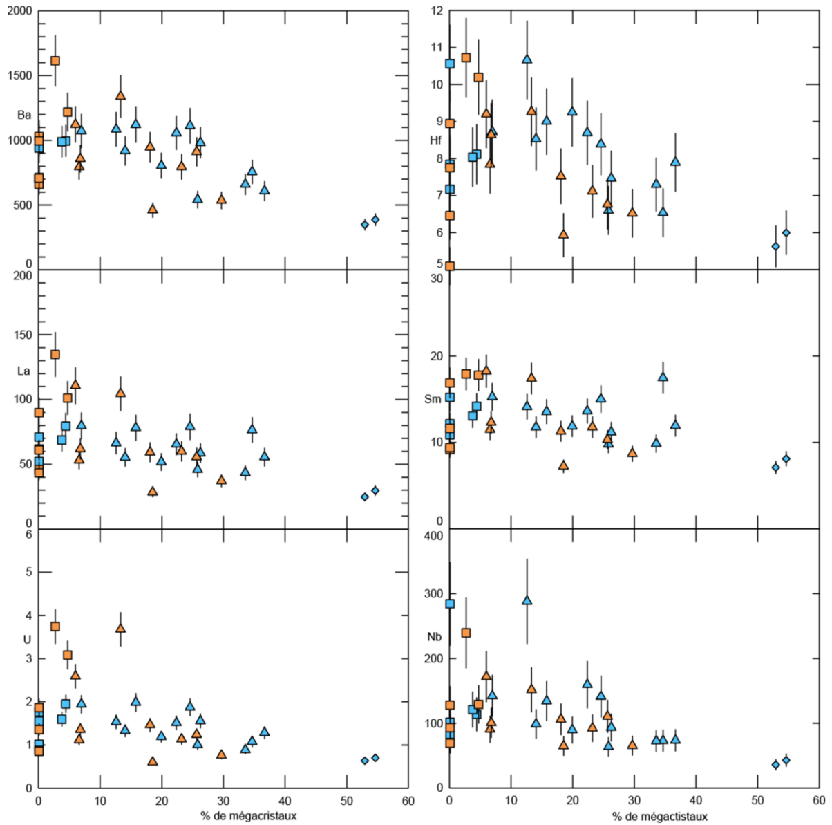
Figure 4.9: Teneurs (en ppm) de différents éléments en traces en fonction de la proportion de mégacristaux (pyroxènes, olivines et amphiboles).
