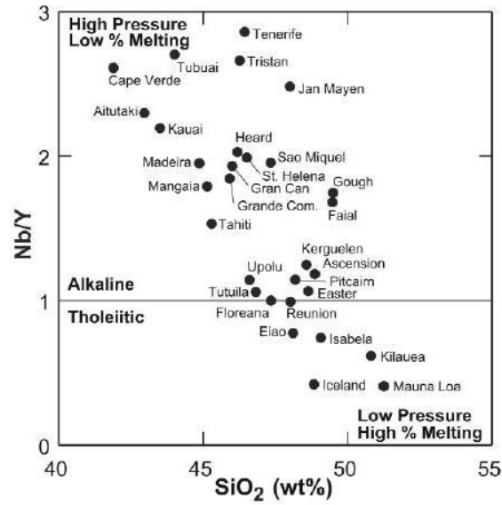
Figure 1.6 : Nb/Y versus SiO 2 dans les OIB ( Ocean Island Basalts ), illustrant la différence entre les basaltes alcalins et les tholéiites en terme de pourcentage et de profondeur (pression) de fusion. D'après Greenough et al. (2005).
