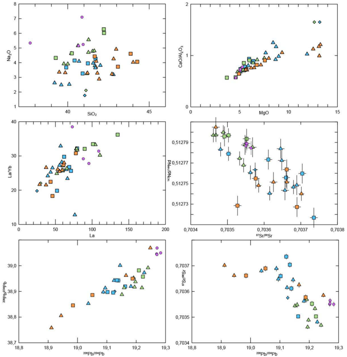
Figure 4.15 : Diagrammes présentant les différentes analyses chimiques des roches totales. En vert sont représentés les échantillons dont la chronologie relative indique qu'ils se sont mis en place dans une période proche de l'effondrement. Les autres symboles sont les mêmes que précédemment. Il est à noter que ces échantillons sont toujours présents sur une extrémité des diagrammes.
