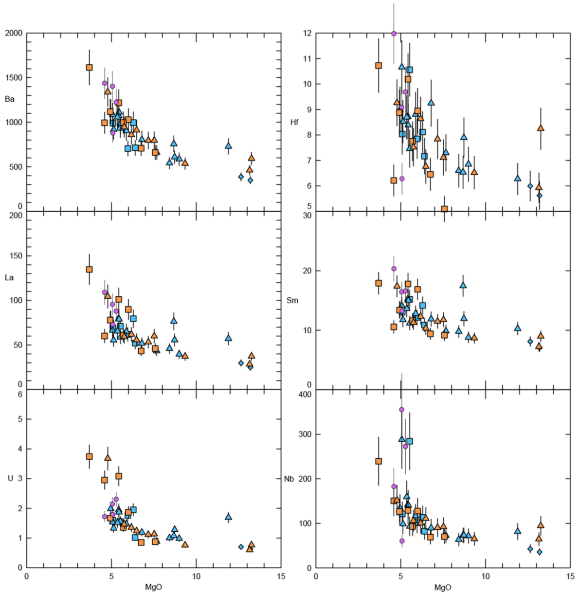
Figure 5.2 : Variation des teneurs en Ba, U, Nb, Hf, La et Sm (ppm) en fonction de MgO (pds.%) dans les laves de Fogo. On observe systématiquement une co-variation négative entre le magnésium et les différents éléments en traces, que ce soit pour les échantillons post ou pré-effondrement, qui traduit l'influence des processus de cristallisation fractionnée et d'accumulation d'antécristaux.
