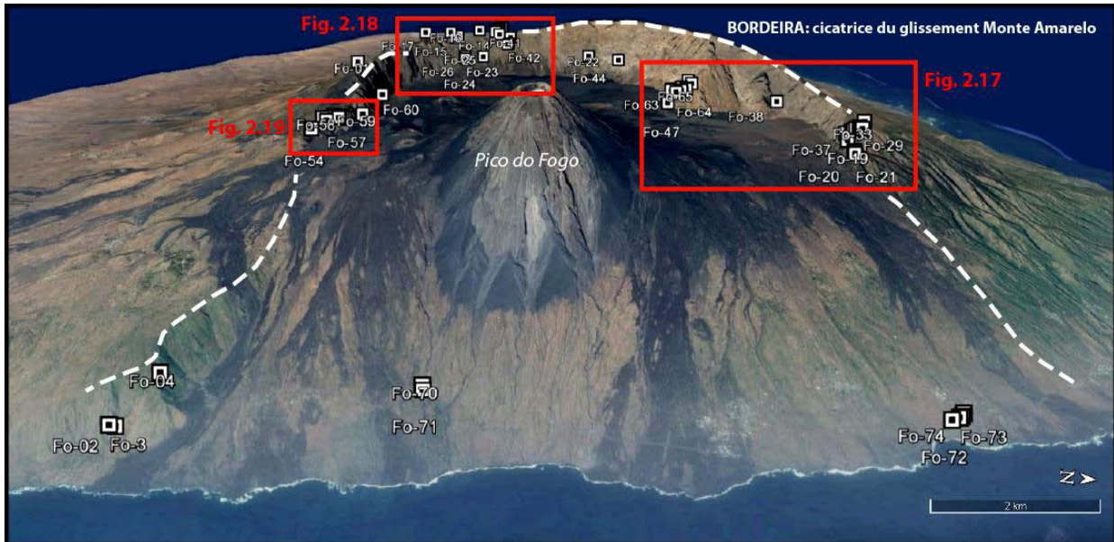
Figure 2.16 : Carte de l'échantillonnage dans la caldera de Fogo (Cap Vert), cicatrice d'une déstabilisation massive de l'édifice volcanique Monte Amarelo. Les échantillons pré-collaps sont situés sur les parois de la caldera (Bordeira), tandis que les échantillons post-effondrement fossilisent la paroi ou remplissent la cicatrice de glissement.
