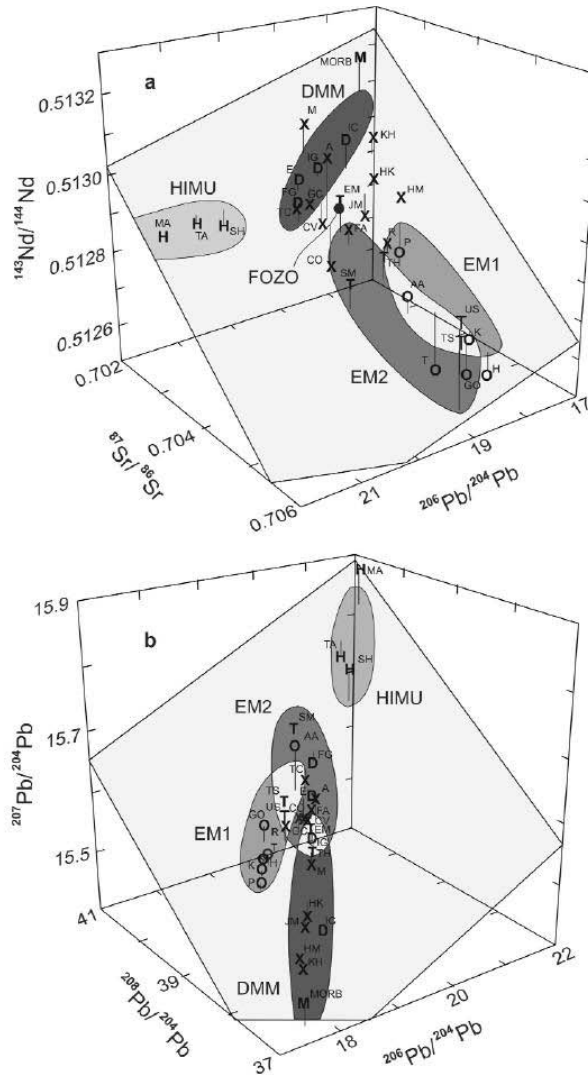
Figure 1.7 : Rapports isotopiques Pb, Sr, Nd des OIB. DMM : Depleted MORB Mantle ; EM1 : Enriched Mantle 1 ; EM2 : Enriched Mantle 2 ; HIMU : high μ ( \mu=238\text{U}/204\text{Pb} ) ; FOZO : Focal Zone composition . D'après Greenough et al. (2005).
