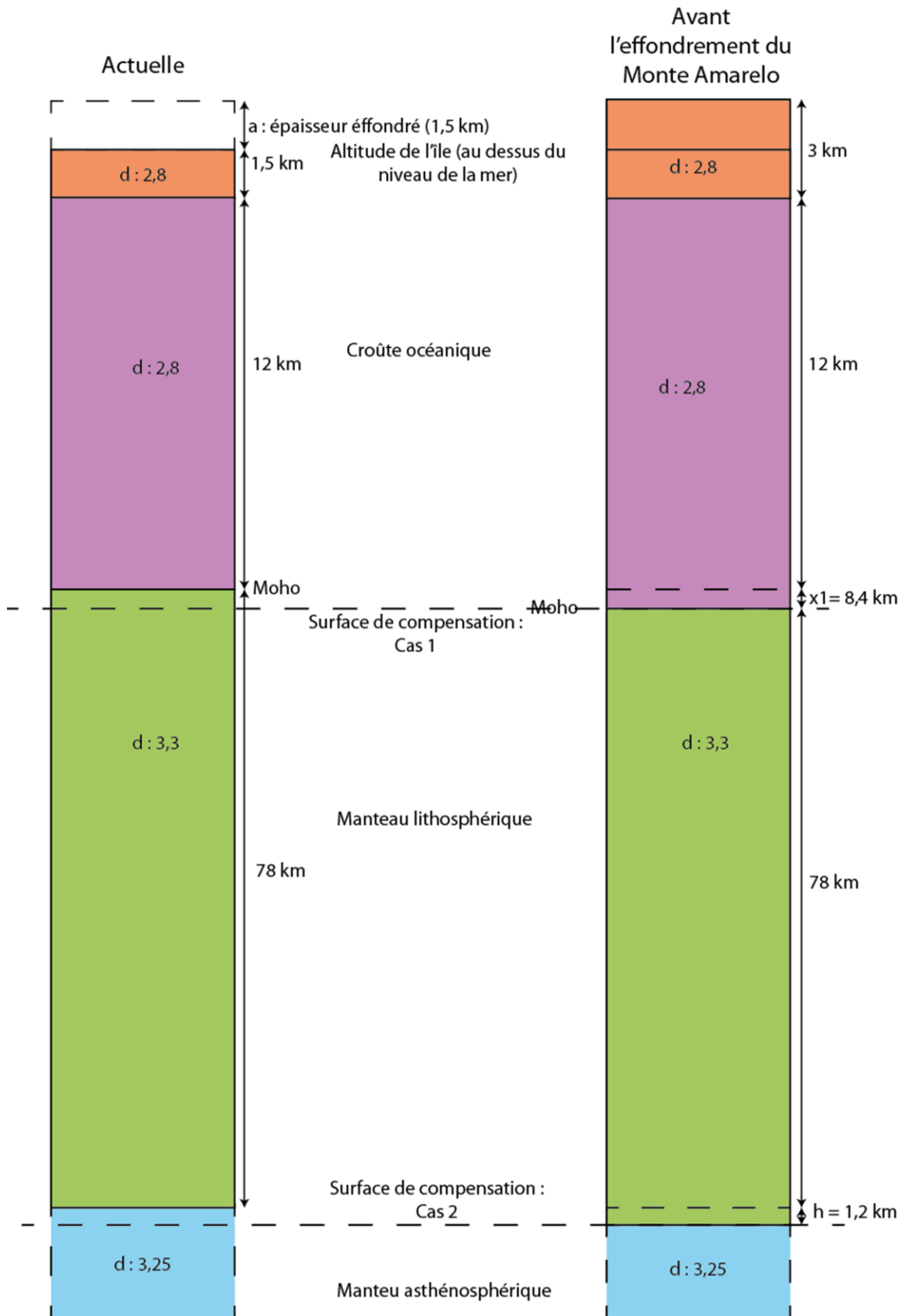
Figure 5.9 : Schéma représentatif du calcul de compensation isostatique liée à l'effondrement de flanc du Monte Amarelo. Deux hypothèse sont testées : la surface de compensation se situe au niveau du Moho (cas 1) ou au niveau de la transition lithosphère/asthénosphère (cas 2). Ce modèle simple montre l'influence de l'effondrement en profondeur.
