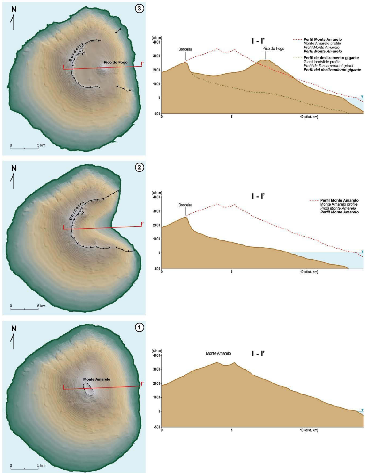
Figure 2.13 : Reconstruction de la déstabilisation massive du flanc Est de l'édifice Monte Amarelo à Fogo (d'après Pérez-Torrado et al. , 2017). 1 : Edifice au maximum de sa croissance, avant le collapse Amarelo ; 2 : glissement massif du flanc oriental il y a 65-123 ka (Foeken et al. , 2009 ; Paris et al. , 2011 ; Ramalho et al. , 2015), volume 130-160 km 3 (Masson et al. , 2008) ; 3 : topographie actuelle montrant le remplissage de la cicatrice de glissement par les produits éruptifs post-effondrement, dont le Pico do Fogo, nouvel édifice central culminant à 2829 m.
