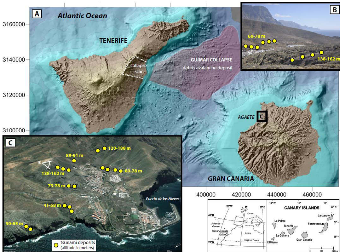
Figure 1.3 : Altitude de dépôts de mégatsunami sur la côte Ouest de Gran Canaria, engendré par une déstabilisation massive du flanc Est de Tenerife (Gúímar effondrement, 830 ka : Paris et al. , 2004 ; Pérez-Torrado et al. , 2006 ; Carracedo et al. , 2011).
