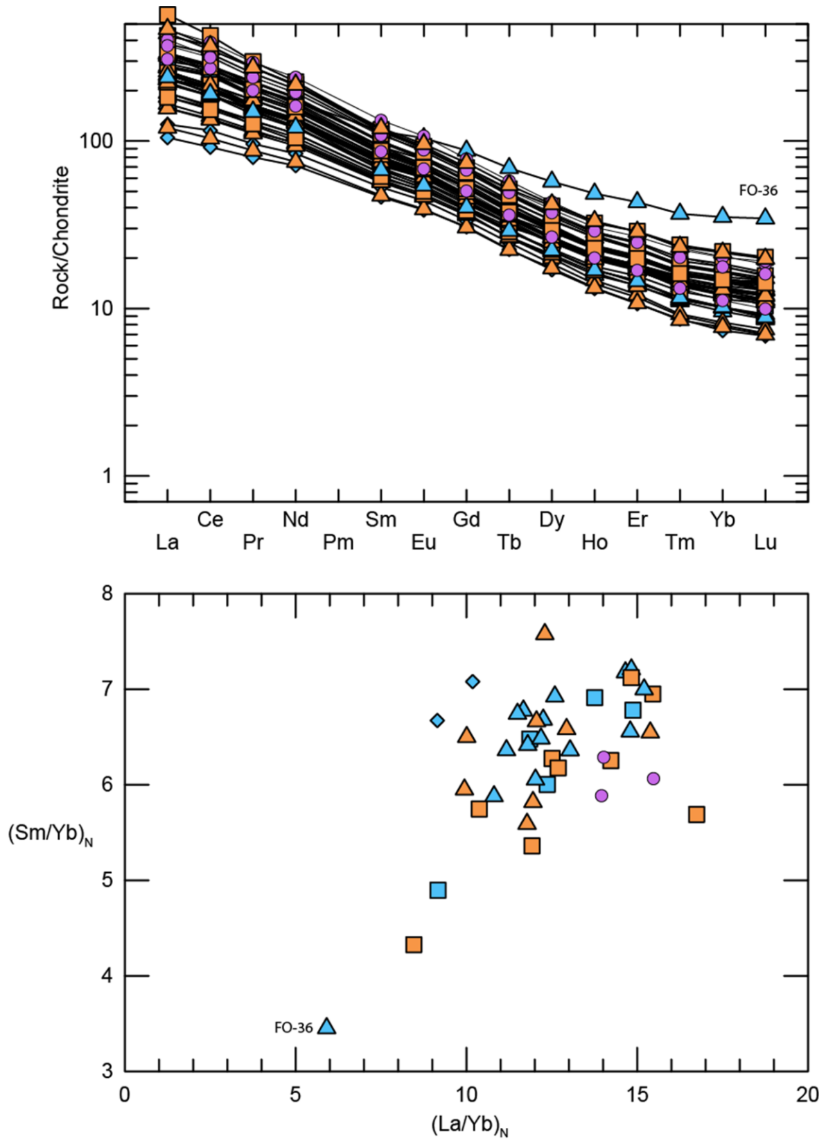
Figure 4.8 : A : Spectre des terres rares des échantillons de Fogo. Les concentrations sont normalisées aux chondrites (Sun et McDonough, 1989). B : Rapport Sm/Yb et La/Yb normalisés aux chondrites.
