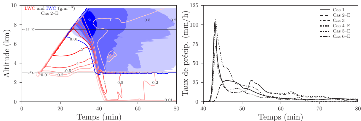
FIGURE R.6 – (a, gauche) Contenu en eau liquide ( \text{g.m}^{-3} , rouge) et contenu en glace ( \text{g.m}^{-3} , bleu) simulé par DESCAM en fonction de l’altitude et du temps pour le cas où tous les INP et mécanismes de glaciation sont actifs (cas 2-E). (b, droite) Évolution temporelle du taux de précipitation ( \text{mm.h}^{-1} ) pour le cas référence (cas 1, noir continu), et pour les cas où tous les INP et où tous les mécanismes sont considérés comme actifs (cas 2-E, violet discontinu), où la nucléation homogène est considérée seule (cas 3, noir pointillé-discontinu court), où la glaciation par immersion est considérée seule (cas 4-E, violet discontinu court), où la glaciation par contact est considérée seule (cas 5-E, violet pointillé-discontinu) et où la nucléation par dépôt est considérée seule (cas 6-E, violet double pointillé-discontinu).
