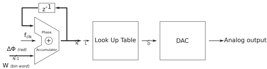
FIGURE 1.14 – Principe de fonctionnement d'une DDS
