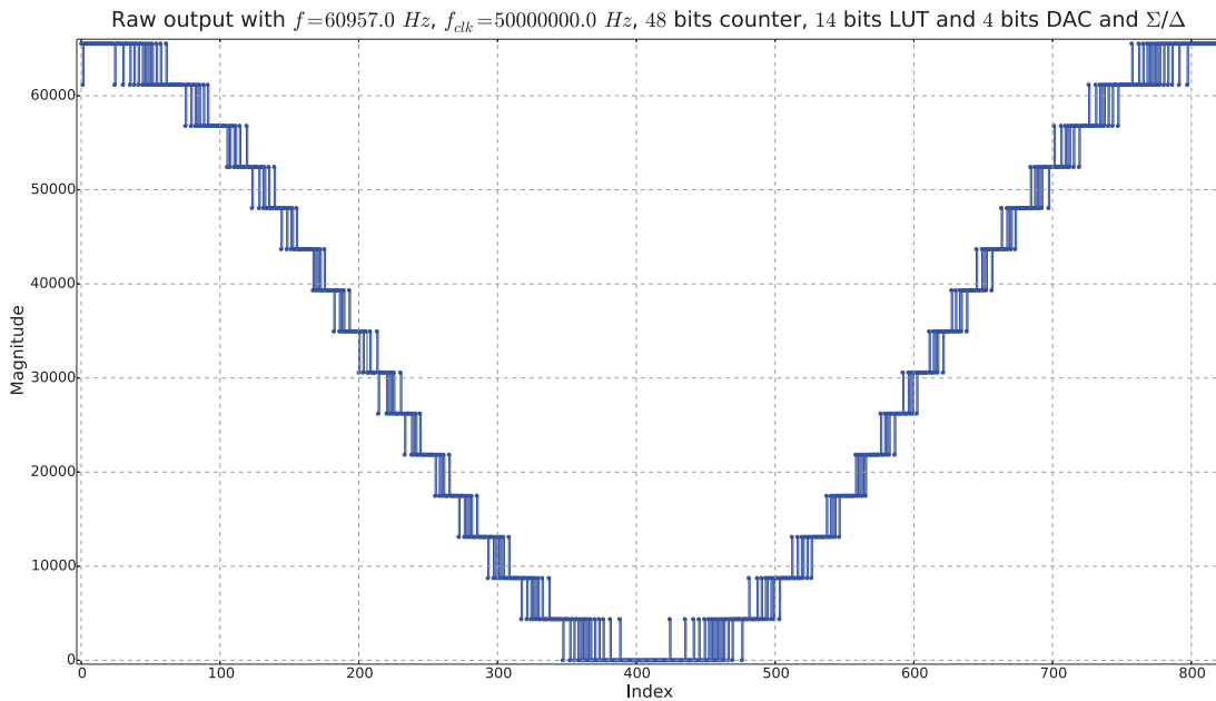
FIGURE 2.31 – Sortie d’une DDS avec un DAC de 4 bits et un convertisseur \Sigma/\Delta
