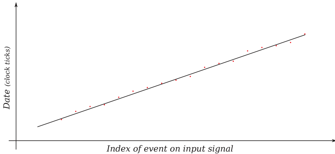
FIGURE 2.7 – Comptage de fréquence par marquage temporel. On relève les dates, exprimées en nombre de périodes d'horloge, des fronts montants du signal d'entrée. La fréquence du signal est donnée par la pente de la droite de régression.
