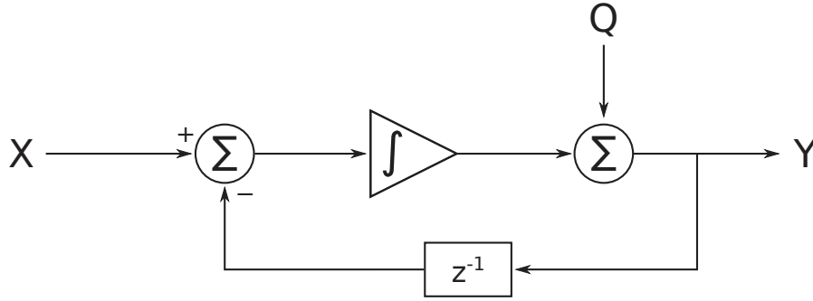
FIGURE 2.29 – Schéma bloc d'un modulateur \Sigma/\Delta
