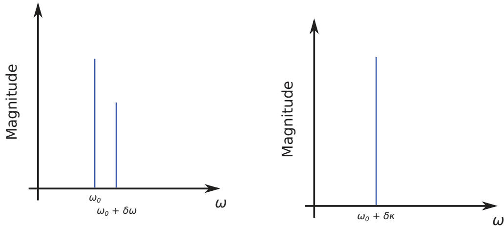
(a) Pulsation réelle (fondamental à \omega_0 et spur à \omega_0 + \delta\omega )
