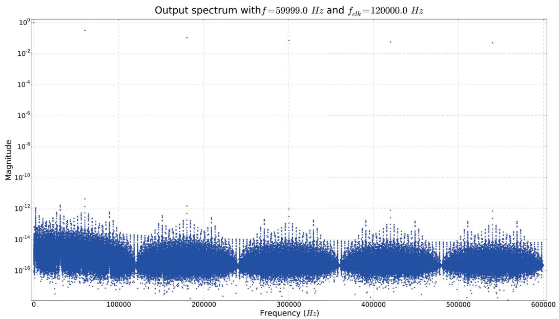
FIGURE 2.11 – Sortie d'une DDS dans un cas non idéal avec un taux de sur-échantillonnage faible (2 ici)
