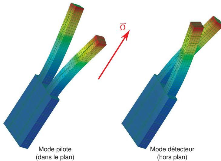
FIGURE 1.11 – Mode de vibration pilote et détecteur du diapason du VIG
