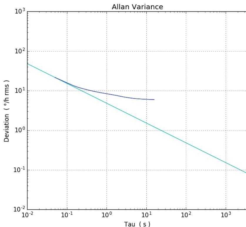
FIGURE 4.7 – Variance d'ALLAN de la sortie du gyromètre. Variance calculée à partir des mesures (bleu). Asymptote pour les temps d'intégration courts (clair).
