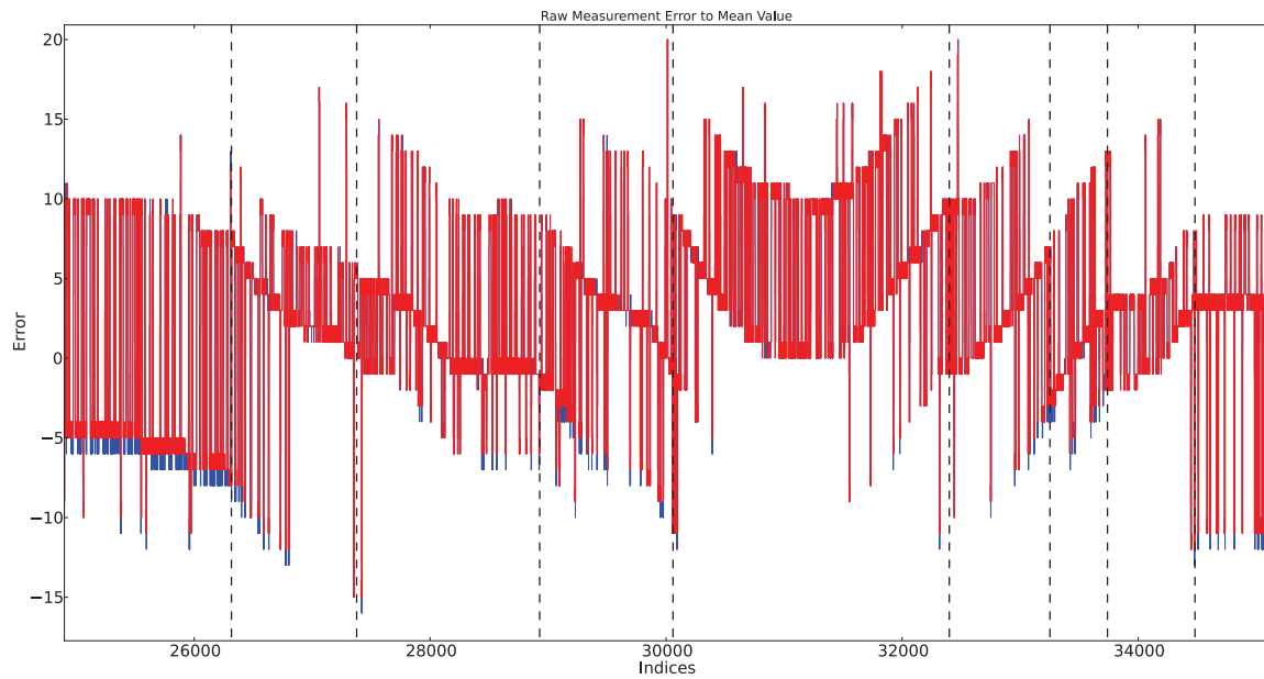
(a) Erreur des différences de date à la moyenne sur 10 000 points environ ( P = 1000 )
