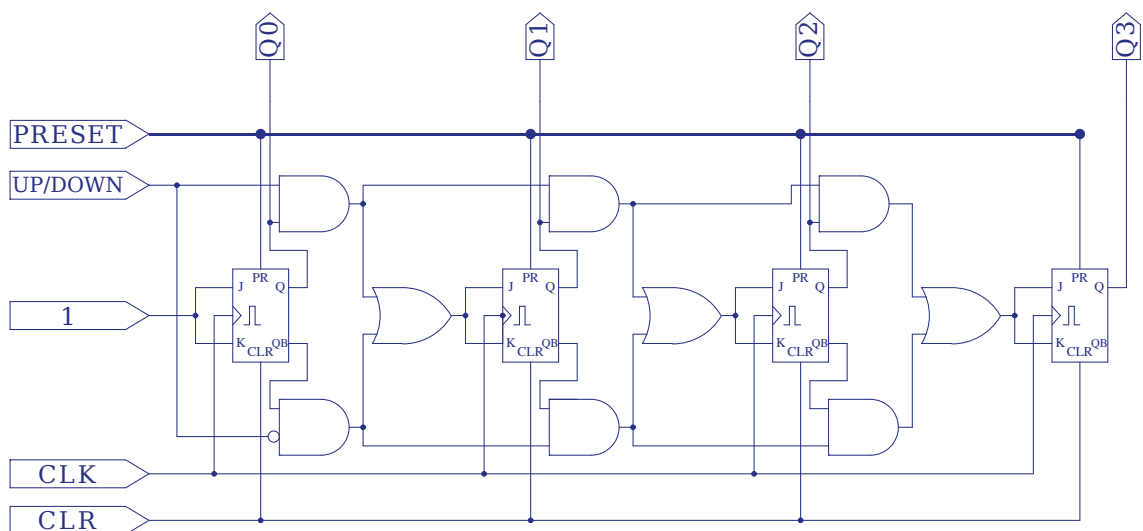
FIGURE B.2 – Architecture d'un compteur synchrone à bascules JK
