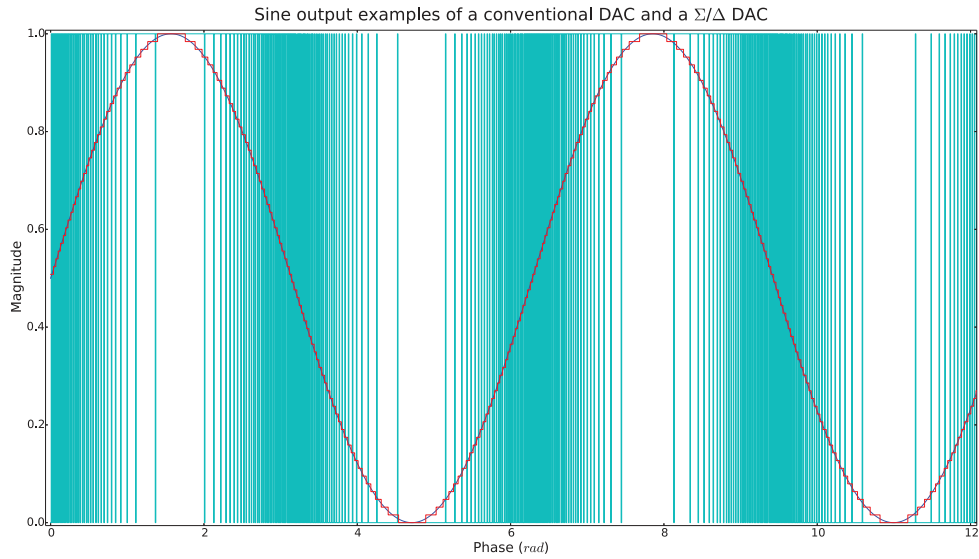
FIGURE 2.27 – Comparaison des sorties d'un DAC conventionnel et d'un convertisseur \Sigma/\Delta par rapport à une sinusoïde de référence
