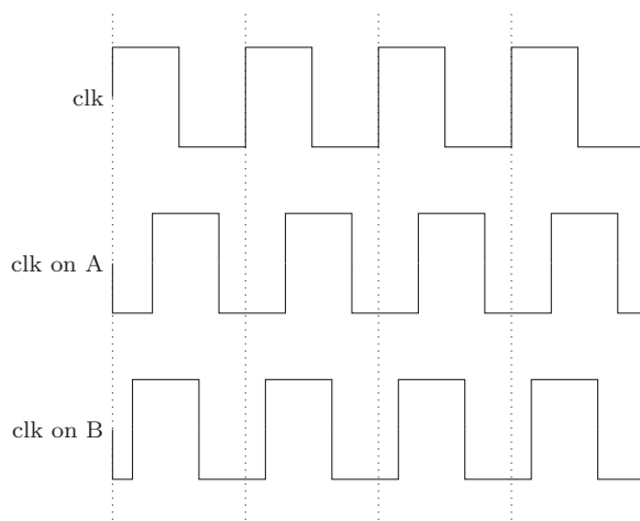
FIGURE 3.13 – Illustration du biais d'horloge, «clock skew» en Anglais : les temps d'arrivée sur les composants A et B diffèrent
