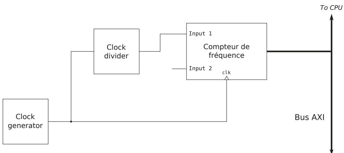
FIGURE 3.12 – Schéma de principe de l'expérience de discrimination de la source des imperfections
