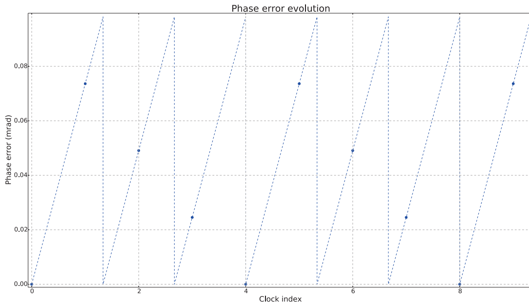
FIGURE 2.17 – Allure du signal d'erreur de phase causé par la troncature
