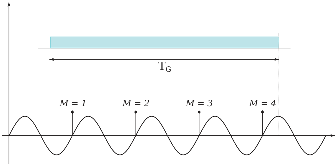
FIGURE 2.1 – Comptage simple d'un signal sinusoïdal
