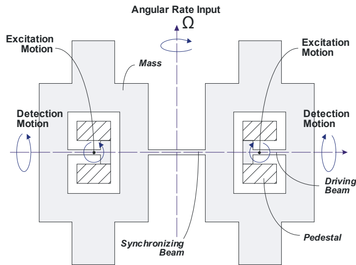
FIGURE 1.8 – Structure et principe du gyromètre de Sensoror
