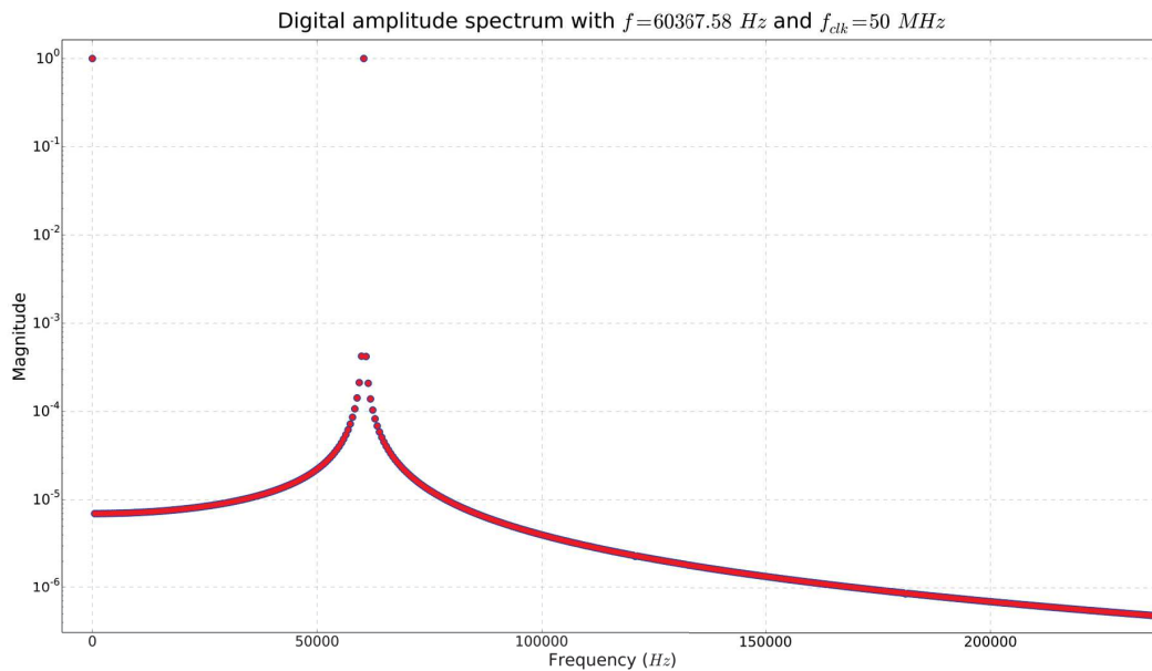
FIGURE 2.15 – Zoom sur les spectres de la figure 2.14
