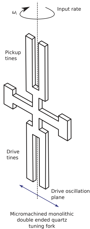
FIGURE 1.9 – Structure du QRS de Systron Doner
