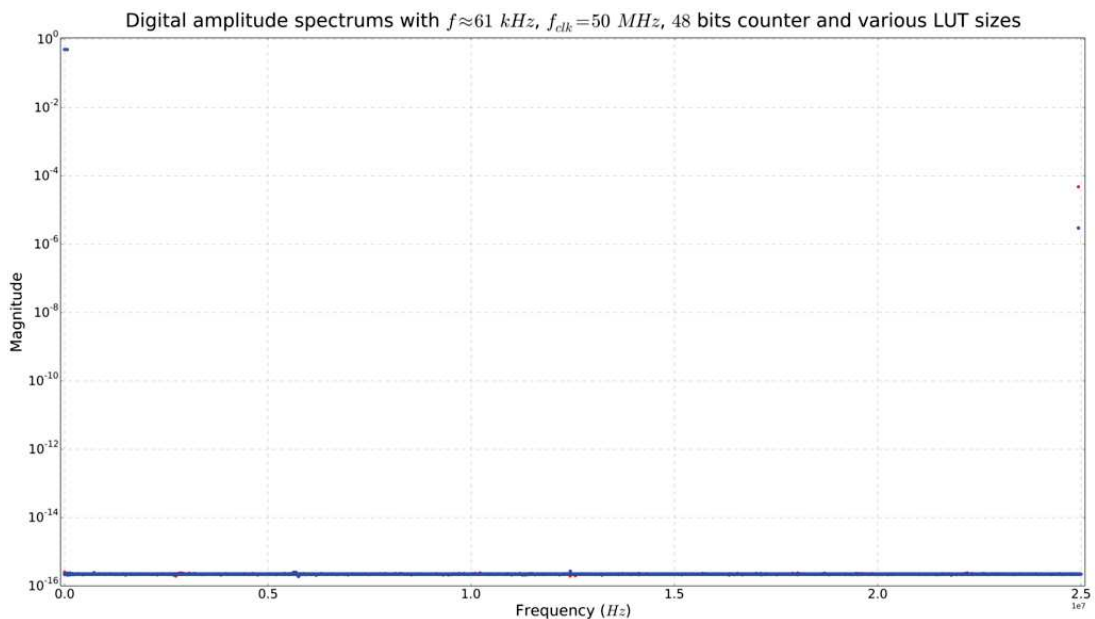
FIGURE 2.21 – Spectres de sortie dans un pire cas (LUT de 14 et 18 bits en rouge et bleu respectivement)
