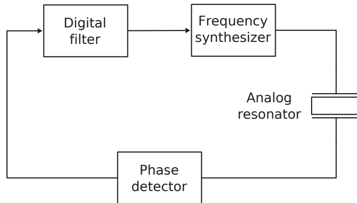
FIGURE 1.13 – Schéma blocs d'un oscillateur numérique avec un résonateur analogique
