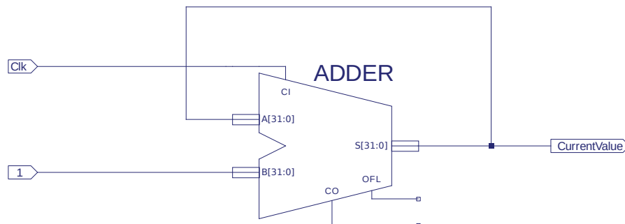
FIGURE 3.3 – Câblage d'un additionneur en compteur
