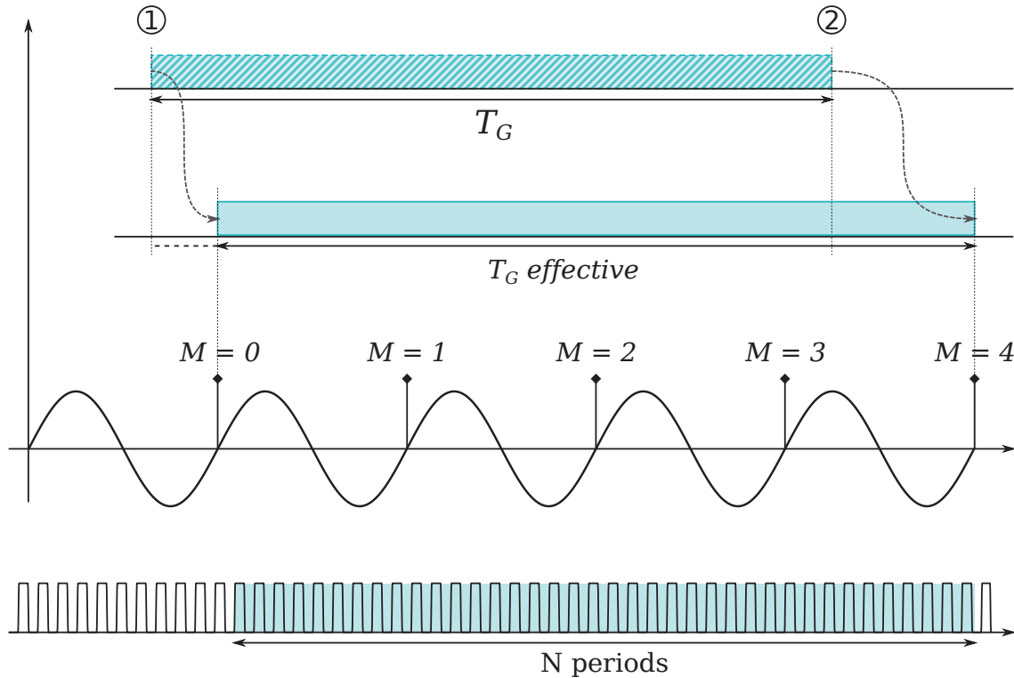
FIGURE 2.2 – Comptage réciproque d'un signal sinusoïdal
