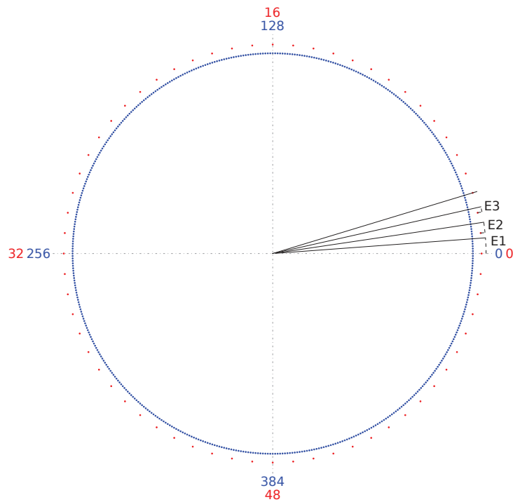
FIGURE 2.16 – Représentation de l'erreur de phase sur le cercle de phase
