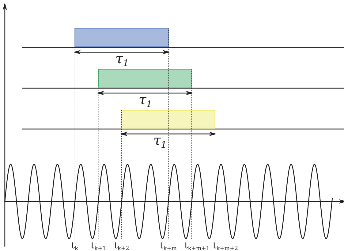
FIGURE 2.4 – Glissement du gate de comptage réciproque en marquage temporel
