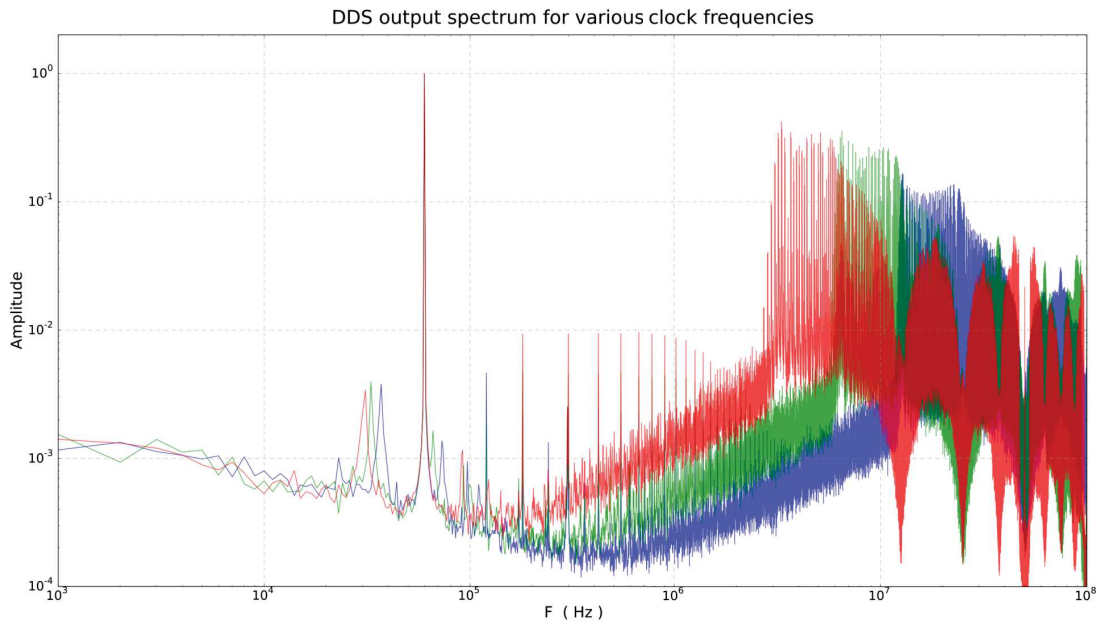
FIGURE 3.21 – Spectre de sortie mesuré de la DDS, avant filtrage, pour trois fréquences d'horloge : 25 MHz (rouge), 50 MHz (vert) et 100 MHz (bleu)
