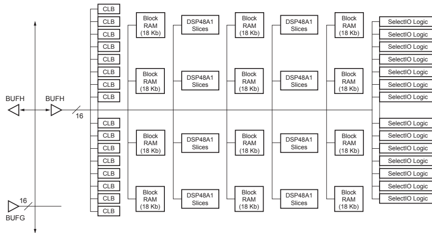
FIGURE 3.16 – Architecture simplifiée d'une rangée du FPGA. Image tirée de [Xila]
