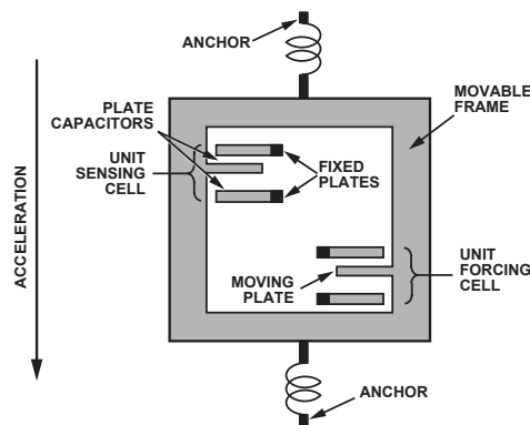
FIGURE 1.2 – Technologie iMEMS pour les accéléromètres [Dev]
