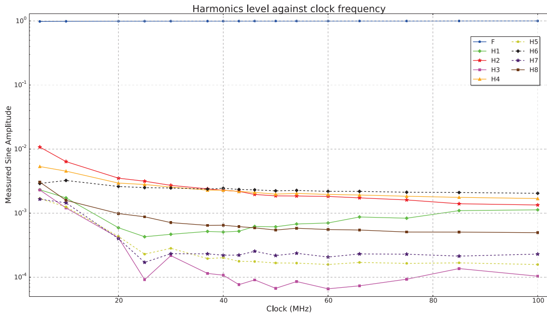
FIGURE 3.22 – Amplitudes relatives des harmoniques en fonction de la fréquence d’horloge de la DDS
