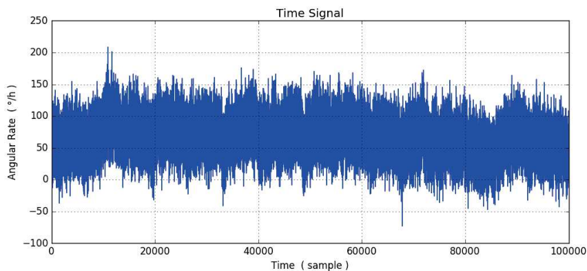
FIGURE 4.6 – Signal temporel de sortie du gyromètre au repos
