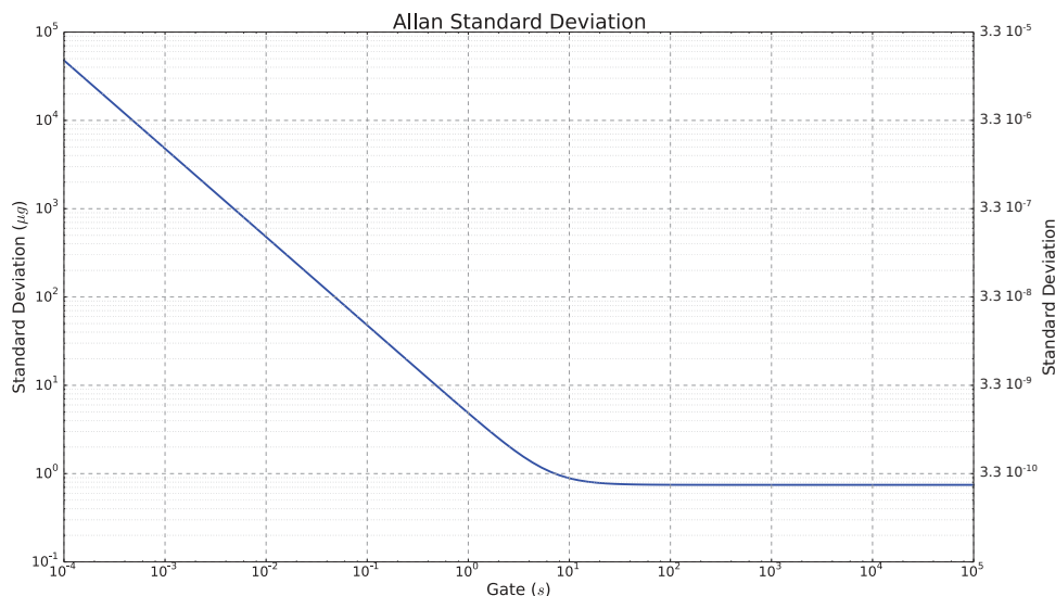
FIGURE 1.5 – Variance d'ALLAN de l'accéléromètre VIA (normalisée par rapport à la fréquence de résonance au repos)
