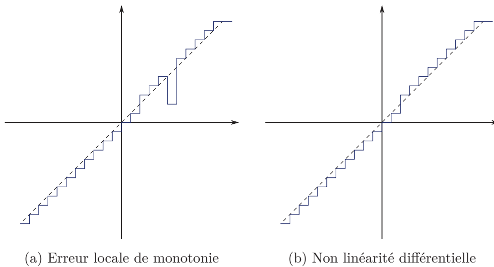
FIGURE 2.26 – Erreurs de linéarité d'un DAC
