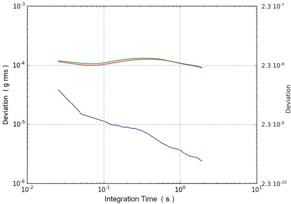
FIGURE 4.3 – Variance d’ALLAN pour la cellule accélérométrique. (rouge, vert) variance pour les cellules séparées. (bleu) variance du signal différentiel.
