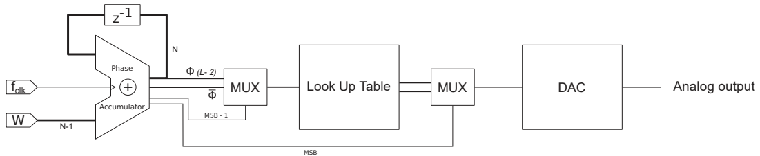
FIGURE 3.18 – DDS avec table demie-onde et utilisation du MSB de l’accumulateur de phase pour former le MSB du DAC
