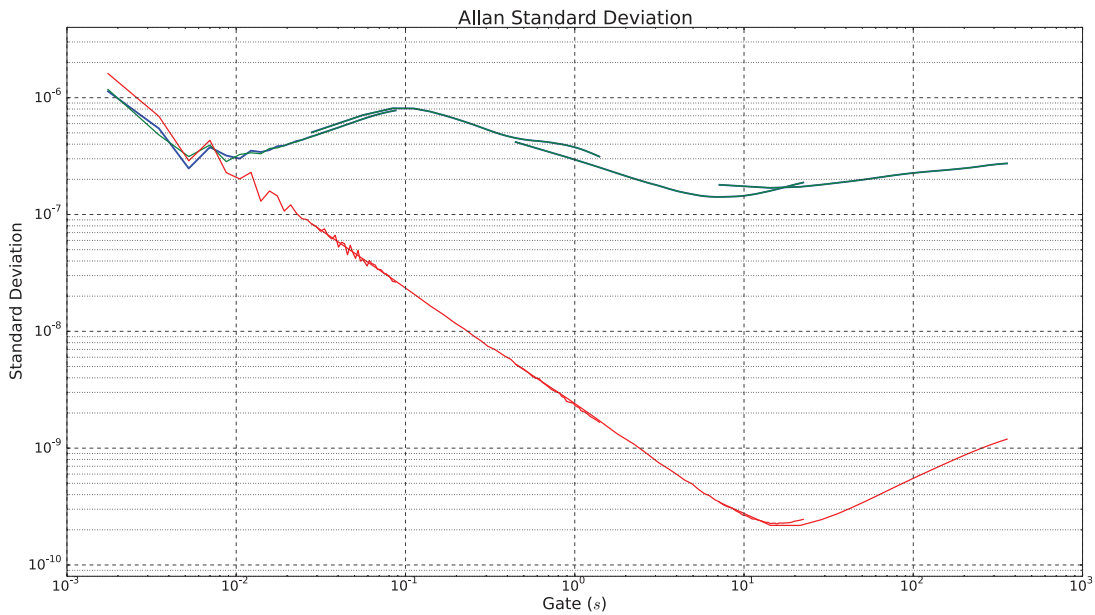
FIGURE 3.8 – Variance d’ALLAN d’une mesure différentielle en rouge, à partir des mesures simples en bleu et vert.
