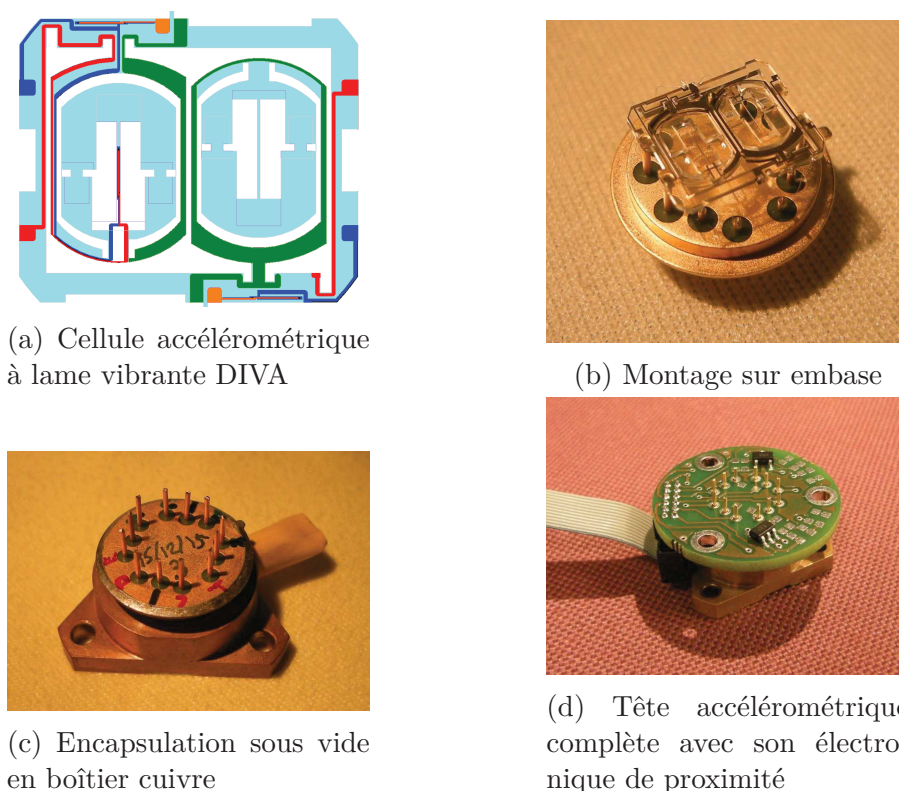
FIGURE 4.1 – Prototype d'un accéléromètre VIA
