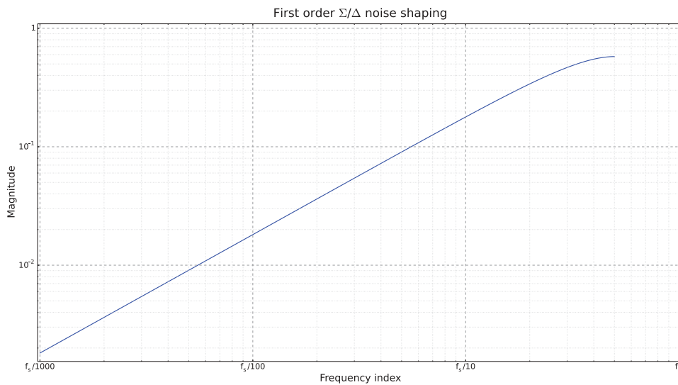
FIGURE 2.30 – Densité spectrale de bruit d'un DAC \Sigma/\Delta du premier ordre (normalisée par rapport à la fréquence d'échantillonnage et au pas de quantification).
