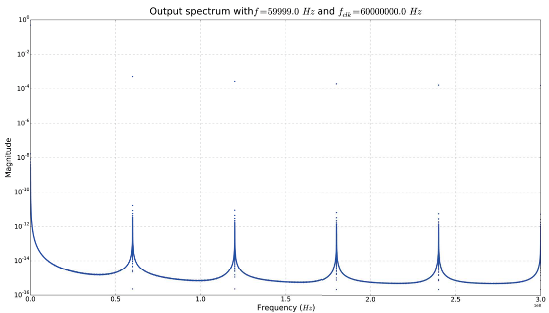
FIGURE 2.12 – Sortie d'une DDS dans un cas non idéal avec un taux de sur-échantillonnage élevé
