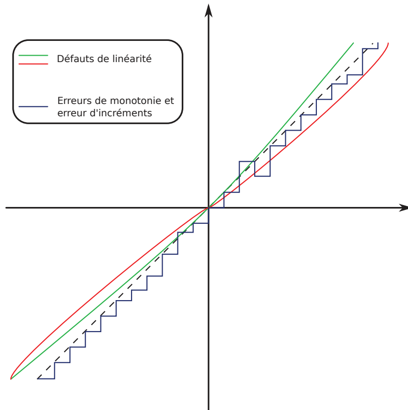
FIGURE 2.25 – Représentation des erreurs de non-linéarité d'un DAC
