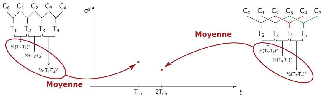
FIGURE C.2 – Représentation graphique du calcul de la variance d'ALLAN
