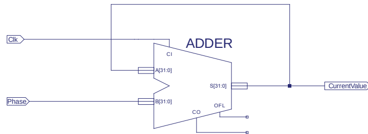
FIGURE 3.15 – Câblage d'un additionneur en accumulateur
