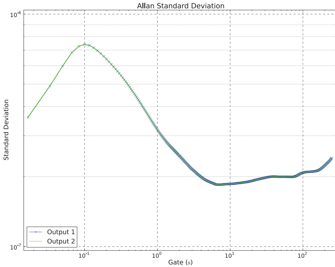
FIGURE 3.7 – Variance d’ALLAN d’un Agilent 33522A obtenue avec le FPGA pour une fréquence de comptage de 300 MHz
