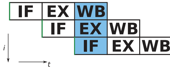
FIGURE E.2 – Exécution d’instructions dans un processeur avec un pipeline à 3 niveaux
