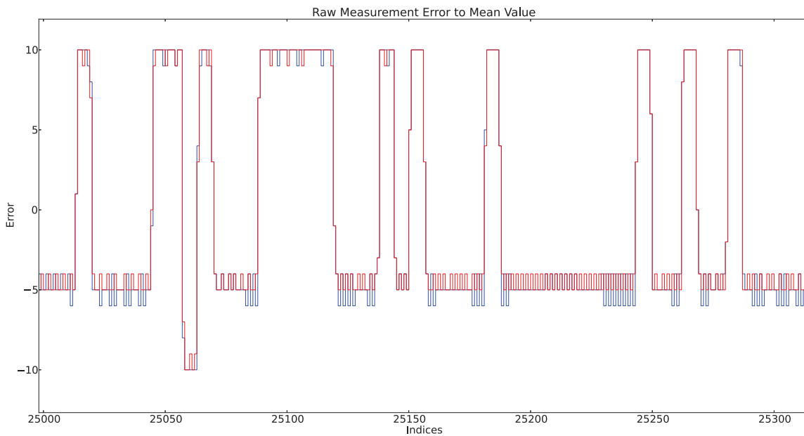
FIGURE 3.11 – Erreur des différences de date à la moyenne sur 300 points environ ( P = 1000 )
