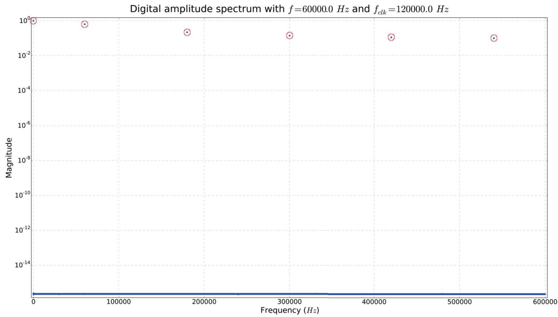
FIGURE 2.10 – Spectre de sortie d'un signal à 60 kHz avec une fréquence d'échantillonnage de 120 kHz
