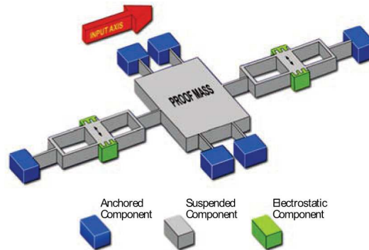
FIGURE 1.3 – Schéma de principe de l'accéléromètre SOA du Draper Laboratory (d'après [HMS + 06])
