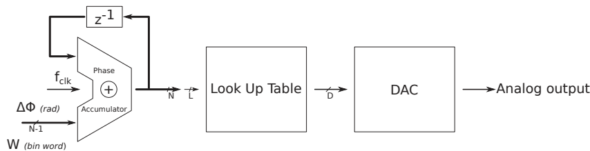
FIGURE 2.8 – Schéma de principe d'une DDS
