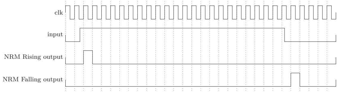
FIGURE 3.4 – Fonctionnement d'un monostable non réenclenchable
