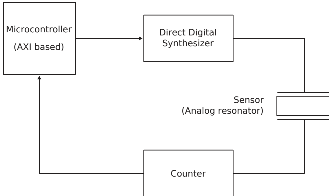
FIGURE 1.15 – Architecture numérique retenue pour les capteurs vibrants de l'Onera (les amplificateurs de charges ne sont pas représentés, ils se situent juste avant et juste après le capteur)
