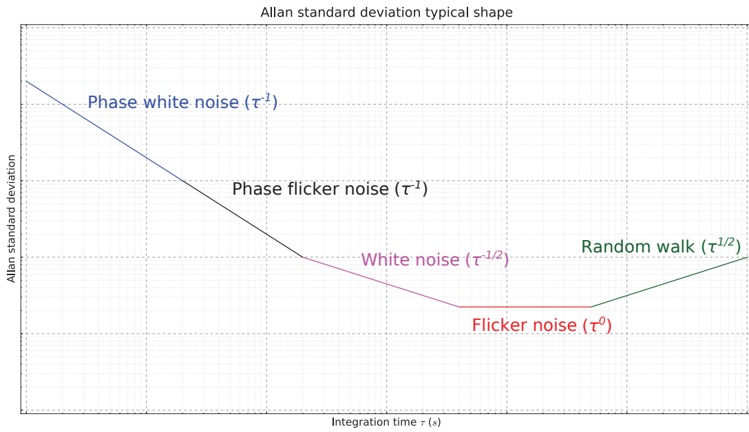
FIGURE C.1 – Forme caractéristique de l'écart type ( \sigma_y(\tau) ) d'ALLAN
