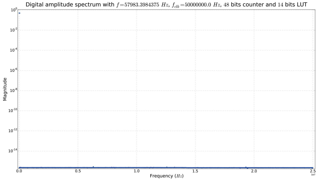
FIGURE 2.19 – Spectre de sortie en l’absence de troncature de phase : fondamental parfait (en haut, à gauche, amplitude \frac{1}{2} ), bruit spectral confondu avec le bruit de calcul, et raies parasites à la fréquence de NYQUIST-SHANNON.
