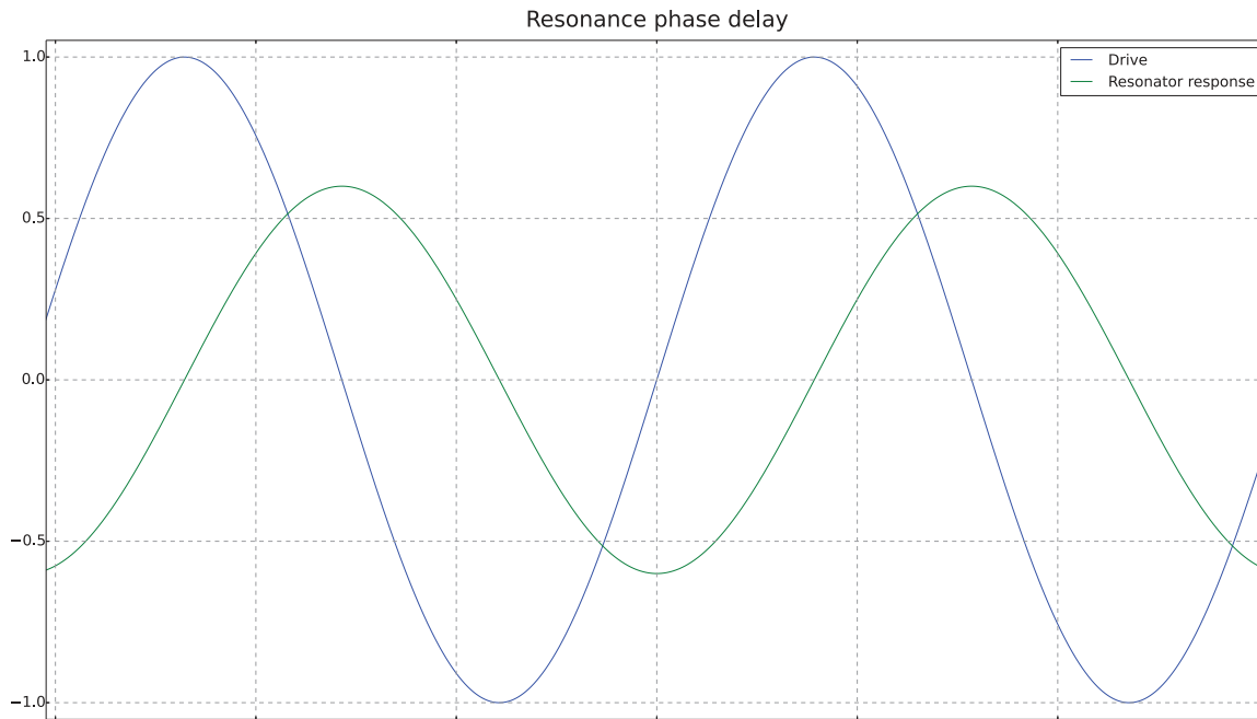
FIGURE 3.14 – Représentation du déphasage entre le signal d'excitation et la réponse du capteur
