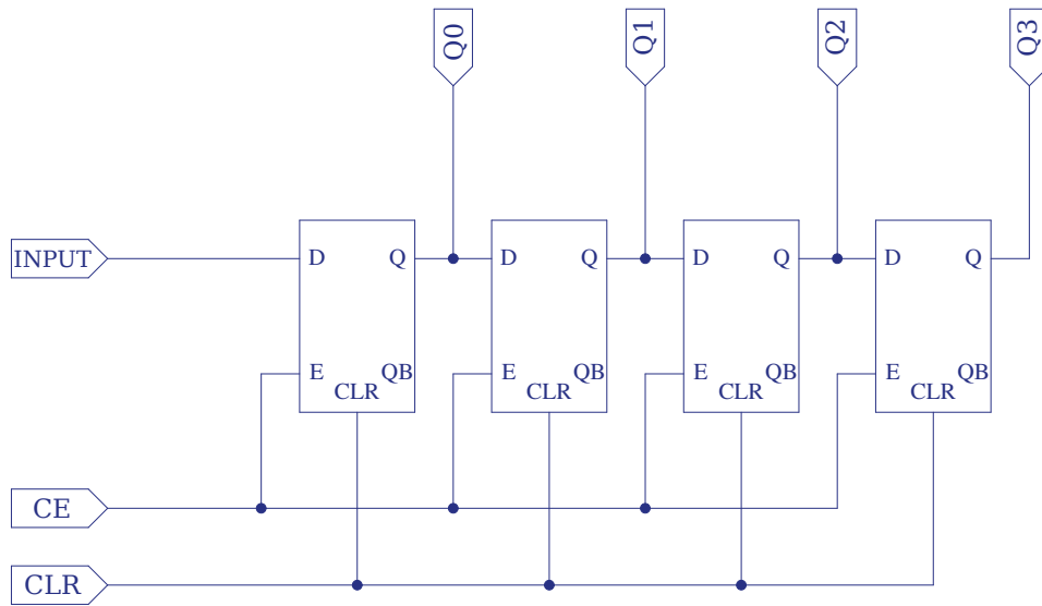
FIGURE 2.3 – Exemple d’une chaîne à retard à bascules D. Plutôt que d’avoir une sortie toutes les portes, il est possible d’en avoir toutes les n portes.
