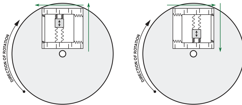
(b) Illustration du fonctionnement d'un gyromètre iMEMS®
