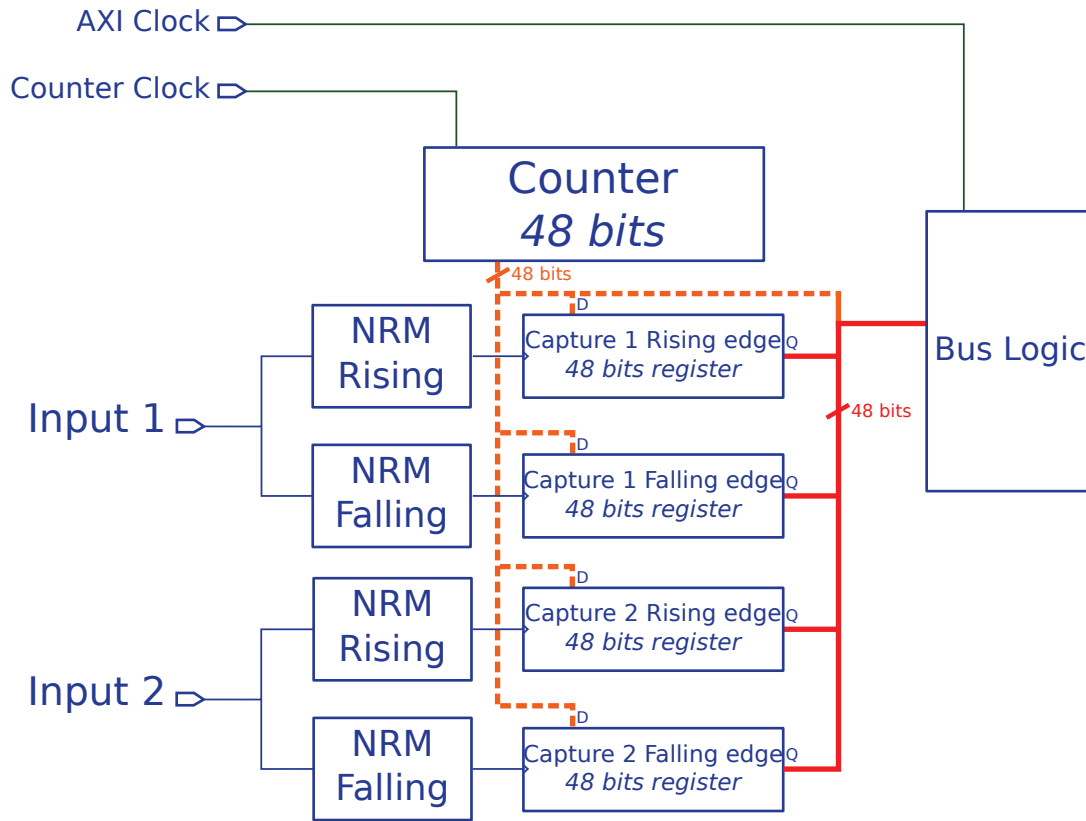
FIGURE 3.5 – Architecture du périphérique de comptage de fréquence développé
