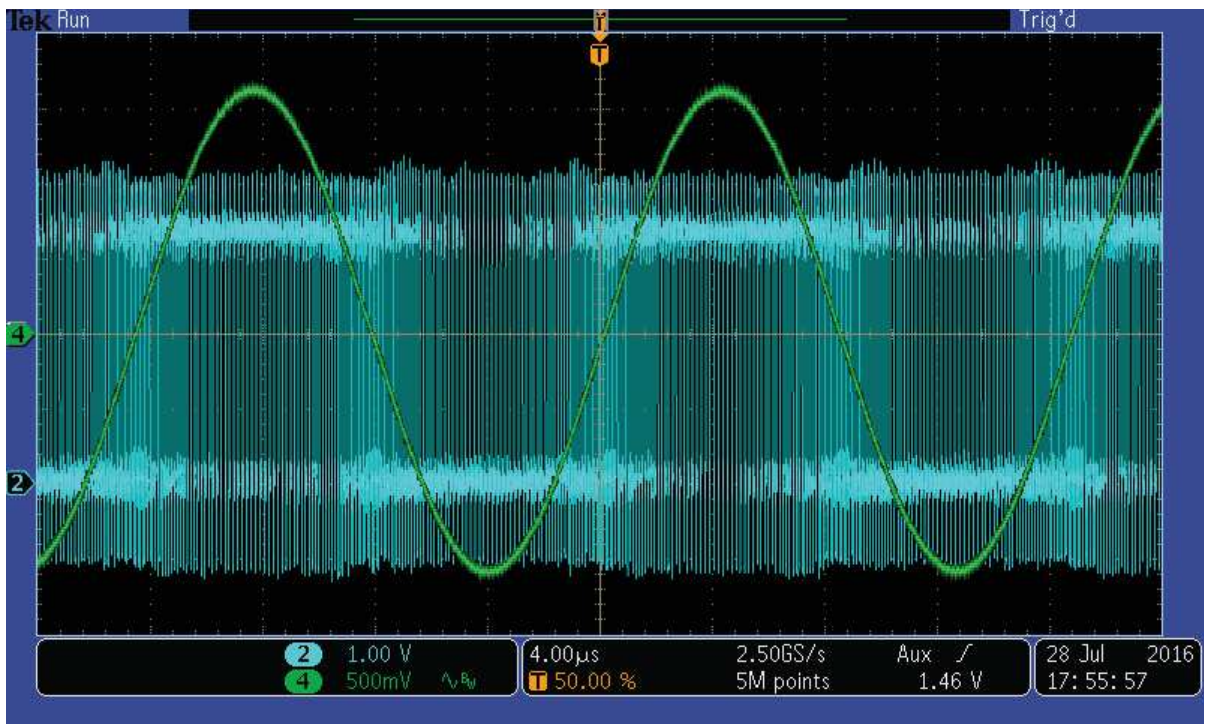
(a) Mesures en sortie de DDS et après le filtre.
