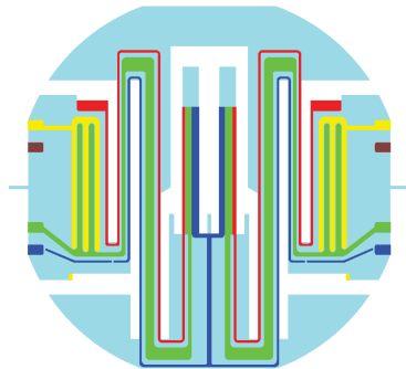
(a) Cellule gyrométrique vibrante VIG
