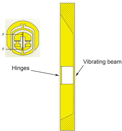
FIGURE 1.4 – Une cellule VIA
