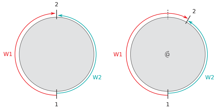
FIGURE 1.6 – Illustration de l'effet SAGNAC : deux signaux lumineux qui partent dans des directions opposées présentent une différence de marche lorsqu'ils se rejoignent si le mobile en leur centre entre en rotation
