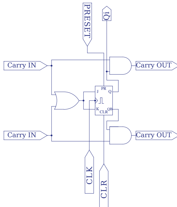
FIGURE B.3 – Étage d'un compteur universel à bascule JK
