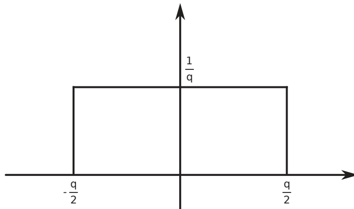
FIGURE 2.24 – Probabilité d'erreur de quantification d'un DAC
