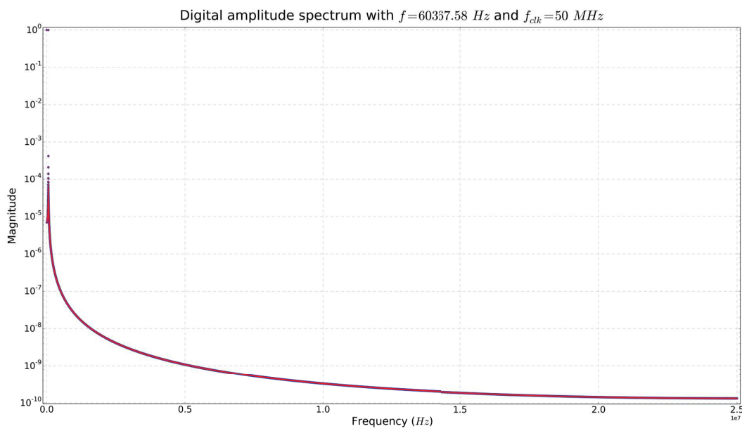
FIGURE 2.14 – Spectres de sorties de deux DDS qui ne diffèrent que par leur nombre de bits sur l'accumulateur de phase
