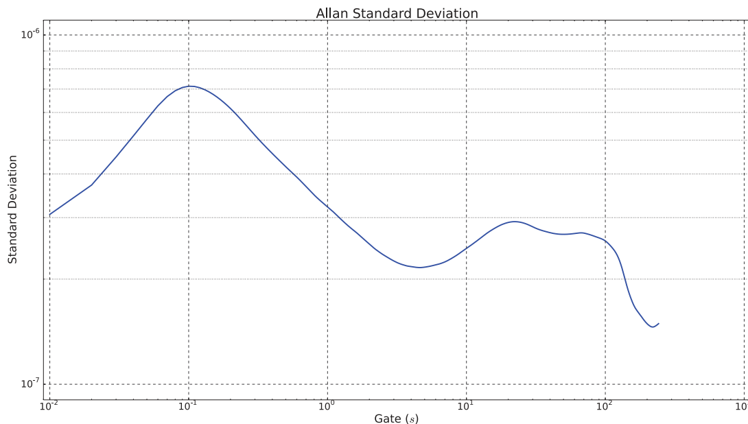
FIGURE 3.6 – Variance d'ALLAN obtenue lors de la mesure d'un signal à 1 kHz (normalisée par rapport à F_0 )
