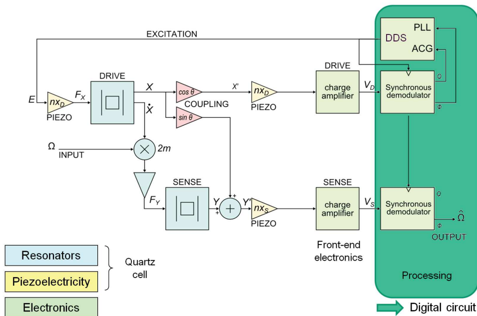
FIGURE 4.5 – Architecture électronique du gyromètre vibrant. Les propriétés piézoélectriques du quartz sont utilisées aussi bien pour l'excitation (transformation de la tension appliquée en force exercée sur le résonateur pilote), que pour la détection (transformation des déformations du résonateur en charges électriques).
