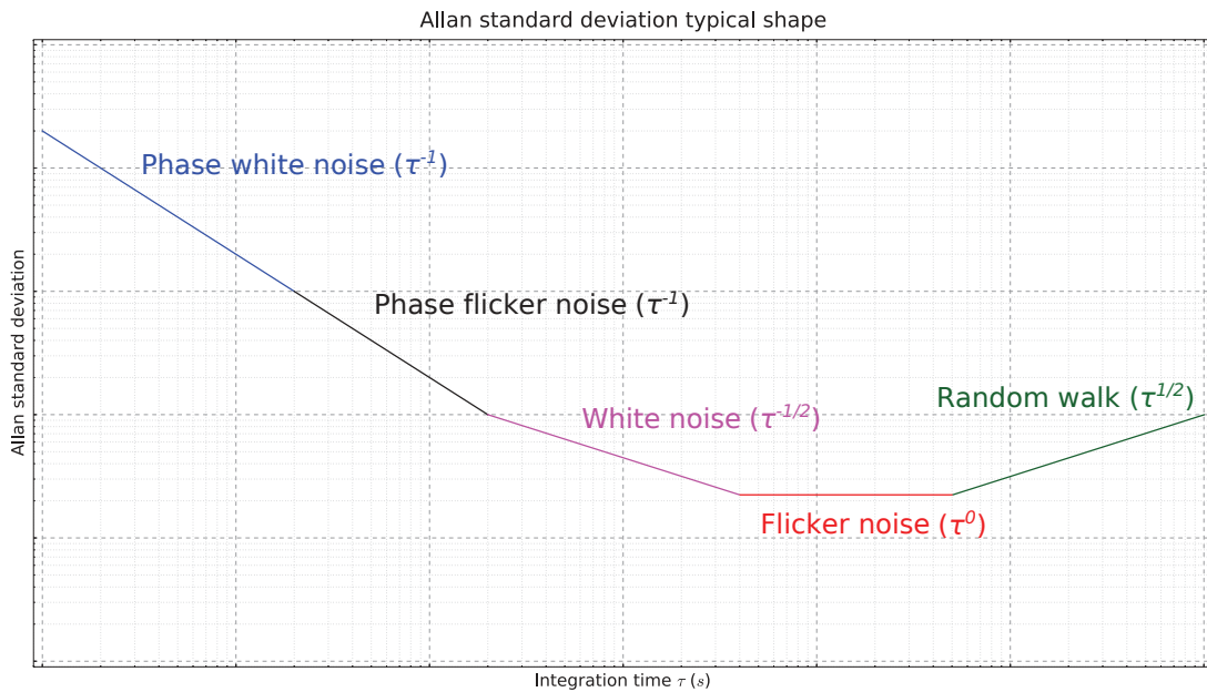
FIGURE 2.6 – Forme caractéristique de la variance d’ALLAN et identification des contributeurs majoritaires
