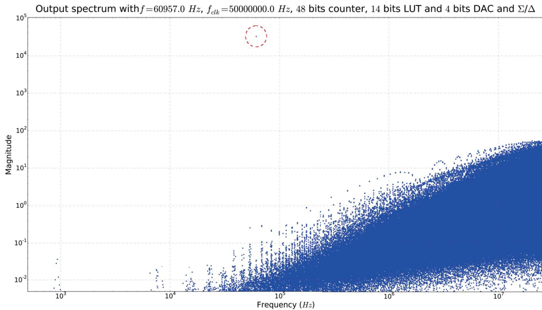
FIGURE 2.33 – Spectre du signal de la figure 2.31 en échelle logarithmique. Le fondamental de la sinusoïde est présent à l’amplitude 3 \times 10^4 , bien au dessus du bruit et des spurs.
