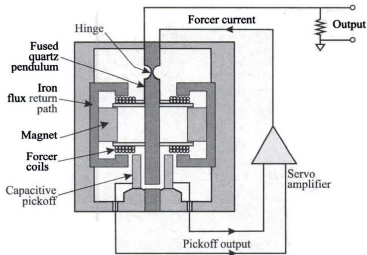
FIGURE 1.1 – Schéma de principe des accéléromètre à technologie Q-Flex® (d'après [Jac72])
