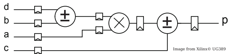
FIGURE 3.2 – Architecture simplifiée d'un bloc DSP48A1
