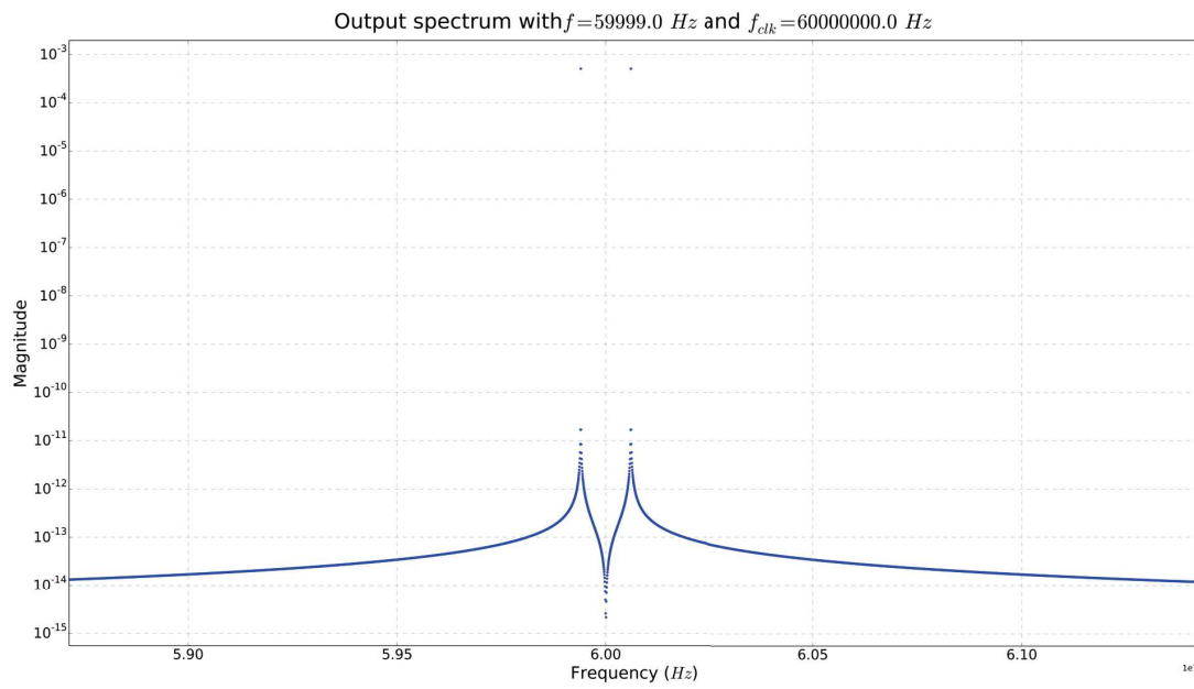
FIGURE 2.13 – Mise en évidence des symétries (zoom de la figure 2.12 autour de f = 60 MHz)
