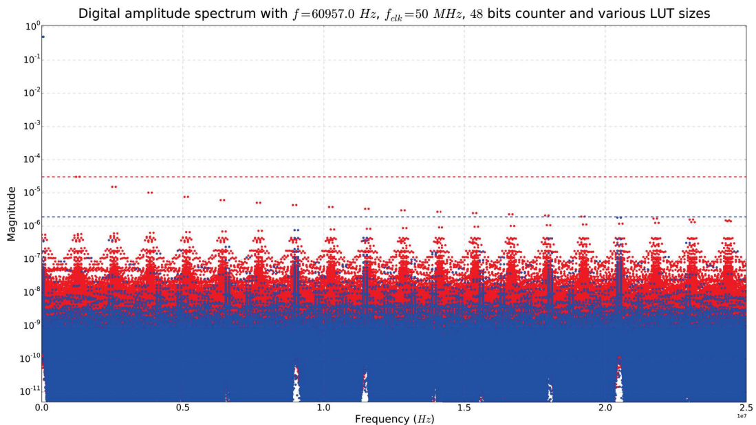
FIGURE 2.22 – Spectres de sortie dans des cas quelconques (LUT de 14 et 18 bits en rouge et bleu respectivement)
