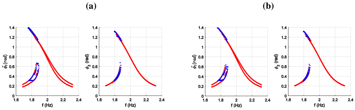
Fig.5.24. Envelopes des amplitudes des réponses \tilde{\phi}_1 et \phi_2 , en coordonnées physiques, des deux pendules calculées par (a) la méthode LHS et (b) la méthode gPC, pour \delta_l = 2\%
