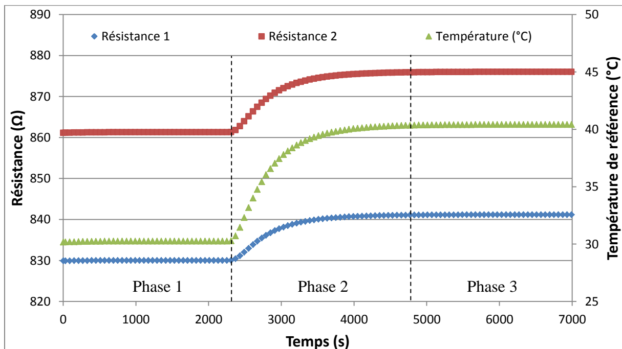
Figure 4.7 : Phases d'étalonnage par comparaison des sondes à résistance pour une température de consigne de 40 °C
