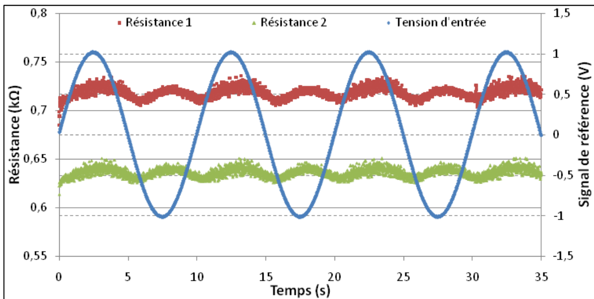
Figure 4.21 : Réponse temporelle des sondes à résistances (Méandre 60 \mu\text{m} , 2 fils - 0,1 mA) en excitation radiative sinusoïdale ( 2 \times 10^{-1} Hz)
