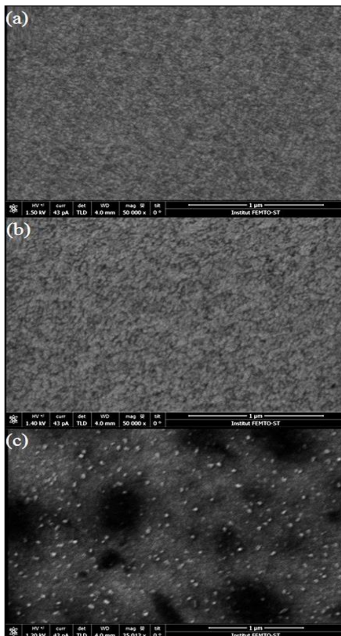
Figure 3.21 : Photos MEBE pour trois films Pt/Cr avant recuit (a), après recuit 250°C (b), et après recuit 450°C (c)
