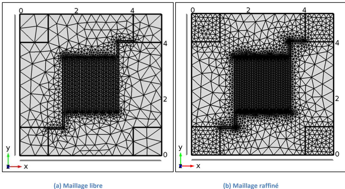
Figure 2.5 : Exemple de maillage du premier modèle (modèle 1)
