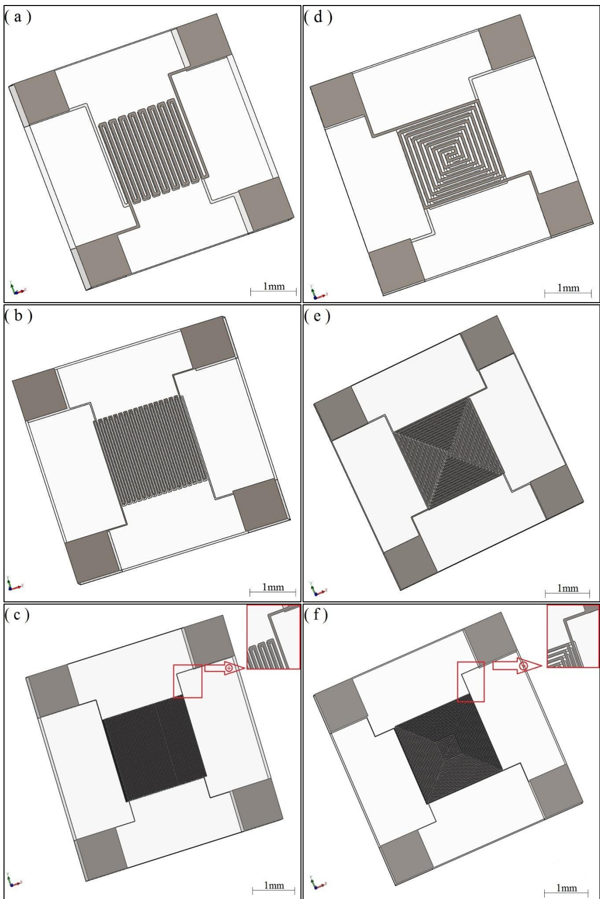
Figure 2.2 : Différentes structures des fluxmètres thermiques
