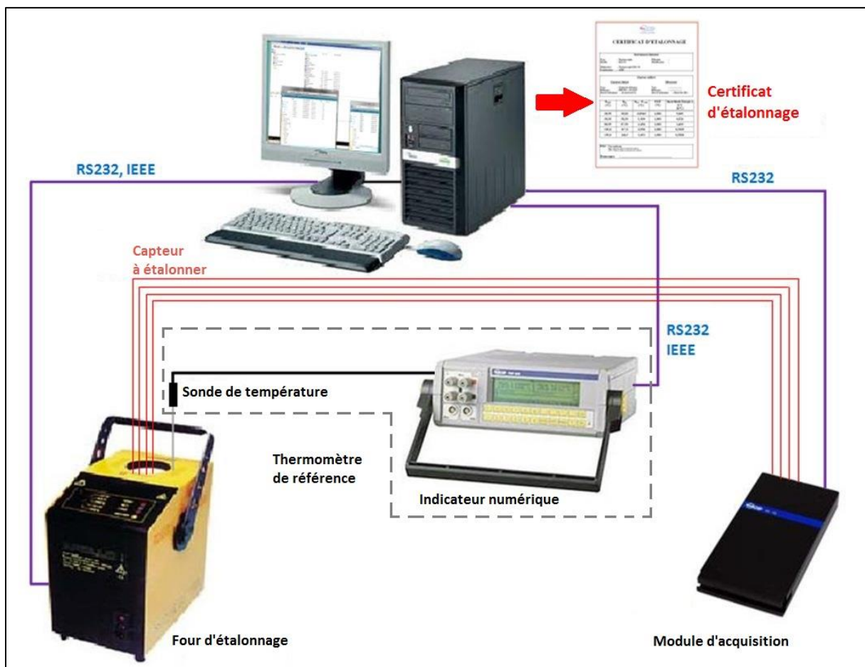
Figure 4.1 : Schéma de principe du banc d'étalonnage (d'après [1]).
