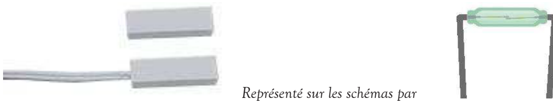
FIGURE 2.46 : Photographie du capteur d'ouverture/fermeture de fenêtre lextronic.fr
