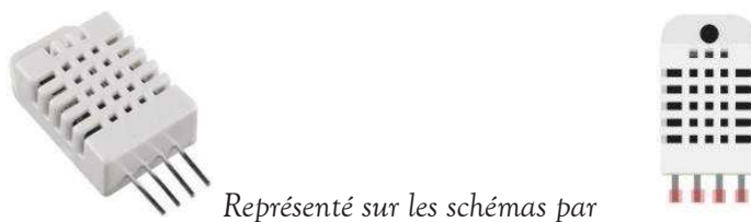
FIGURE 2.45 : Photographie du capteur de température et d'humidité DHT22 roboshop.com
