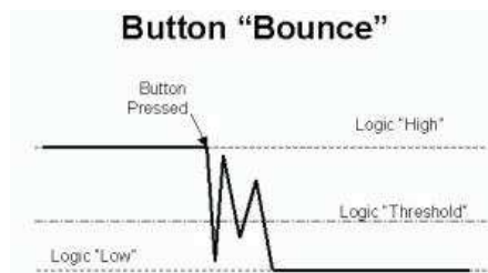
FIGURE 2.47 : Effet rebond lorsqu'un bouton poussoir/interrupteur est actionné (LAMBOT, 2013)
