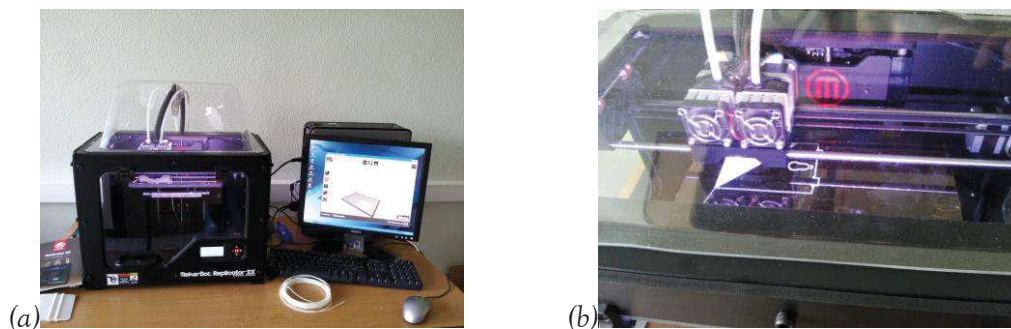
FIGURE 2.59 : Photographie (a) de l'imprimante MakerBot : Replicator 2x et (b) de l'impression d'un couvercle du boîtier de l'auteur
