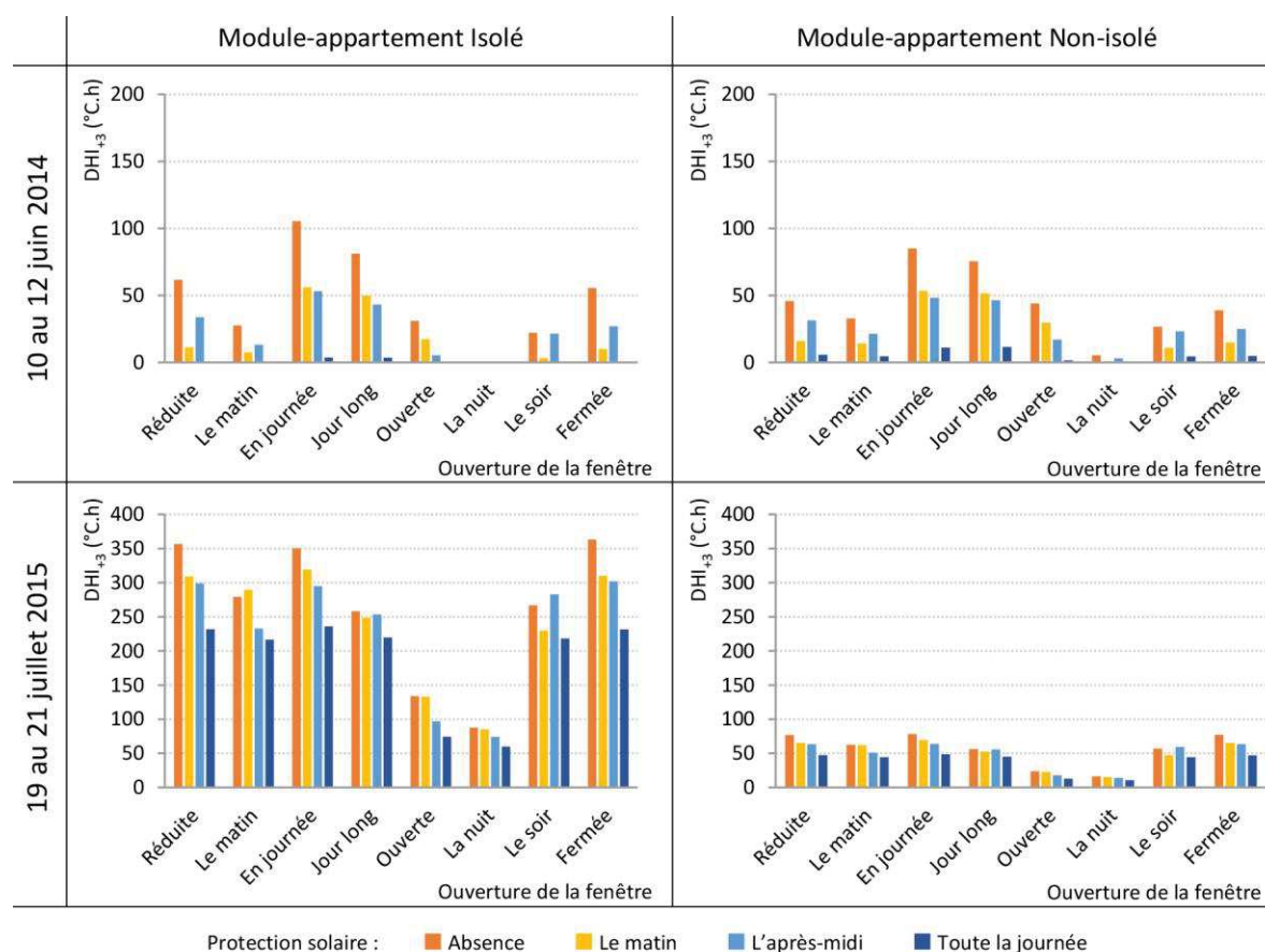
FIGURE 4.14 : DHI +3 des modules-appartements (isolé et non-isolé) orientés Sud en fonction des typologies d'ouverture et de fermeture de la fenêtre et du volet lors des trois jours les plus chauds de 2014 (du 10 au 12 juin) et de 2015 (du 19 au 21 juillet) de l'auteur
