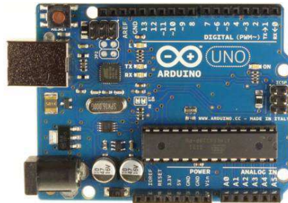
FIGURE C.1 : Photographie de la carte Arduino Uno Arduino.cc
