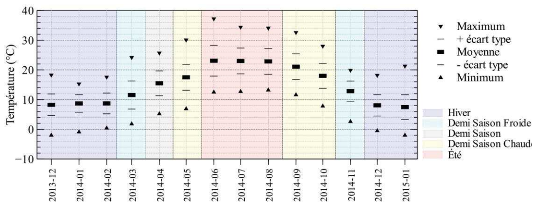
FIGURE 2.11 : Analyse mensuelle des températures et découpage en cinq saisons d'étude de l'auteur grâce au fichier météo de Nîmes-Courbessac de Météo France
