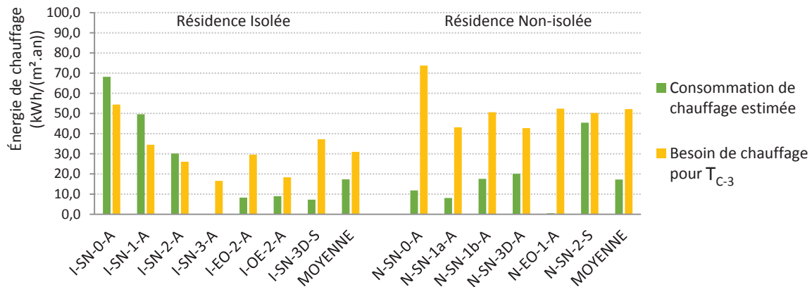
FIGURE 4.7 : Consommation de chauffage estimée et besoin de chauffage simulé avec les scénarios issus des comportements réels, une consigne de température à T_{C-3} et la météo réelle dans les deux résidences sur l'année 2014 de l'auteur
