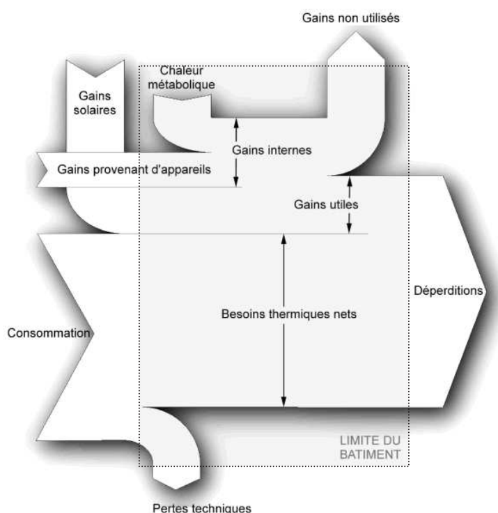
FIGURE 1.7 : Diagramme de Sankey reprenant les différents apports et pertes d'énergie dans le bâtiment
