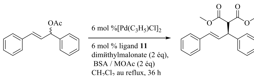
Schéma 5. Réaction Tsuji–Trost utilisant le ligand 11 .
