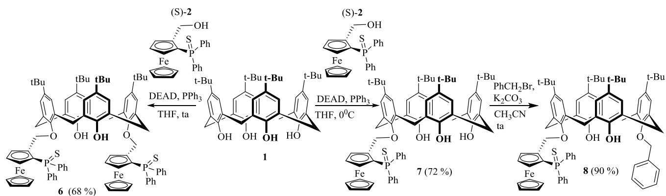
Schéma 2. Synthèse des composés 6-8 .
