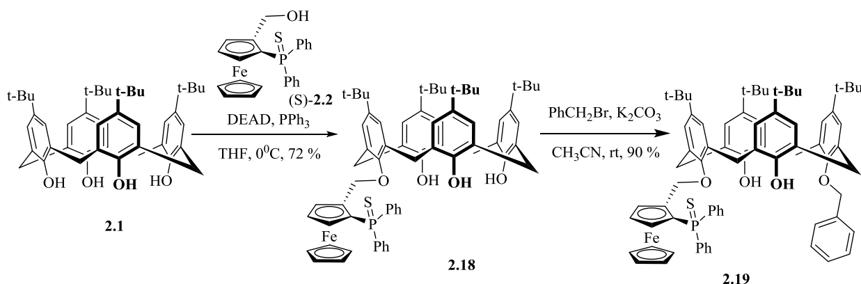
Scheme 2.4.
