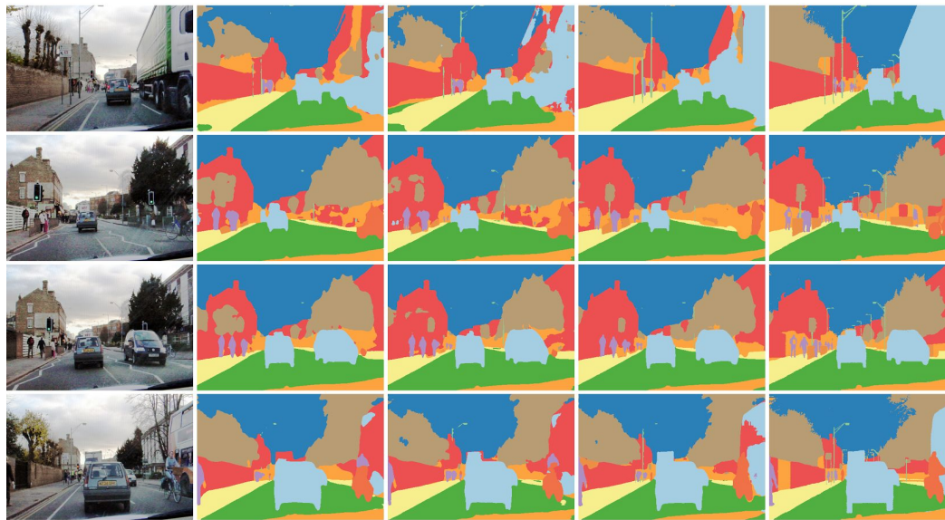
(a) image (b) base-net (c) spatial G-CRF (d) st-G-CRF (e) GT
