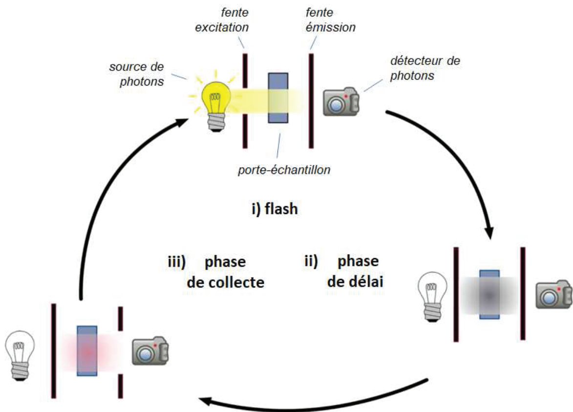
Figure 26 Représentation technique du cycle d'analyse par fluorescence en temps résolu. Source : réalisation laboratoire.
