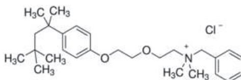
Figure 67 Structure chimique de la molécule Hyamine 1622
