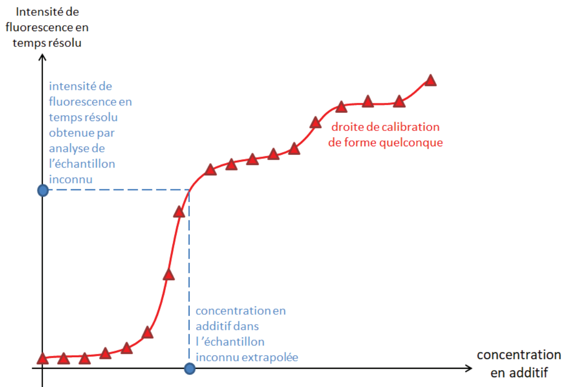
Figure 72 Méthode d'extrapolation graphique de la concentration d'un échantillon à partir de son intensité de fluorescence en temps résolu et de la courbe de calibration
