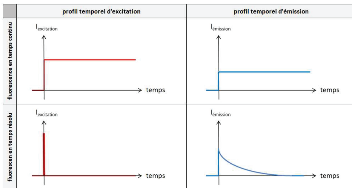
Figure 9 Profils temporels d'excitation et d'émission dans les cas de fluorescence en temps continu et en temps résolu. Source : Réalisation personnelle.
