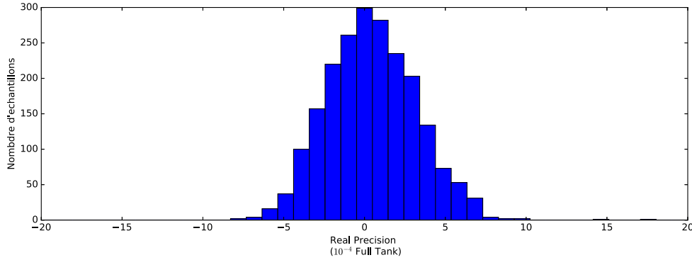
FIGURE III.8: Histogramme de la précision réelle lorsque la valeur mesurée est plus grande que 3000u .
