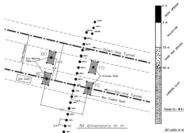
Figure III-22 – Plan d'implantation des pieux et composition du sol – Selemetas et al., (2005)
