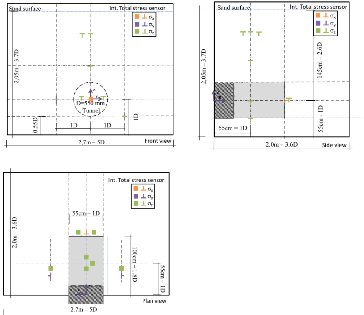
Figure II-26 - Positions génériques des capteurs de contrainte totale
