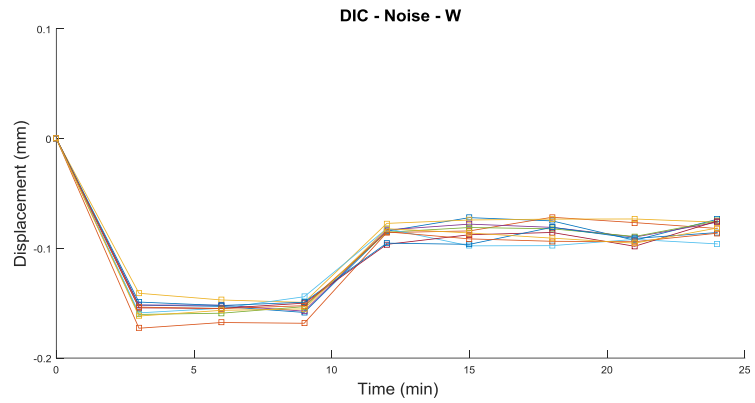
Figure D-3 Réalisation d'un essai de bruit lors de l'analyse de déplacement par DIC
