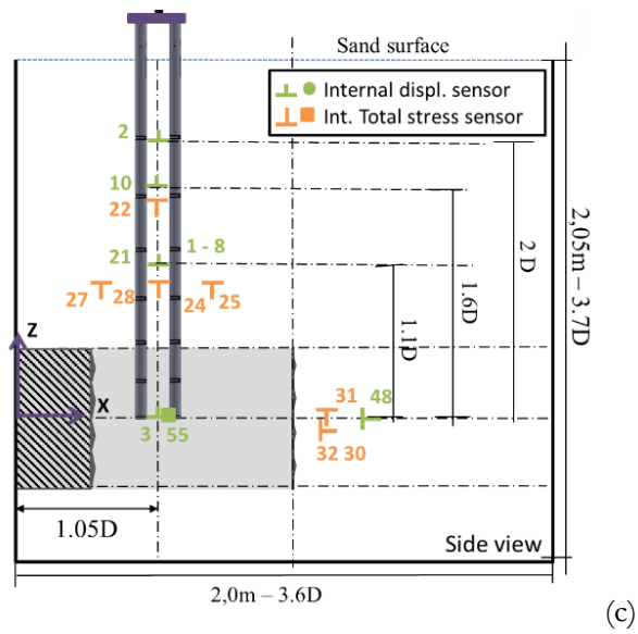
Figure III-53 - Configuration géométrique et instrumentation de l'essai TG2I
