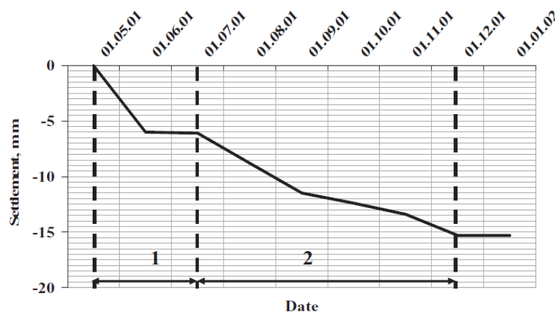
Figure IV-18 Tassement moyen du bâtiment situé au 61/67, Bolshaya Pochtovaya Str. (Moscou), Nikiforova, N. S. et al., (2012) 1 – Installation de la paroi 2 – Excavation du tunnel
