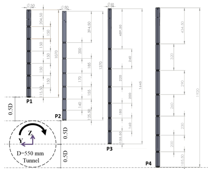
Figure II-37 Schéma des pieux du numéro 1 à 4 (de gauche à droite)
