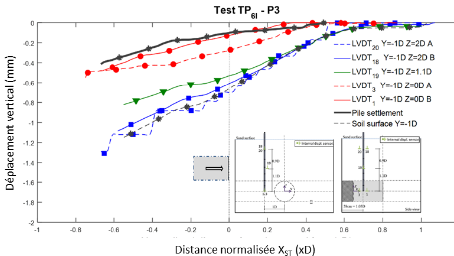
Figure III-81 – Déplacements verticaux du pieu P3 et du sol avoisinant en fonction de l'avancement du tunnelier lors de l'essai TP 6I (A: avant le pieux, B: après le pieu)
