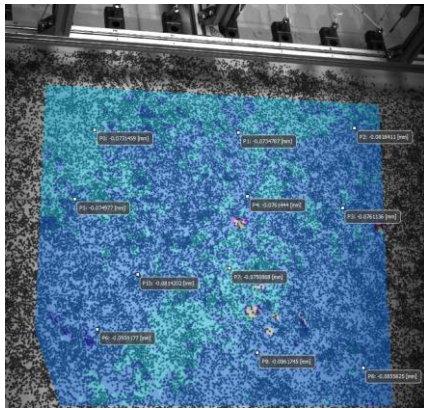
Figure D-3 Réalisation d'un essai de bruit lors de l'analyse de déplacement par DIC
