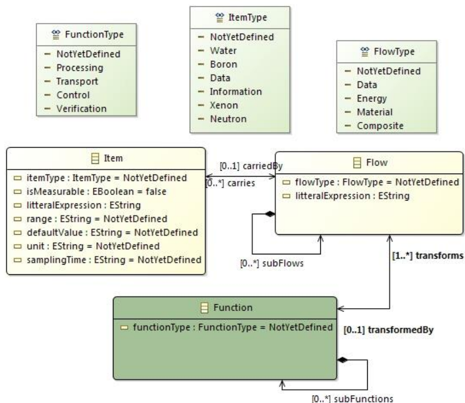
Figure 29: Méta modèle Fonction Flux Item
