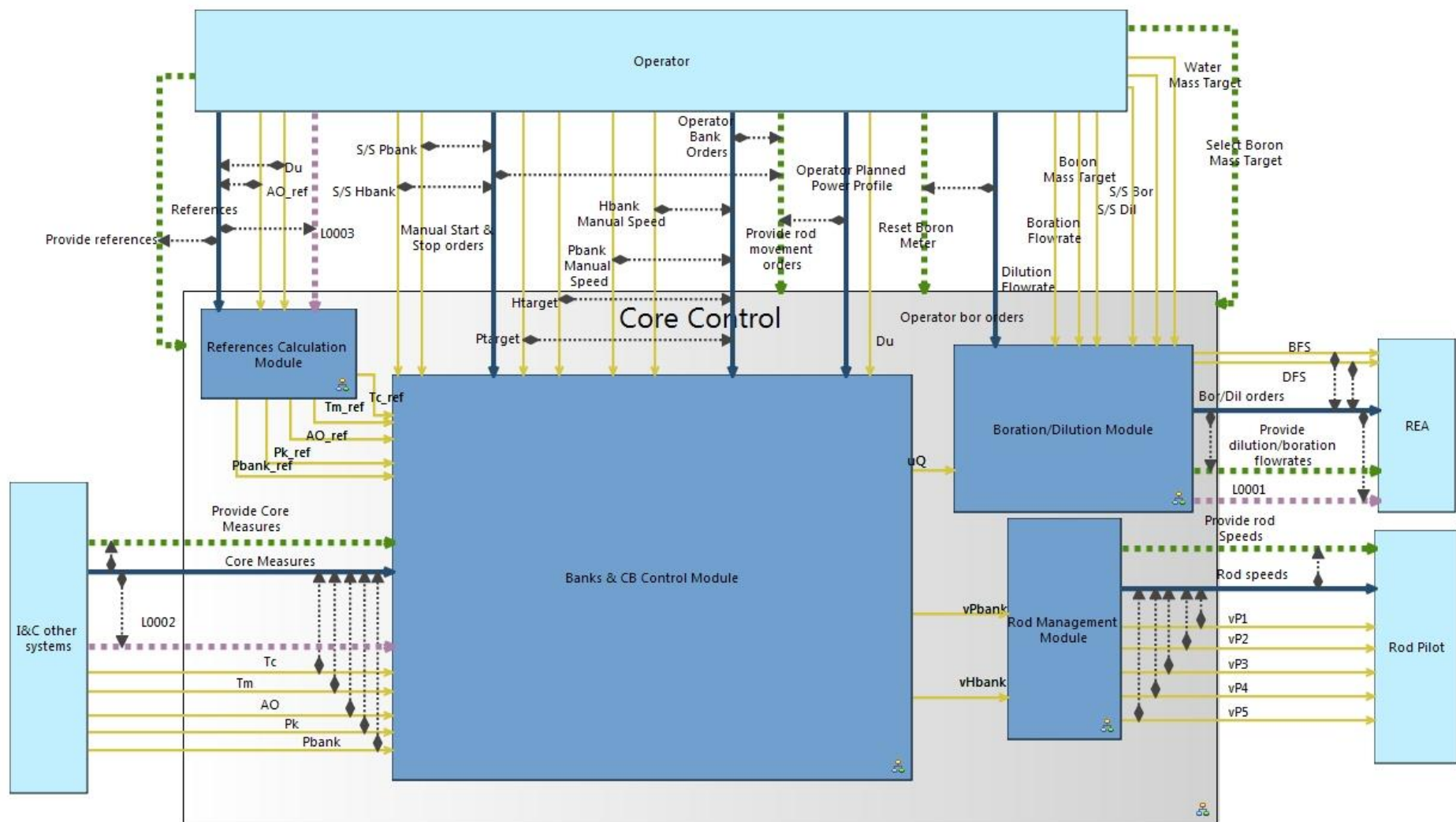
Figure 57: Diagramme de contexte
