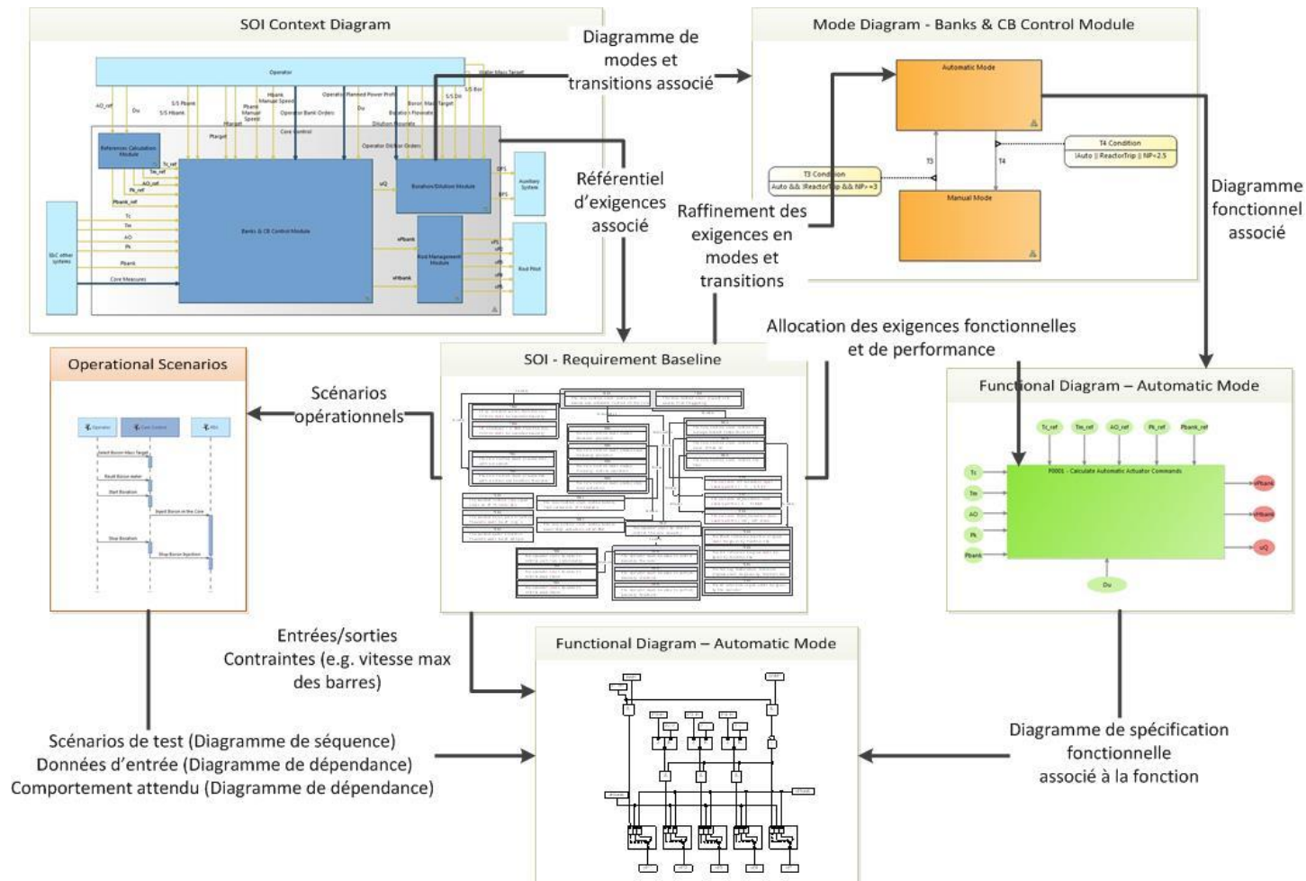
Figure 143: Schéma global des interactions entre les DSML
