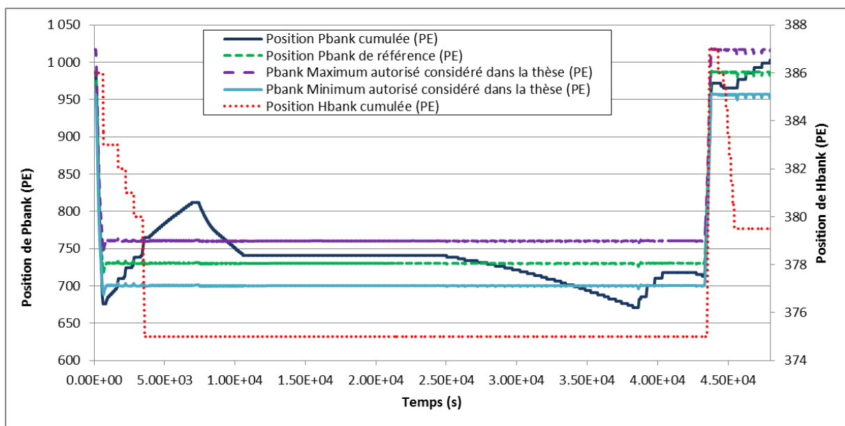
Figure 153: Simulation Mode T – Groupes de grappes Pbank et Hbank - Rampe 100-60-100%PN à 5%/min
