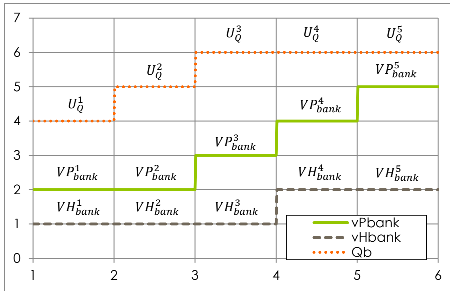
Figure 96: Commandes constantes par morceaux du superviseur
