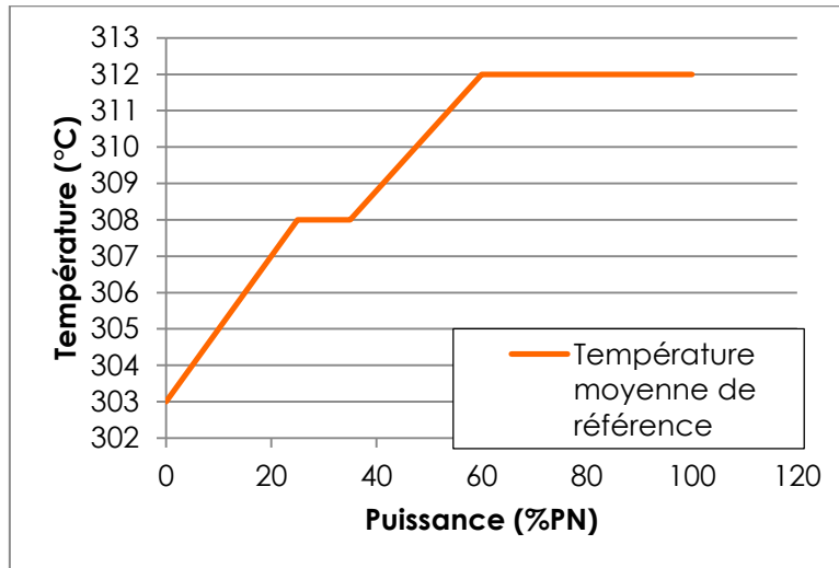
Figure 66: Profil de la température moyenne de référence
