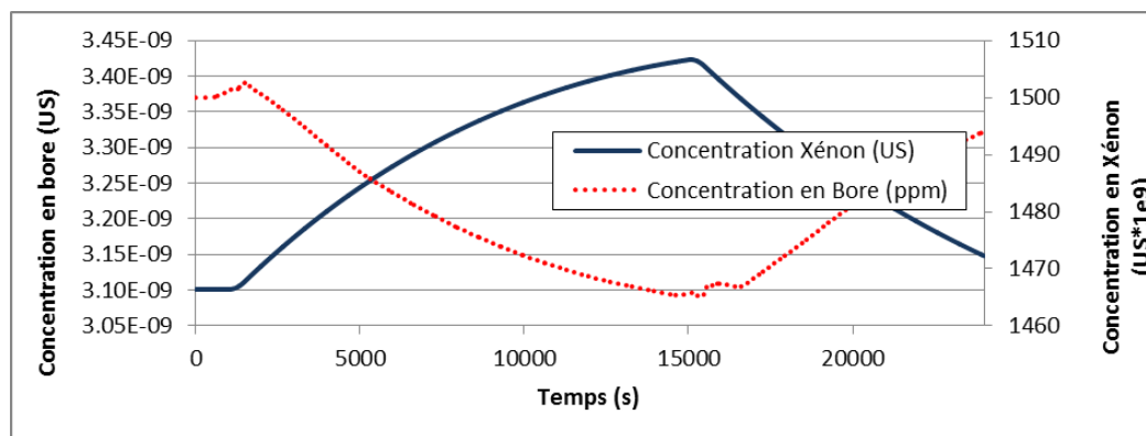
Figure 107: Xénon vs. Concentration en bore - Rampe de puissance 100%PN à 60%PN
