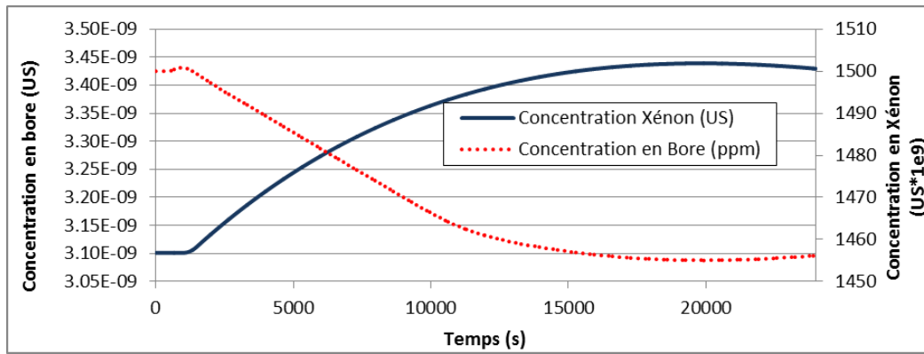
Figure 140: Xénon vs. Concentration en bore - Rampe de puissance 100%PN à 60%PN à 5%PN/min
