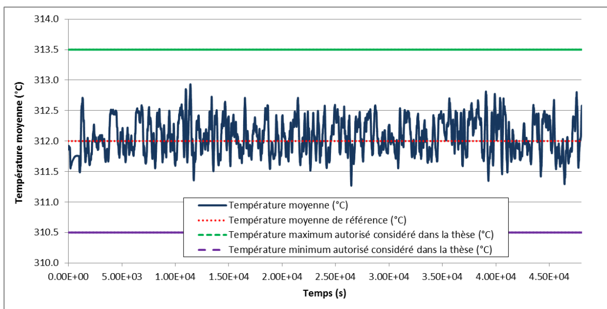
Figure 156: Simulation Mode T – Température moyenne - Réglage de fréquence
