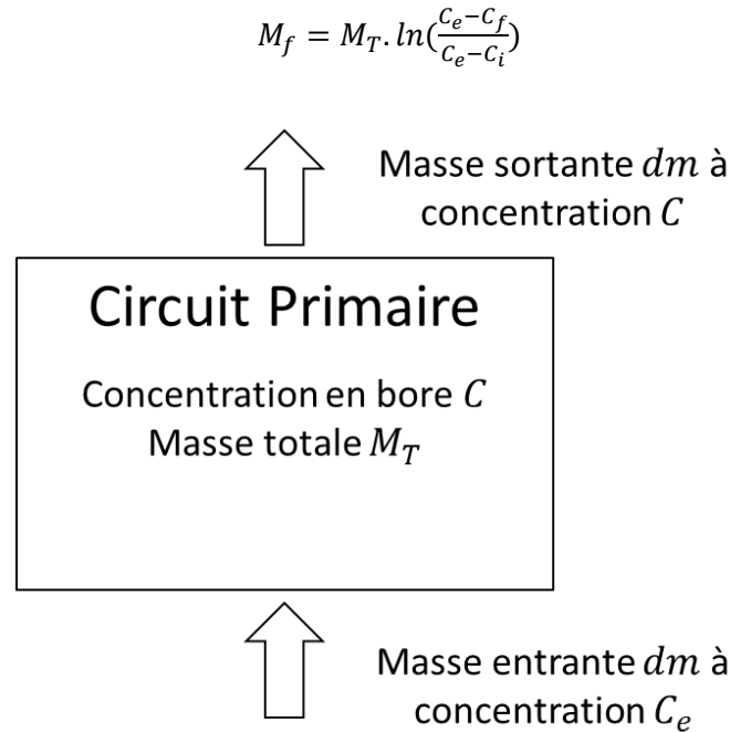
Figure 123: Schématisation du problème de variation de concentration de bore dans le primaire
