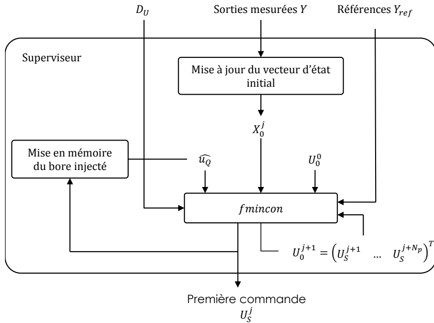
Figure 97: Schéma de principe de l'algorithme du superviseur
