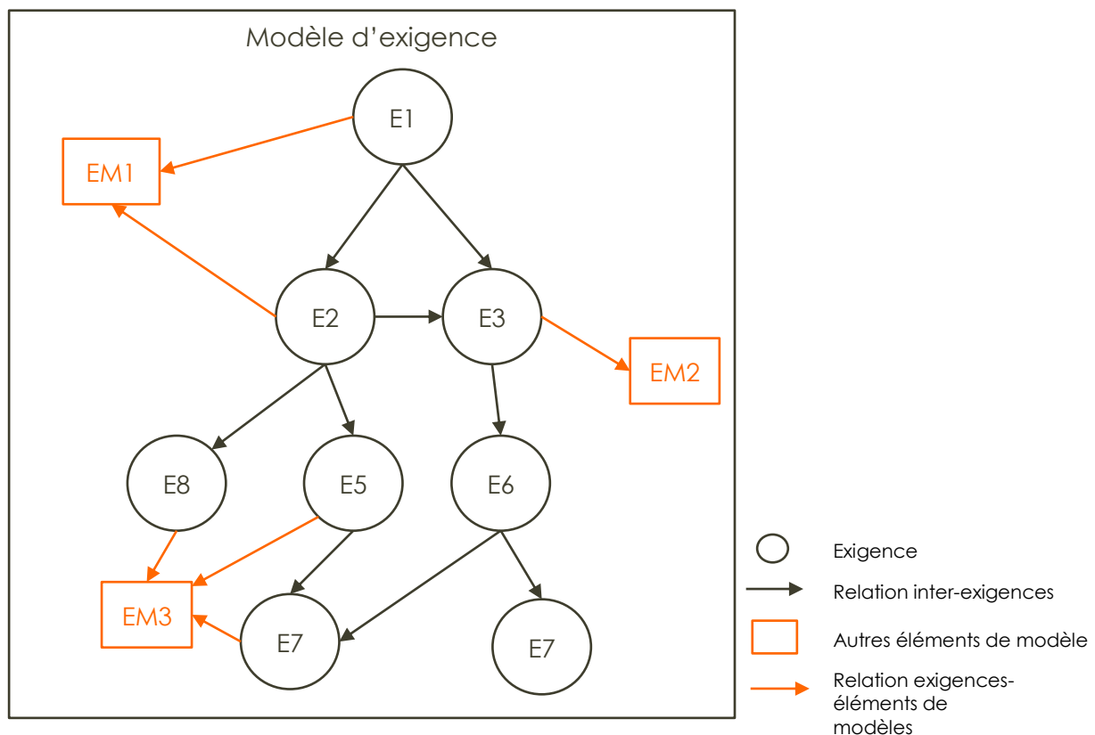
Figure 26: Schéma de principe du modèle d'exigences
