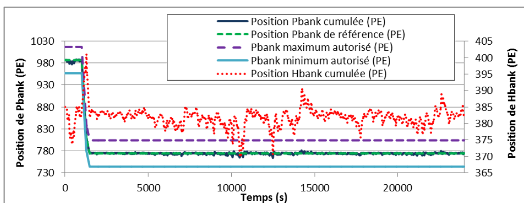
Figure 119: Tracé de la position des groupes - Rampe 100%PN à 70%PN & Réglage de fréquence
