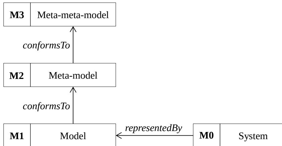
Figure 3 : Les différentes couches de méta modélisation d'OMG
