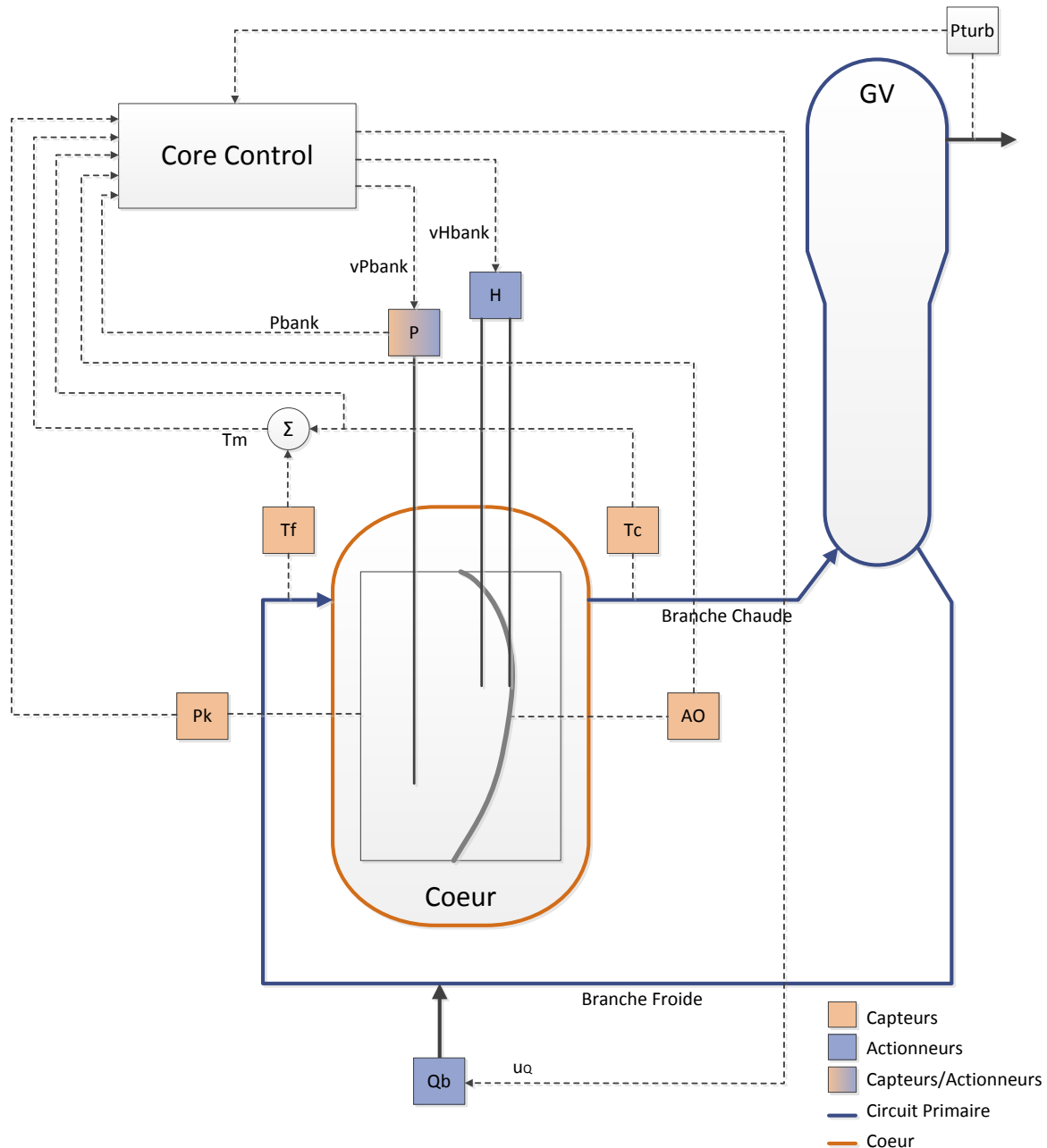
Figure 64: Schéma de principe de la régulation
