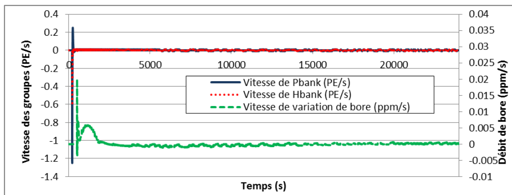
Figure 113: Tracé des vitesses et débit des actionneurs - Step de puissance 100%PN à 90%PN
