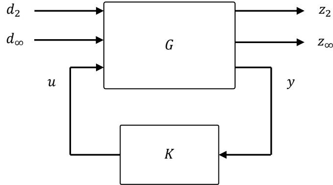
Figure 13: Forme standard de commande dans le cas mixte H_2/H_\infty
