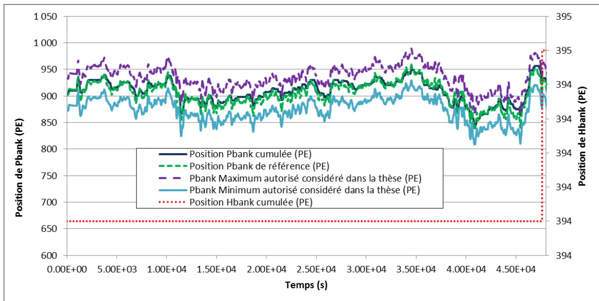
Figure 158: Simulation Mode T – Groupes de grappes Pbank et Hbank - Réglage de fréquence
