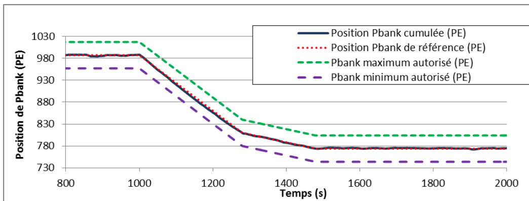
Figure 118: Tracé de la position de Pbank - Rampe 100%PN à 70%PN & Réglage de fréquence
