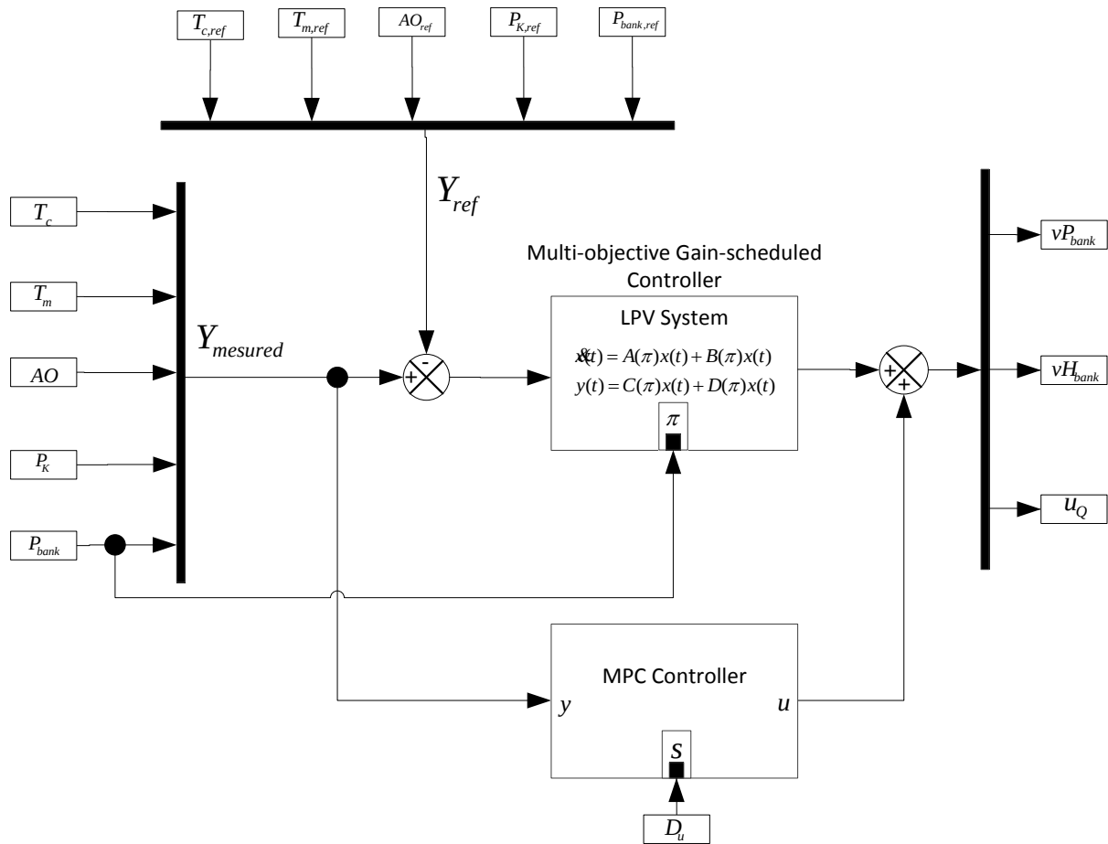
Figure 63: Diagramme de spécification fonctionnelle de la fonction F0001
