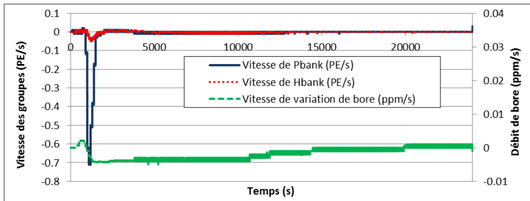
Figure 139: Tracé des vitesses et débit des actionneurs - Rampe de puissance 100%PN à 60%PN à 5%PN/min
