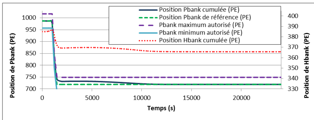
Figure 138: Tracé de la position des groupes - Rampe de puissance 100%PN à 60%PN à 5%PN/min
