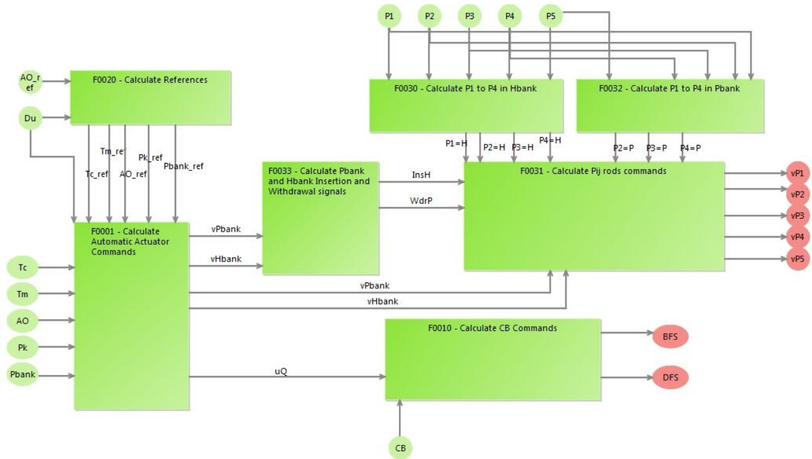
Figure 62: Architecture fonctionnelle du Core Control dans le mode Automatique
