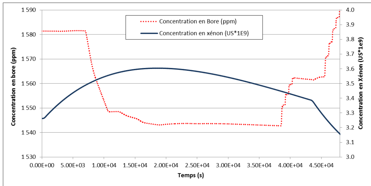
Figure 154: Simulation Mode T – Xénon et Concentration en Bore - Rampe 100-60-100%PN à 5%/min
