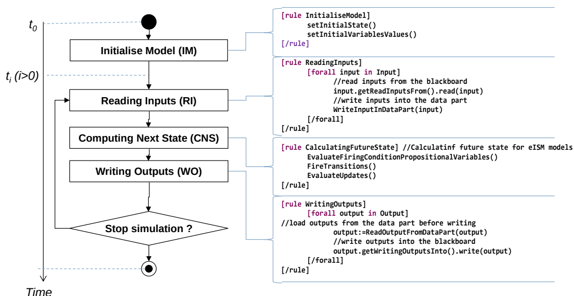
Figure 34 : Moniteur de DSML
