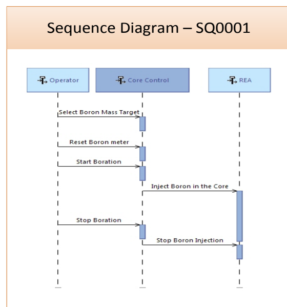
Figure 58: Illustration du diagramme de séquence
