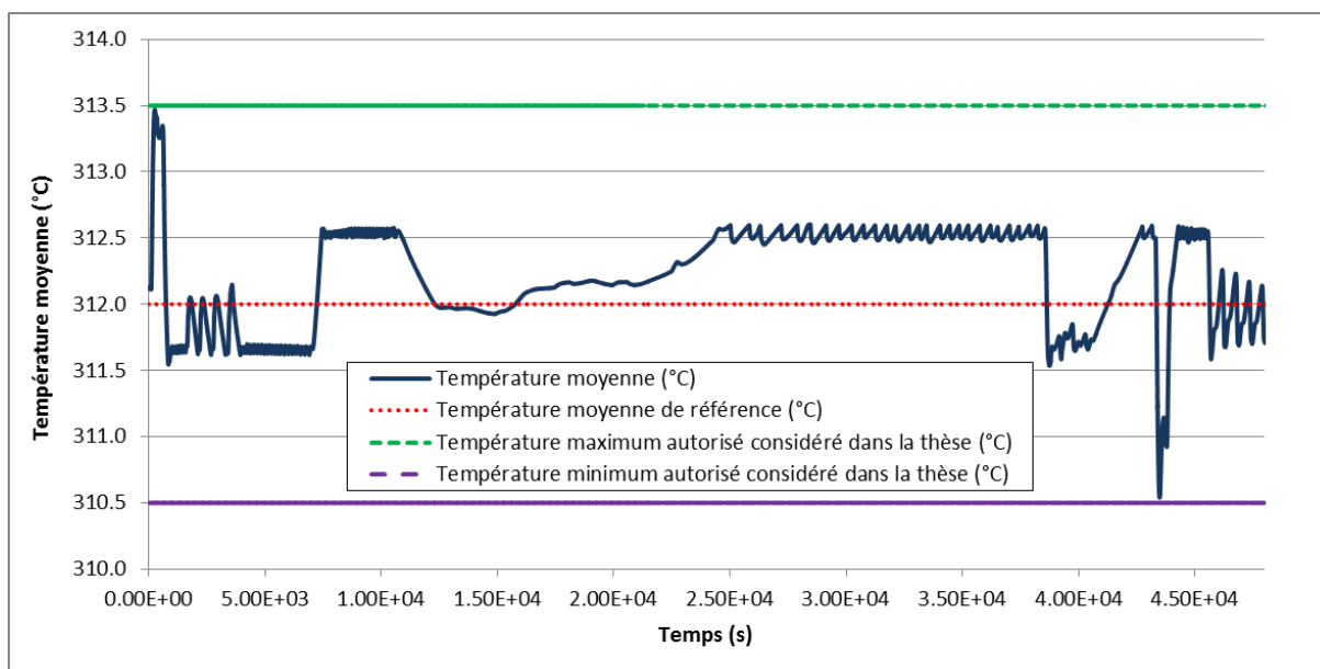
Figure 151: Simulation Mode T – Température moyenne - Rampe 100-60-100%PN à 5%/min
