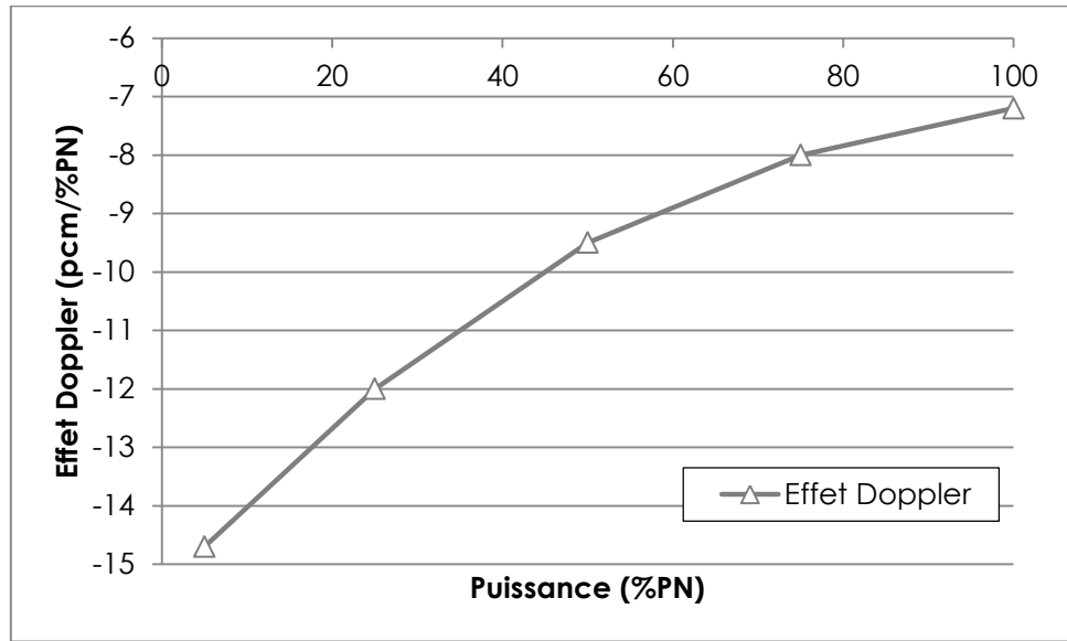
Figure 76: Illustration de l'effet doppler
