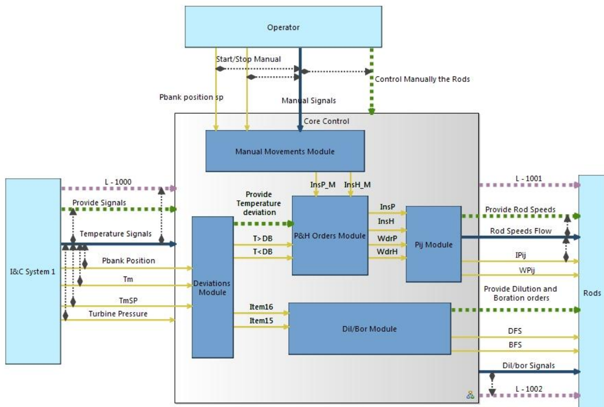
Figure 38: Exemple de diagramme de contexte
