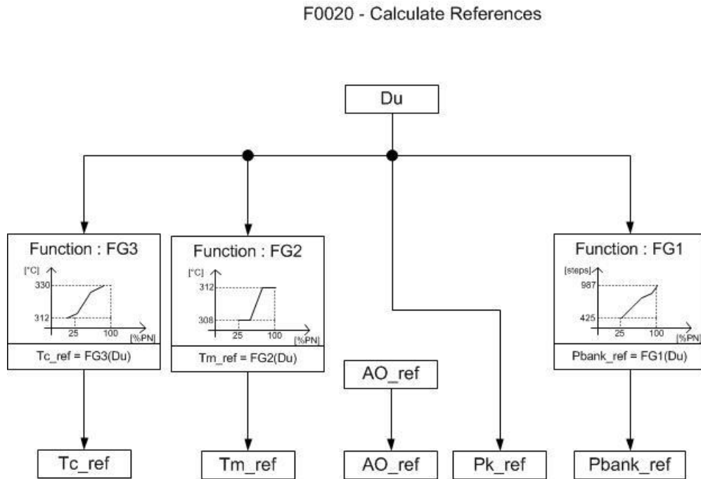
Figure 52: Exemple du langage de spécification I&C Framatome
