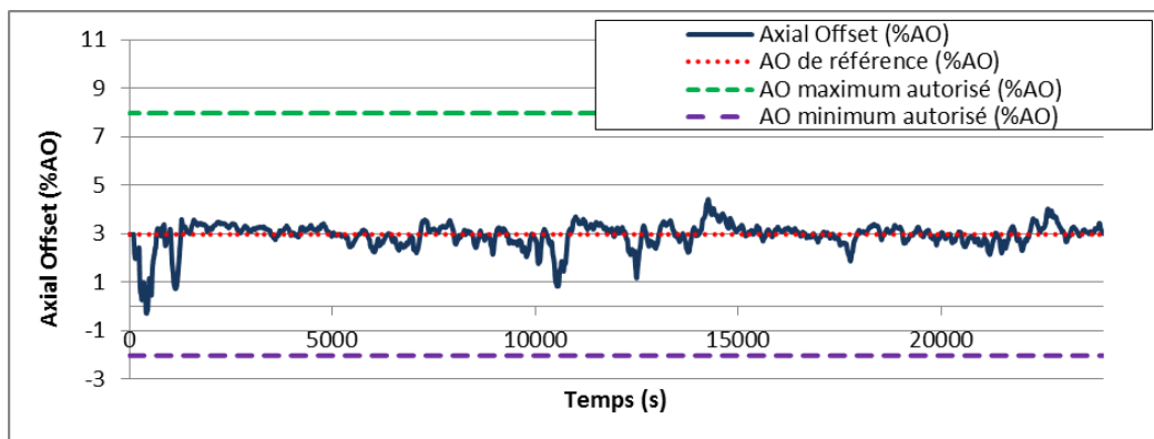
Figure 117: Tracé de l'AO - Rampe 100%PN à 70%PN & Réglage de fréquence
