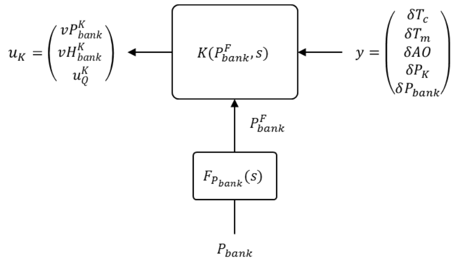
Figure 94: Schéma de séquençement du régulateur à gains séquencés K
