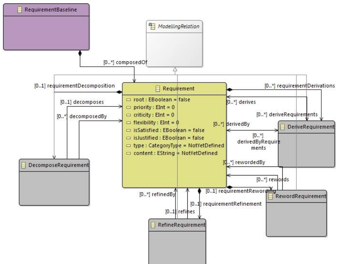
Figure 39: Méta modèle pour le DSML d'exigences
