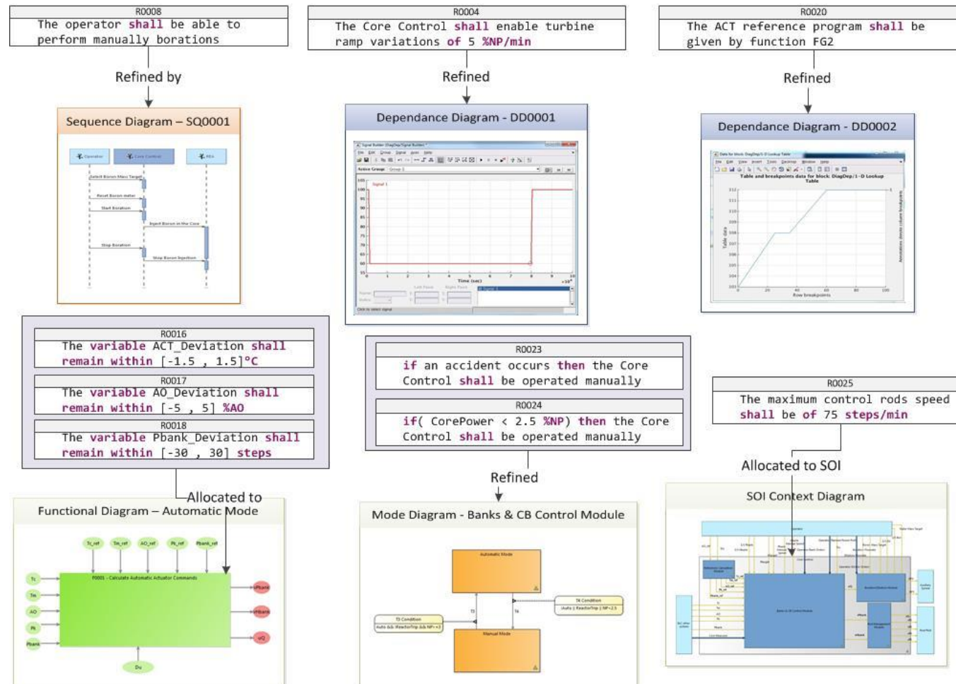
Figure 142 Illustration de l'allocation des exigences
