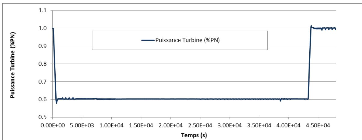
Figure 150: Simulation Mode T - Puissance turbine - Rampe 100-60-100%PN à 5%/min
