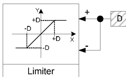
Figure 51: Exemple d'un bloc dans le langage de spécification I&C Framatome ( Limiter )
