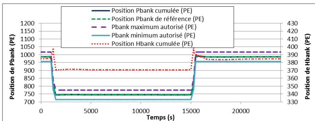
Figure 105: Tracé de la position des groupes - Rampe de puissance 100%PN à 60%PN
