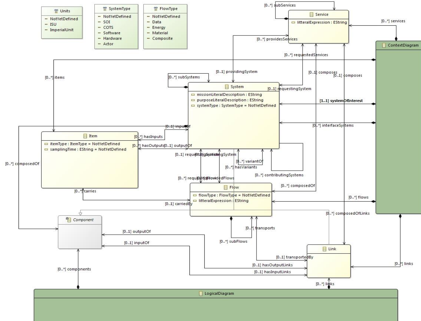
Figure 37: Méta modèle du diagramme de contexte
