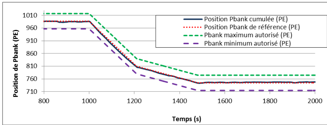
Figure 130: Tracé de la position de Pbank - Rampe de puissance 100%PN à 60%PN à 5%PN/min
