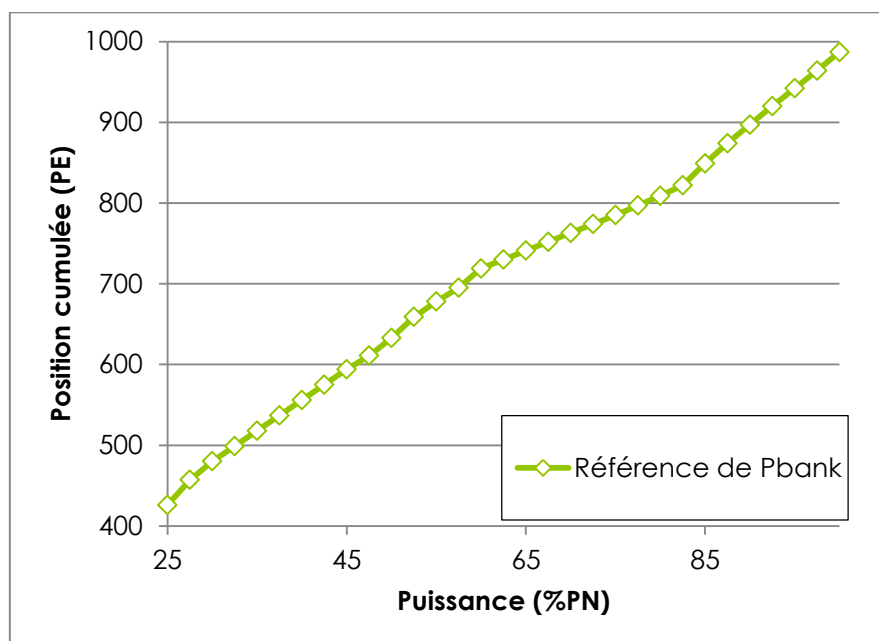
Figure 67: Position de référence pour Pbank (cumulée)
