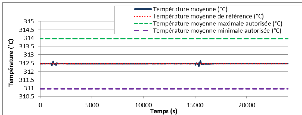
Figure 101: Tracé de la température moyenne - Rampe de puissance 100%PN à 60%PN
