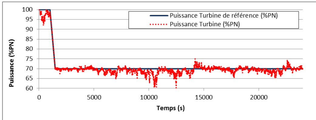
Figure 115: Tracé de la puissance turbine - Rampe 100%PN à 70%PN & Réglage de fréquence
