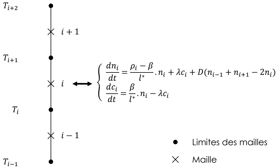
Figure 126: Illustration du couplage thermo-hydraulique des mailles
