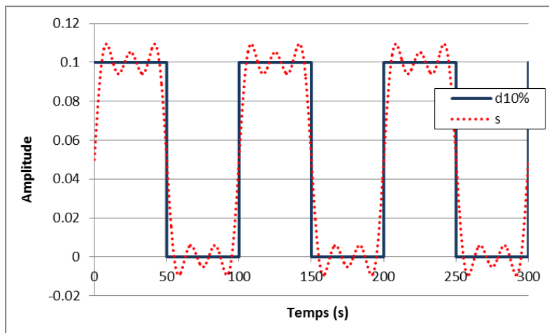
Figure 87: Comparaison signal créneau et décomposition en série de Fourier ordre 3
