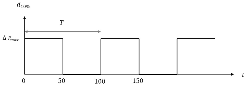
Figure 86: Scénario pire cas de variation de puissance turbine
