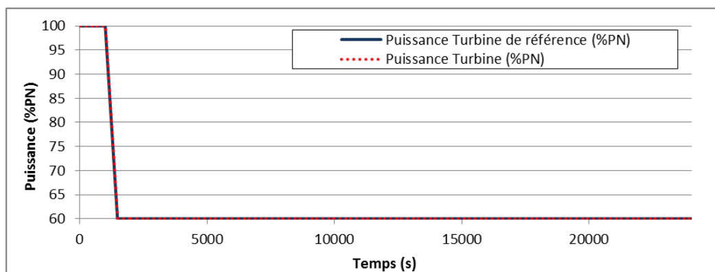
Figure 134: Tracé de la puissance turbine – Rampe de puissance 100%PN à 60%PN à 5%PN/min
