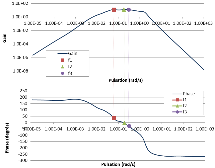
Figure 88: Bode du système considéré
