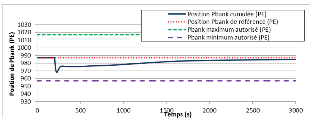
Figure 111: Tracé de la position de Pbank - Step de puissance 100%PN à 90%PN
