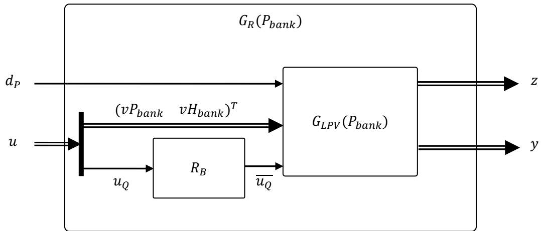
Figure 83: Modèle LPV retardé
