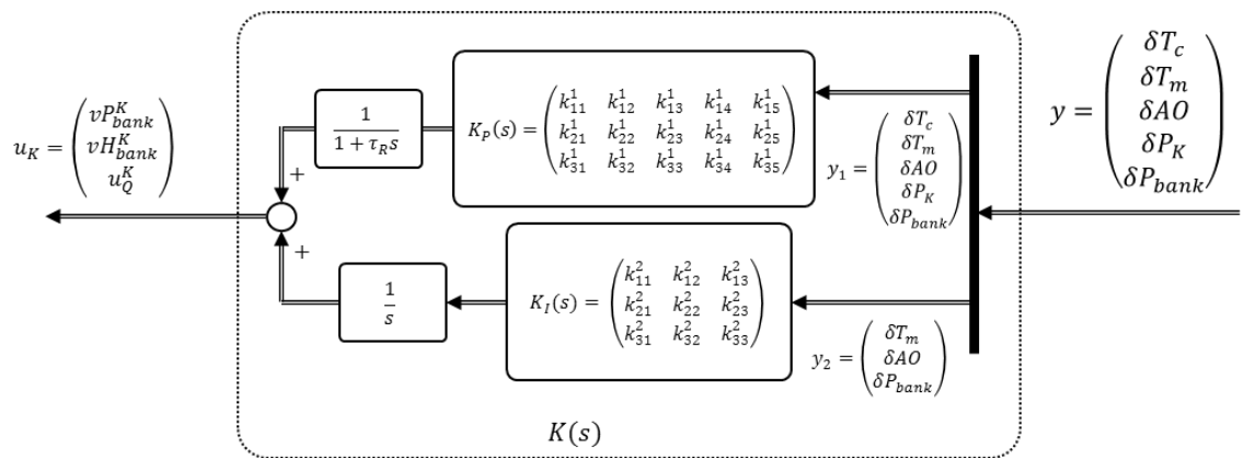
Figure 85: Forme du régulateur multi-objectif
