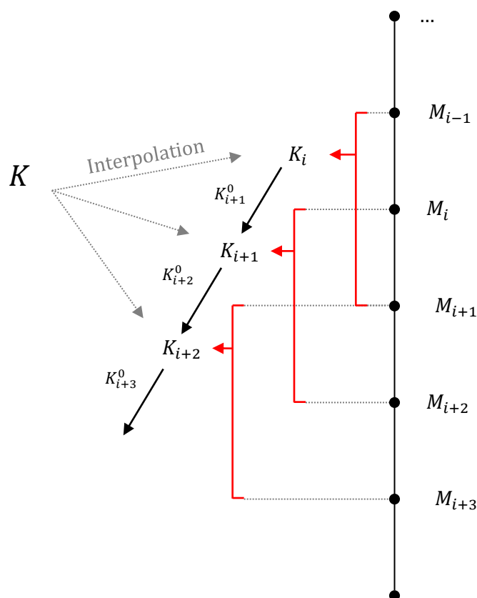
Figure 92: Synthèse multi-modèle par zone
