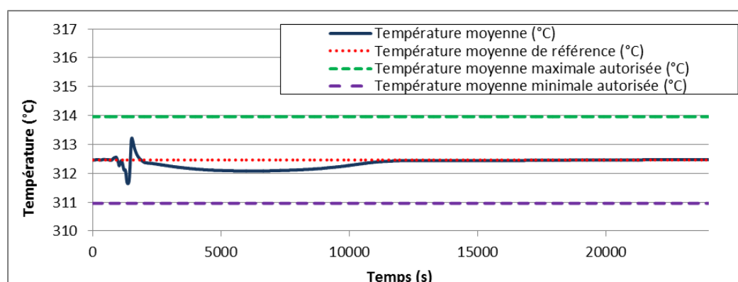
Figure 135: Tracé de la température moyenne - Rampe de puissance 100%PN à 60%PN à 5%PN/min
