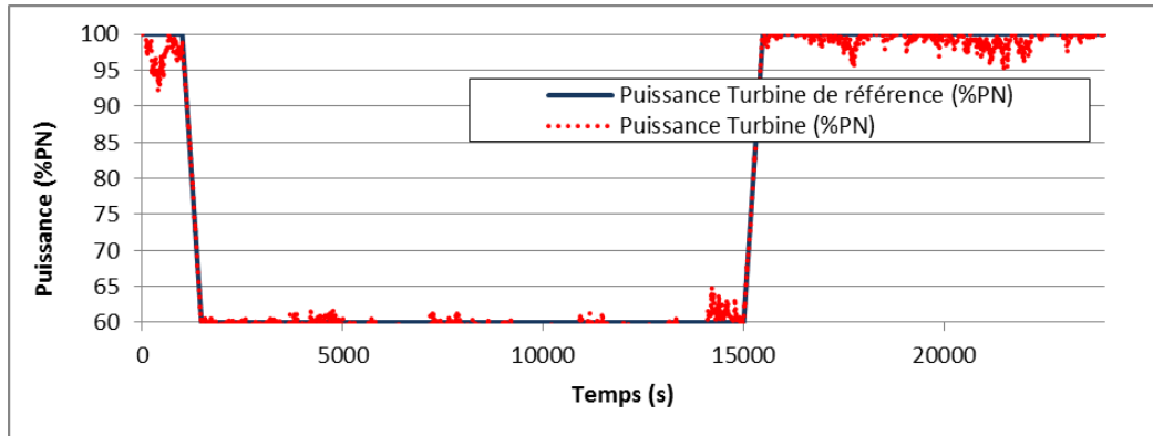
Figure 127: Tracé de la puissance turbine – Rampe de puissance 100%PN à 60%PN à 5%PN/min
