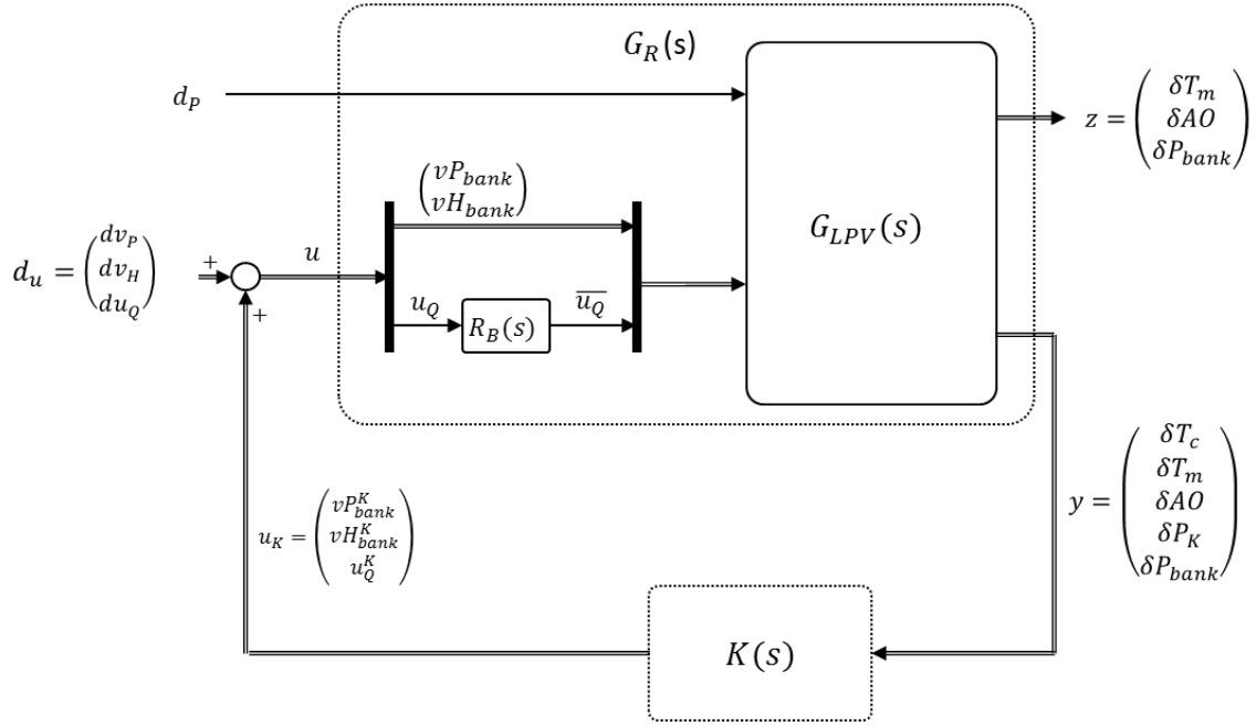
Figure 84: Schéma standard de commande
