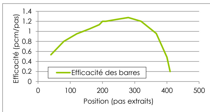
Figure 73: Illustration de l'efficacité ( K_p ) d'un quadruplet de barre en fonction de son insertion (palier TSN – quadruplet PA) – BU150 – E18 7
