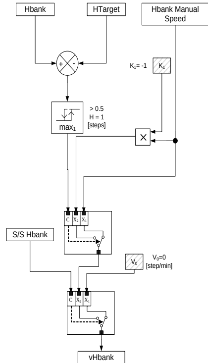
Figure 144 : Diagrammes de Spécification fonctionnelle des fonctions F0002 et F0003
