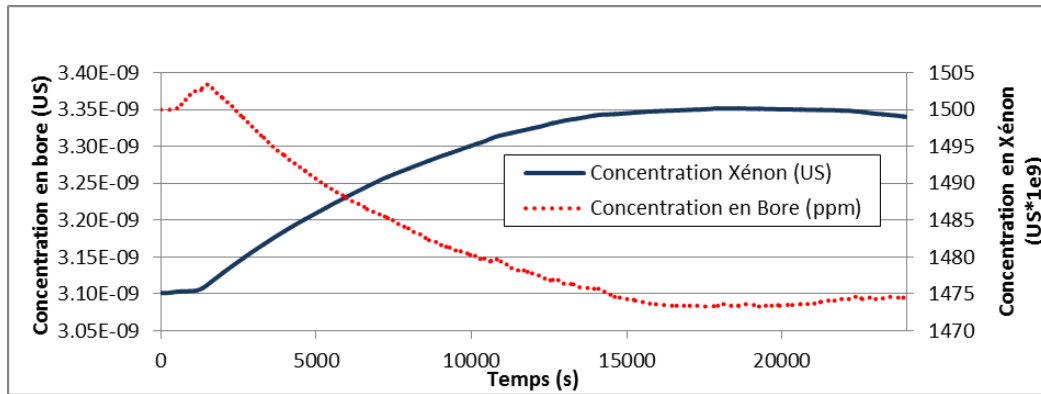
Figure 121: Xénon vs. Concentration en bore - Rampe 100%PN à 70%PN & Réglage de fréquence
