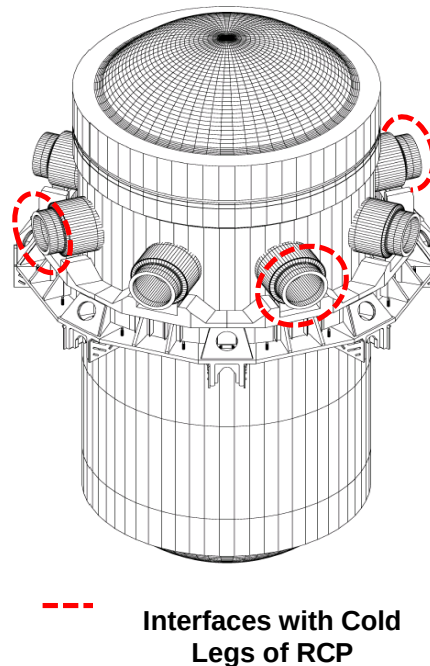
Figure 23: Exemple d'interface – Cœur
