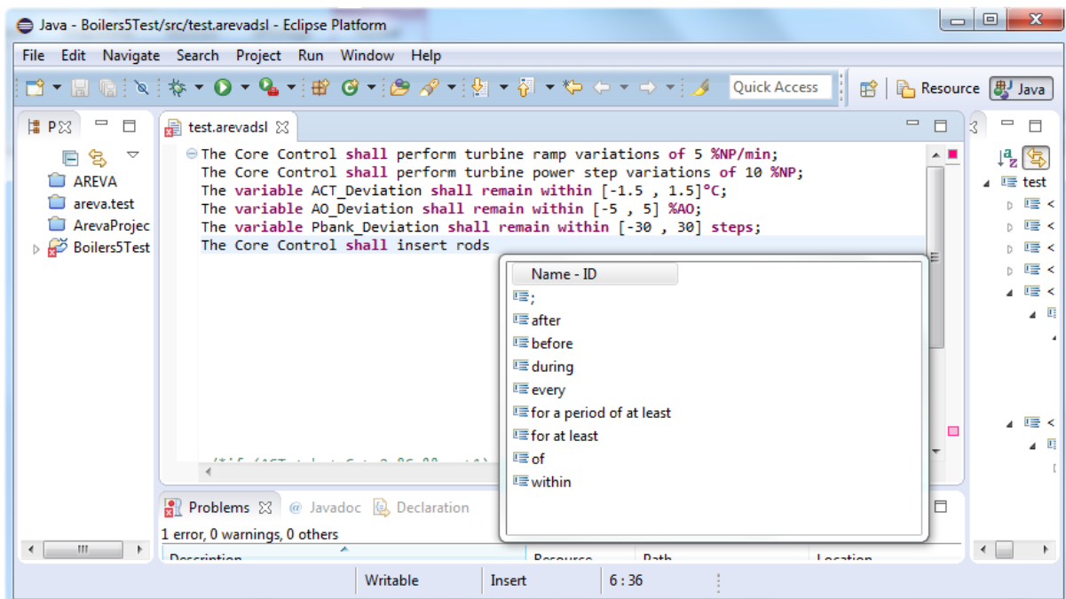
Figure 40: Capture d'écran de l'outil développé pour l'Ingénierie des exigences (avec Xtext)
