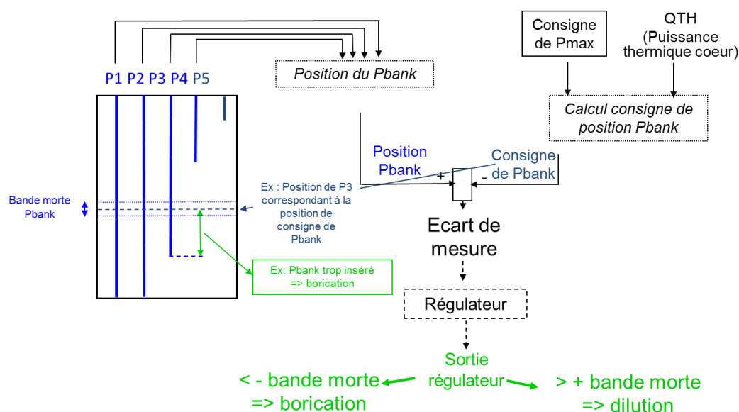
Figure 11: Principe du contrôle du Pmax. Figure tirée de [Grossetête, 2007]
