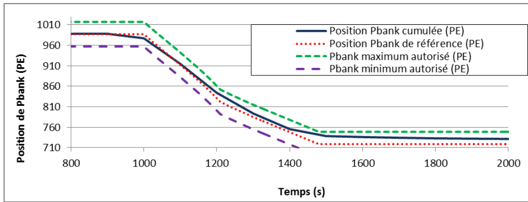
Figure 137: Tracé de la position de Pbank - Rampe de puissance 100%PN à 60%PN à 5%PN/min
