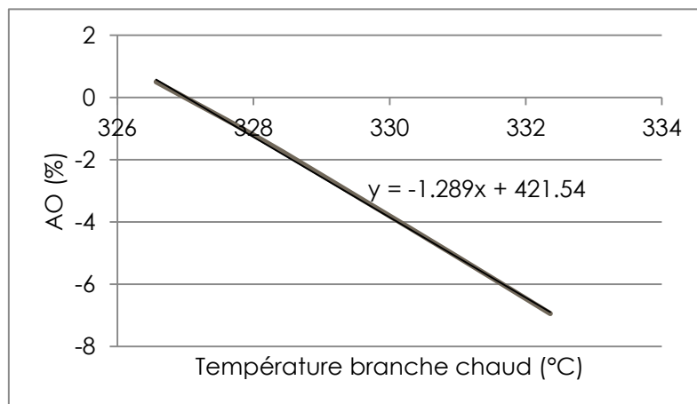
Figure 79: Effet de la température branche chaude sur l'AO à température branche froide constante ( T_f = 295\text{ °C} ) (Données en début de vie)
