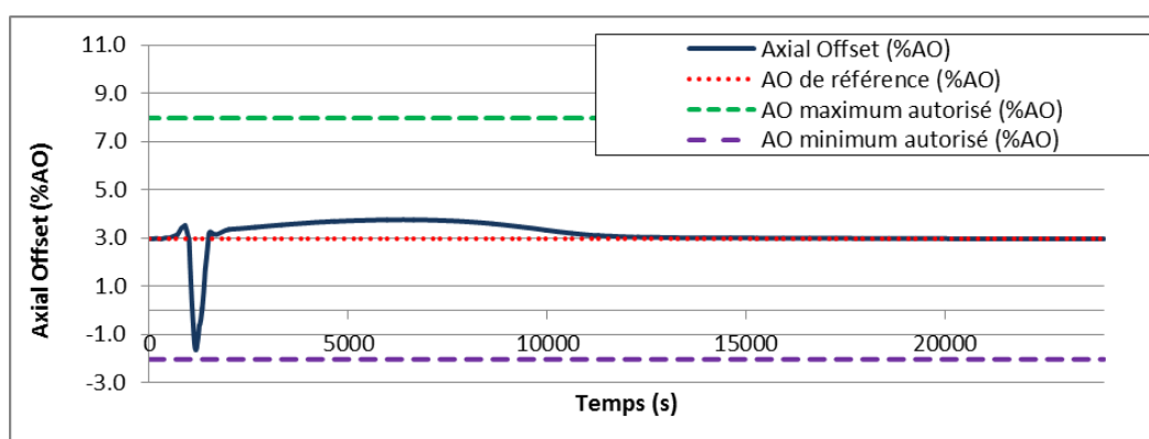
Figure 136: Tracé de l'AO - Rampe de puissance 100%PN à 60%PN à 5%PN/min
