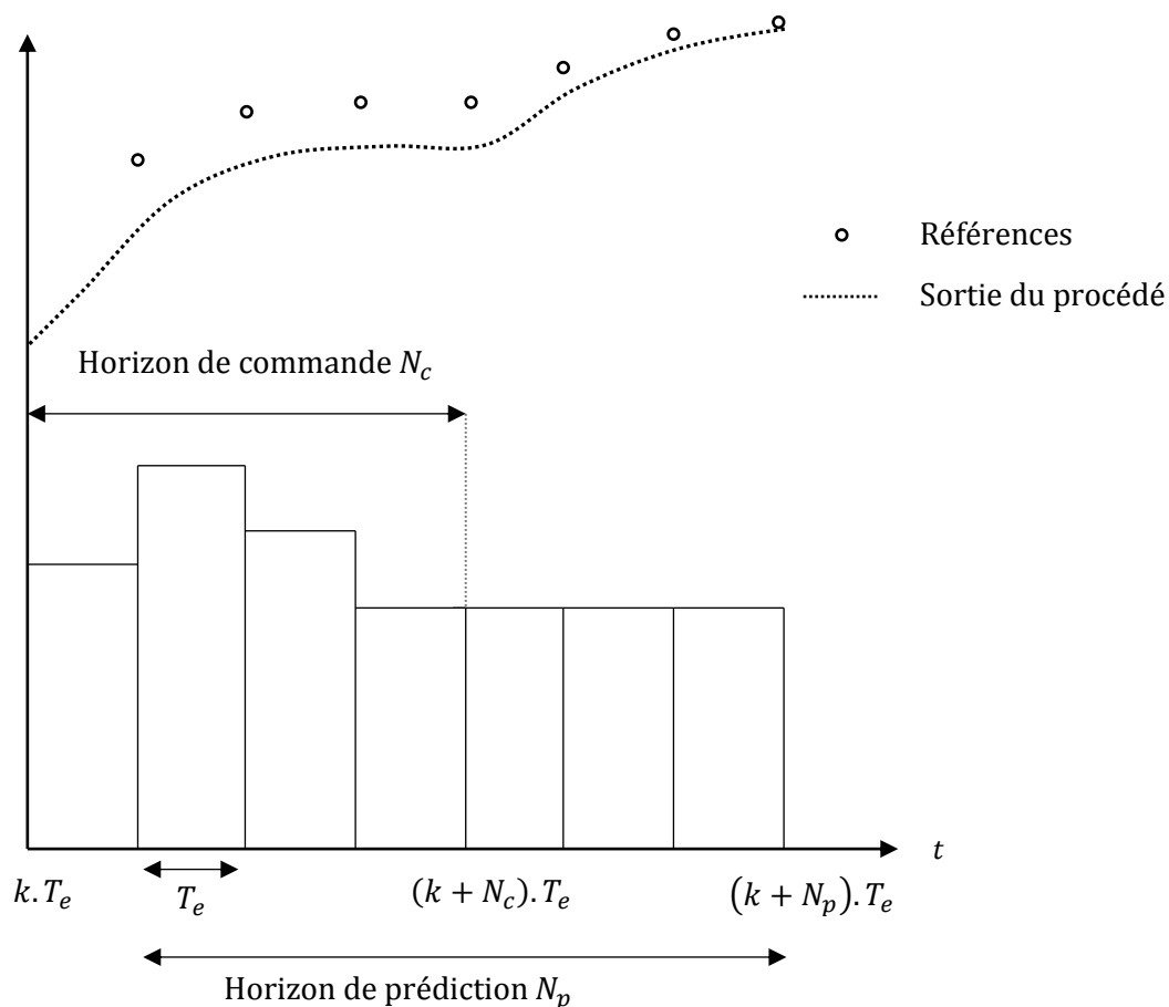
Figure 15: Principe de la commande prédictive
