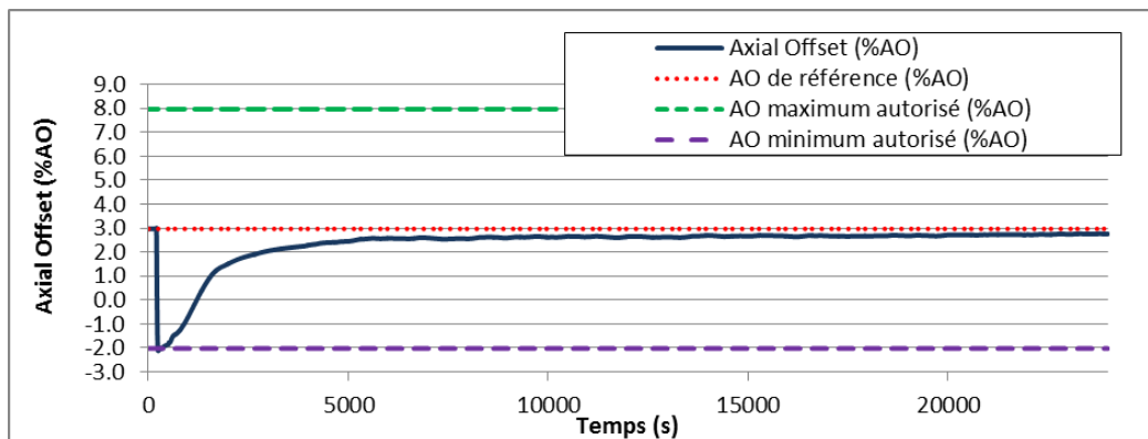
Figure 110: Tracé de l'AO - Step de puissance 100%PN à 90%PN
