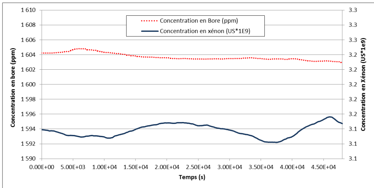
Figure 159: Simulation Mode T – Xénon et Concentration en Bore - Réglage de fréquence
