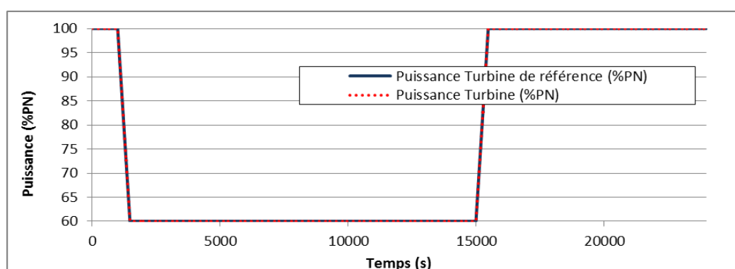
Figure 100: Tracé de la puissance turbine – Rampe de puissance 100%PN à 60%PN
