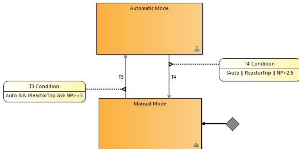
Figure 61 : Diagramme de modes et transition du Core Control
