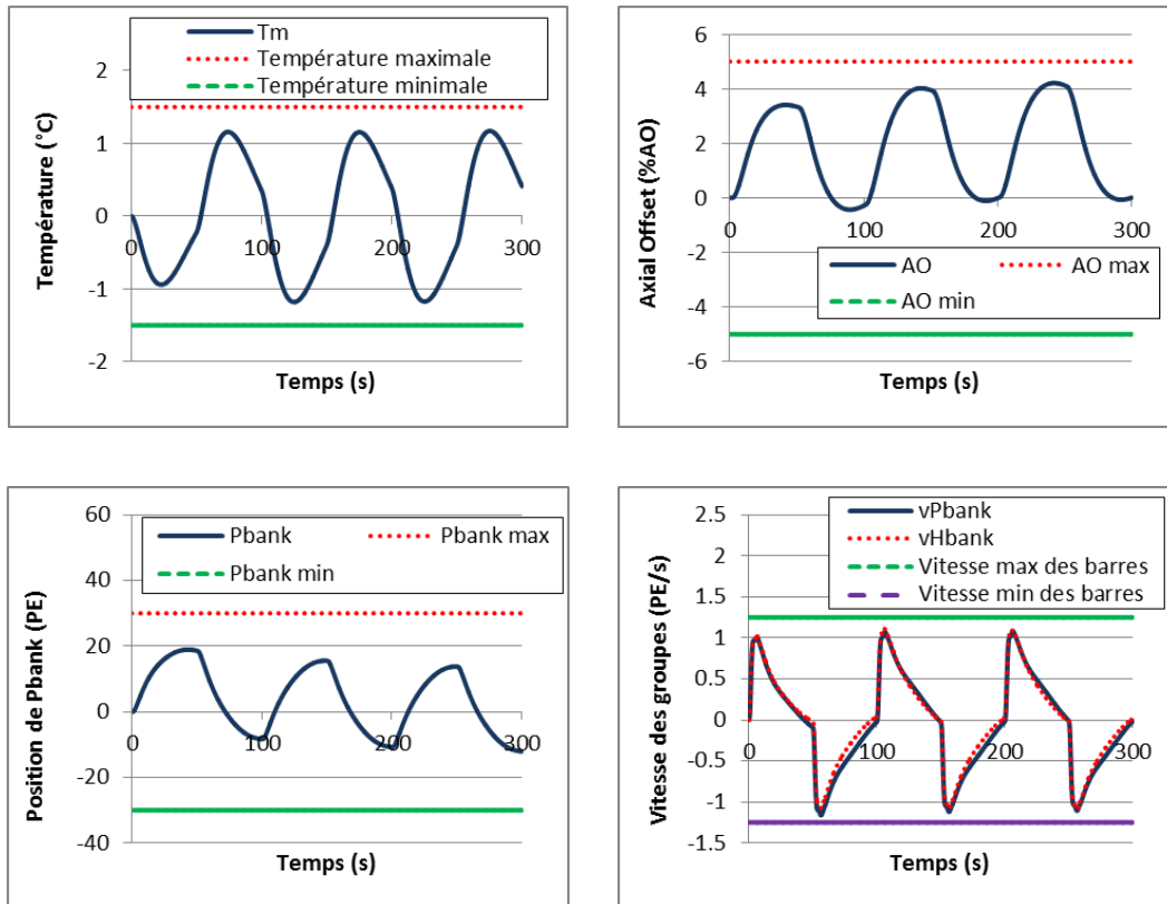
Figure 90: Résultats de simulation d'un régulateur multi-objectif LTI autour d'un point de fonctionnement
