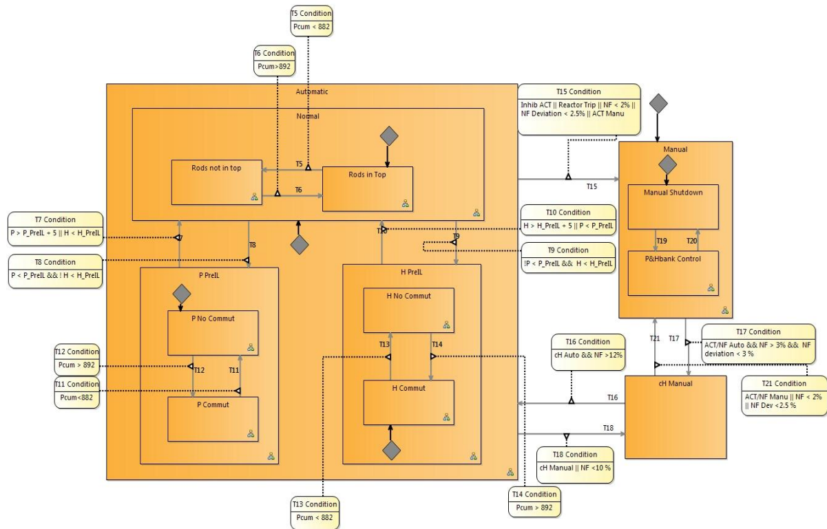
Figure 46: Diagramme de Modes et Transition
