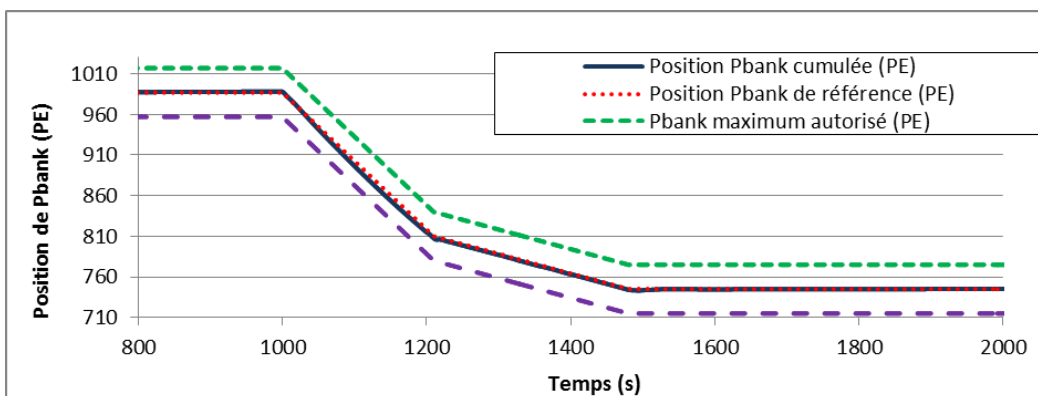
Figure 103: Tracé de la position de Pbank - Rampe de puissance 100%PN à 60%PN – Descente de charge
