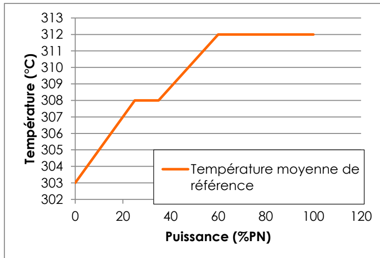
Figure 9: Programme de température moyenne
