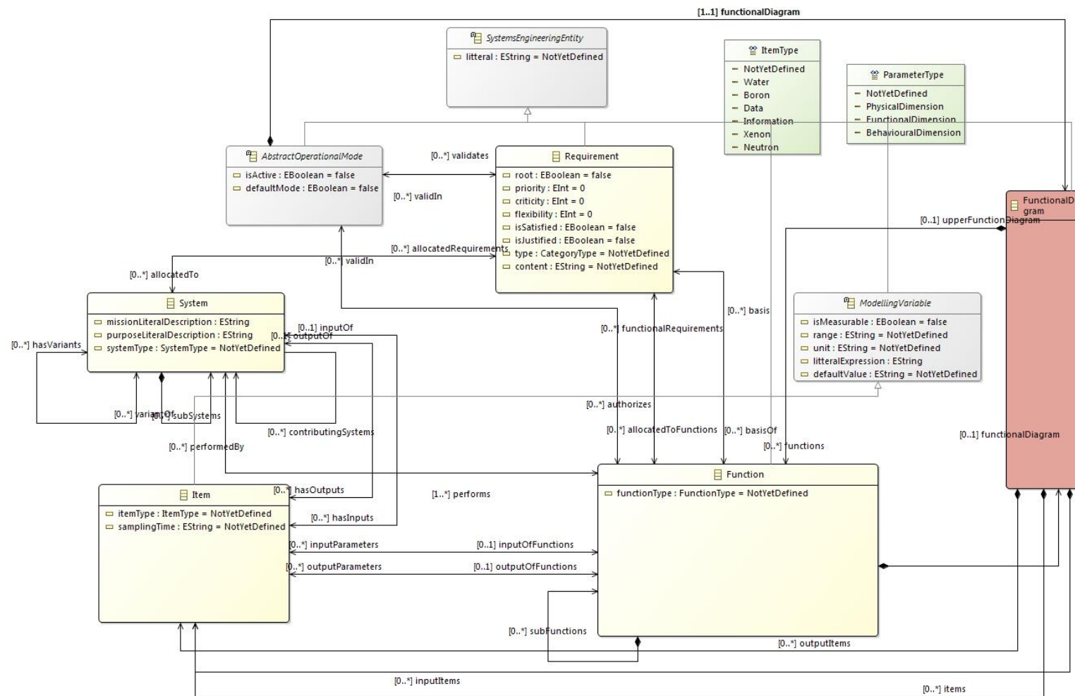
Figure 49: Méta modèle du diagramme fonctionnel
