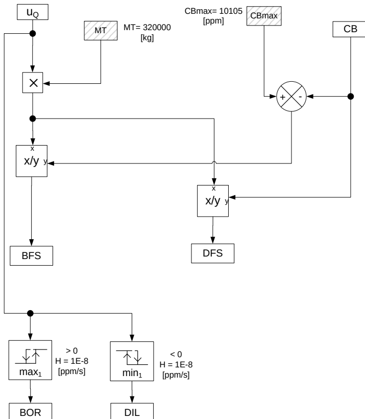
Figure 147: Diagramme de spécification fonctionnelle de la fonction F0010
