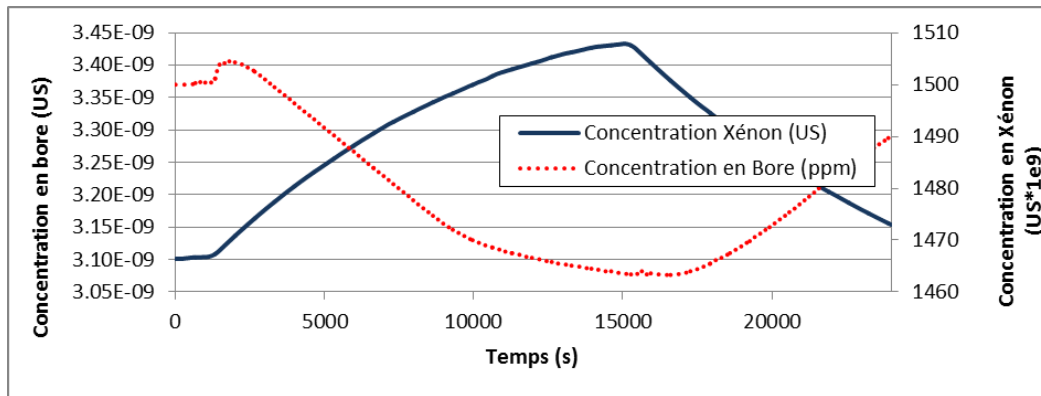
Figure 133: Xénon vs. Concentration en bore - Rampe de puissance 100%PN à 60%PN à 5%PN/min
