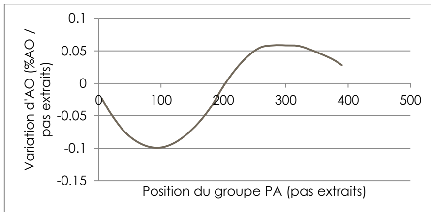
Figure 78: Effet de la barre PA sur l'AO (Données SMART – Palier TSN – Cycle E18 – BU150 – AO initial -3%)
