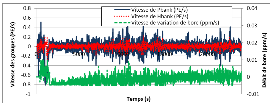
Figure 120: Tracé des vitesses et débit des actionneurs - Rampe 100%PN à 70%PN & Réglage de fréquence
