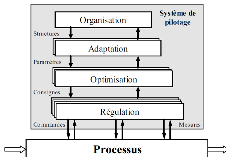
Figure 69: Commande hiérarchisée
