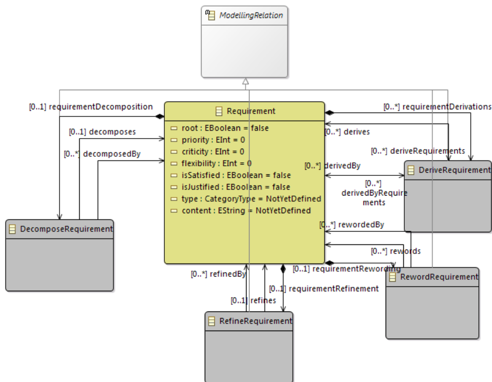
Figure 28: Méta modèle de l'Exigence et ses relations
