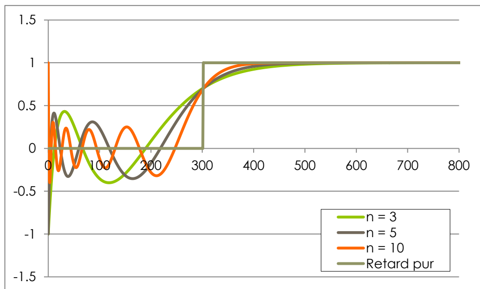
Figure 81: Réponse indicielle de l'approximant de Laguerre
