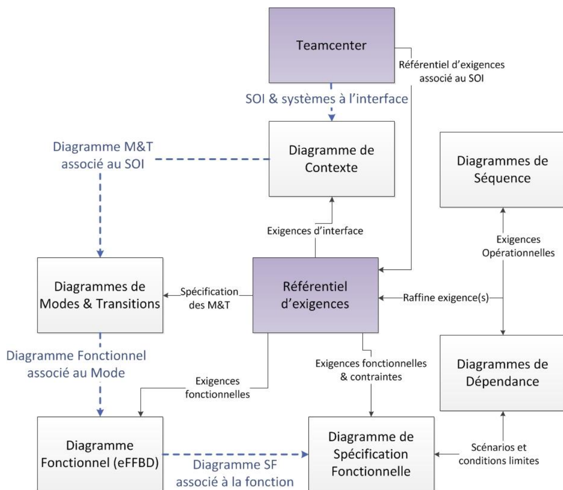
Figure 53: Liens entre les différents langages utilisés
