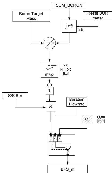
Figure 145: Diagrammes de spécification fonctionnelle des fonctions F0004 et F0005
