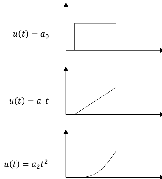
Figure 14: Base de fonctions pour la commande prédictive
