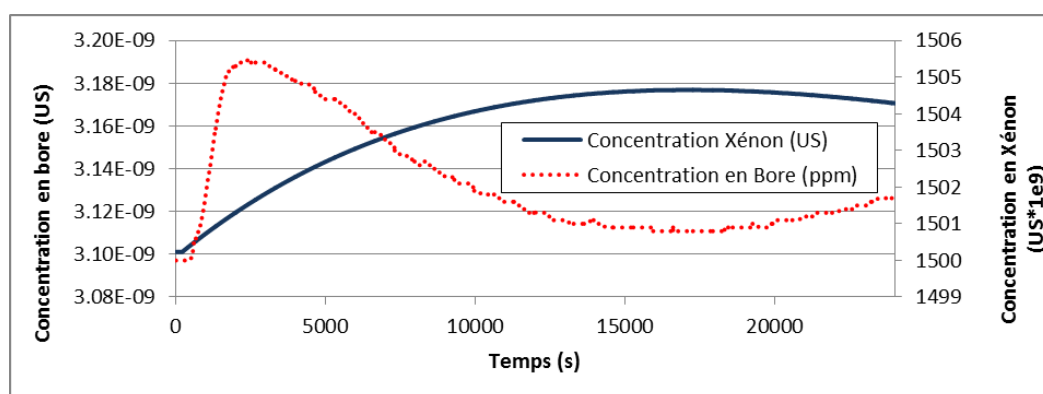
Figure 114: Xénon vs. Concentration en bore - Step de puissance 100%PN à 90%PN
