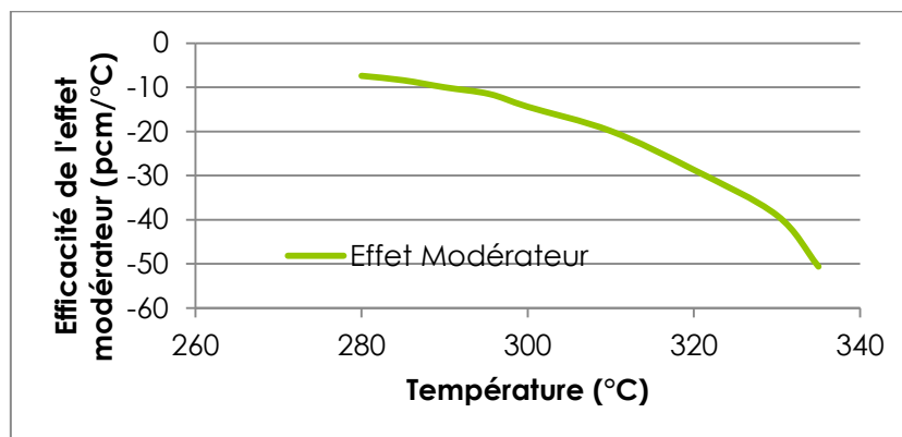
Figure 75: Efficacité de l'effet modérateur en fonction de la température
