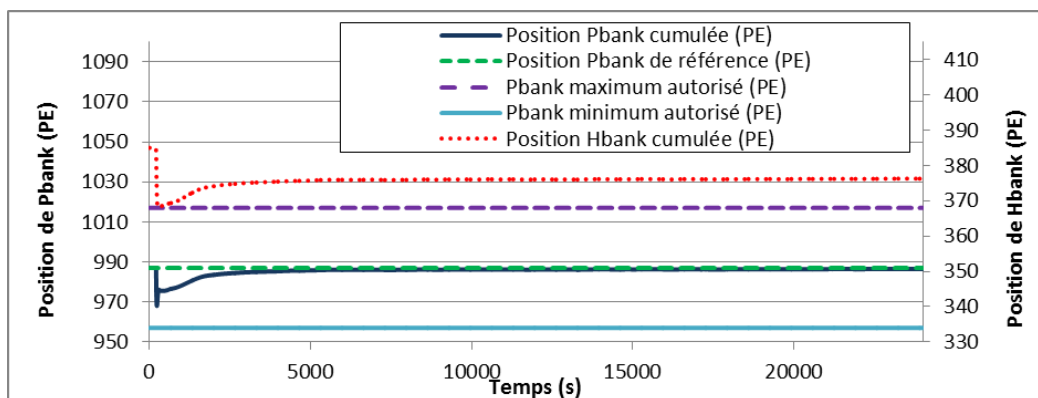
Figure 112: Tracé de la position des groupes - Step de puissance 100%PN à 90%PN
