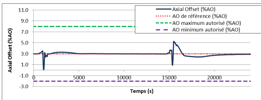
Figure 102: Tracé de l'AO - Rampe de puissance 100%PN à 60%PN
