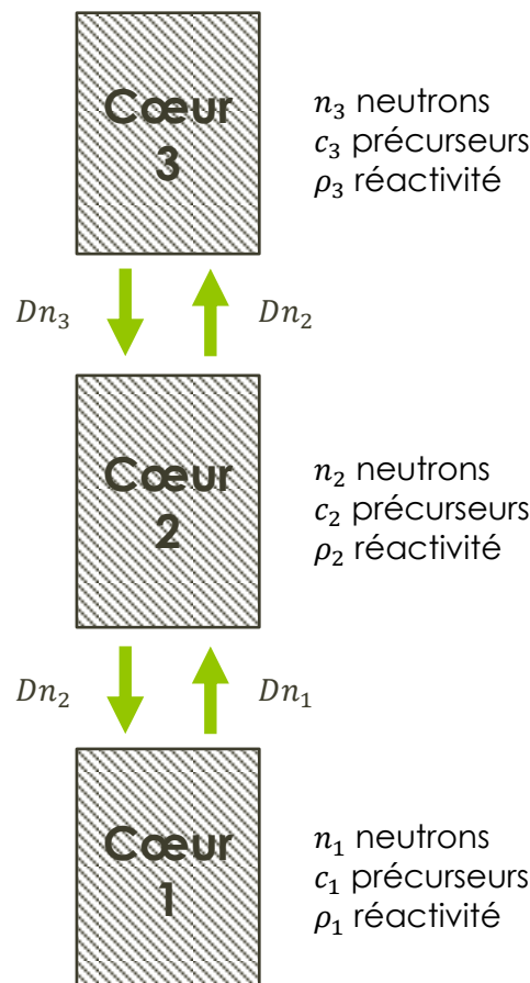
Figure 125: Illustration du principe de la modélisation
