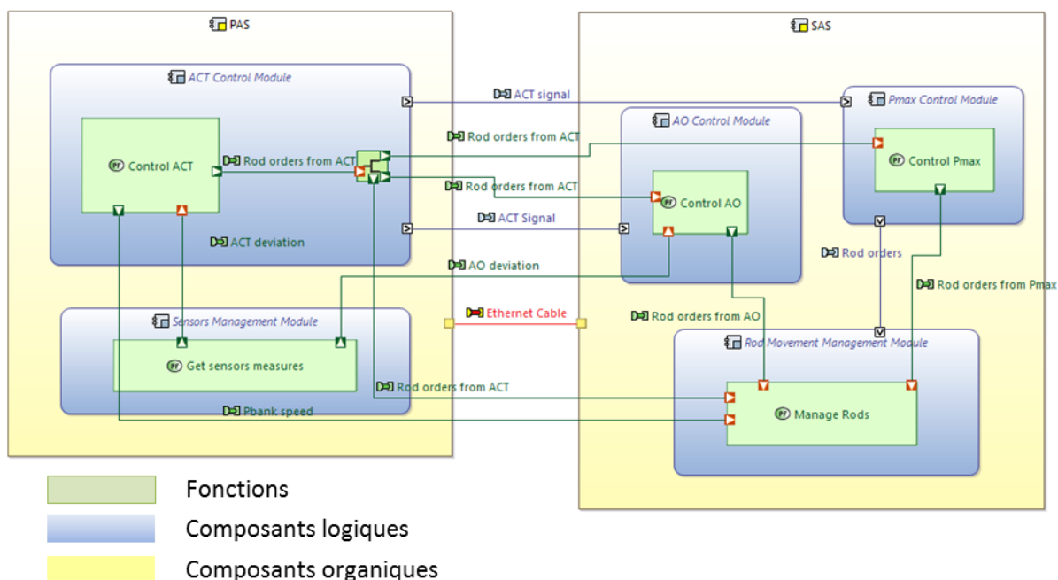
Figure 31: Représentation des liens entre les architectures
