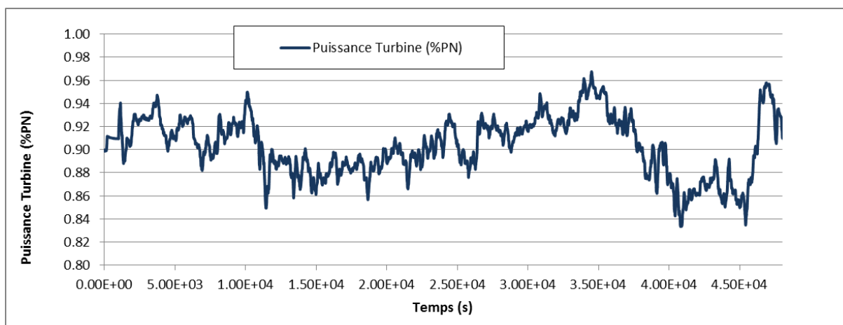
Figure 155: Simulation Mode T – Puissance turbine - Réglage de fréquence
