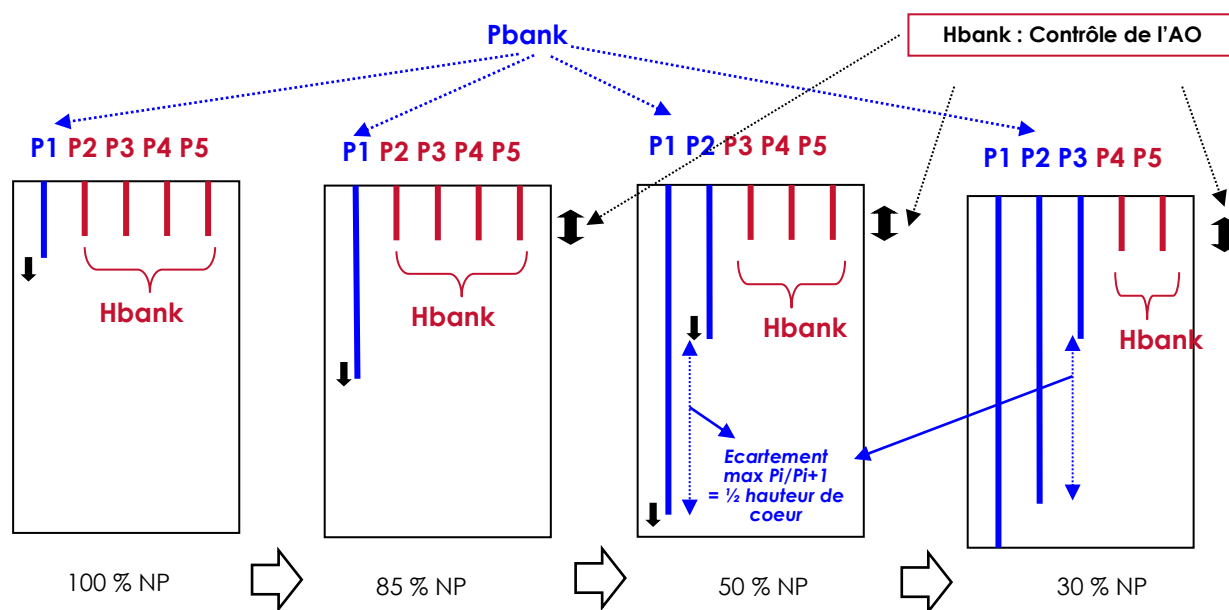
Figure 8 : Mouvement typique des groupes lors d'une variation de puissance. Figure tirée de [Grossetête, 2007]
