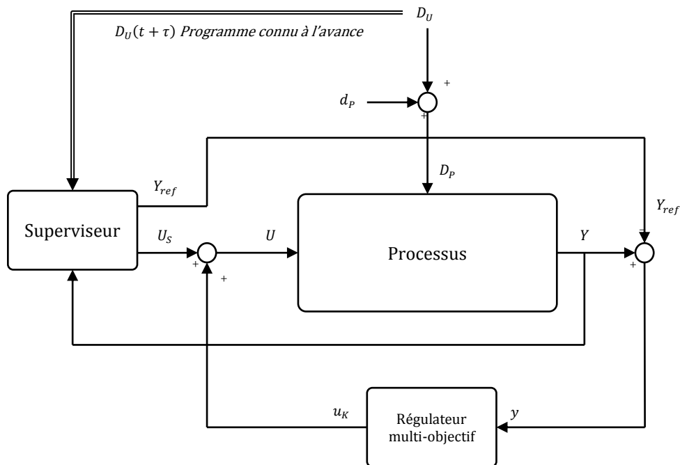
Figure 70: Schéma de principe de la régulation adoptée
