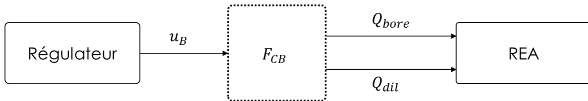
Figure 124: Schéma bloc de la conversion de commande de bore
