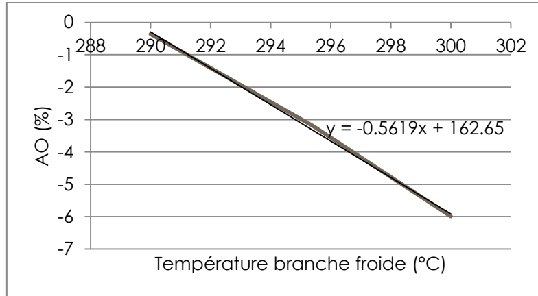
Figure 80 : Effet de la température branche froide sur l'AO à température branche chaude constante ( T_c = 329^\circ\text{C} ) (Données en début de vie)
