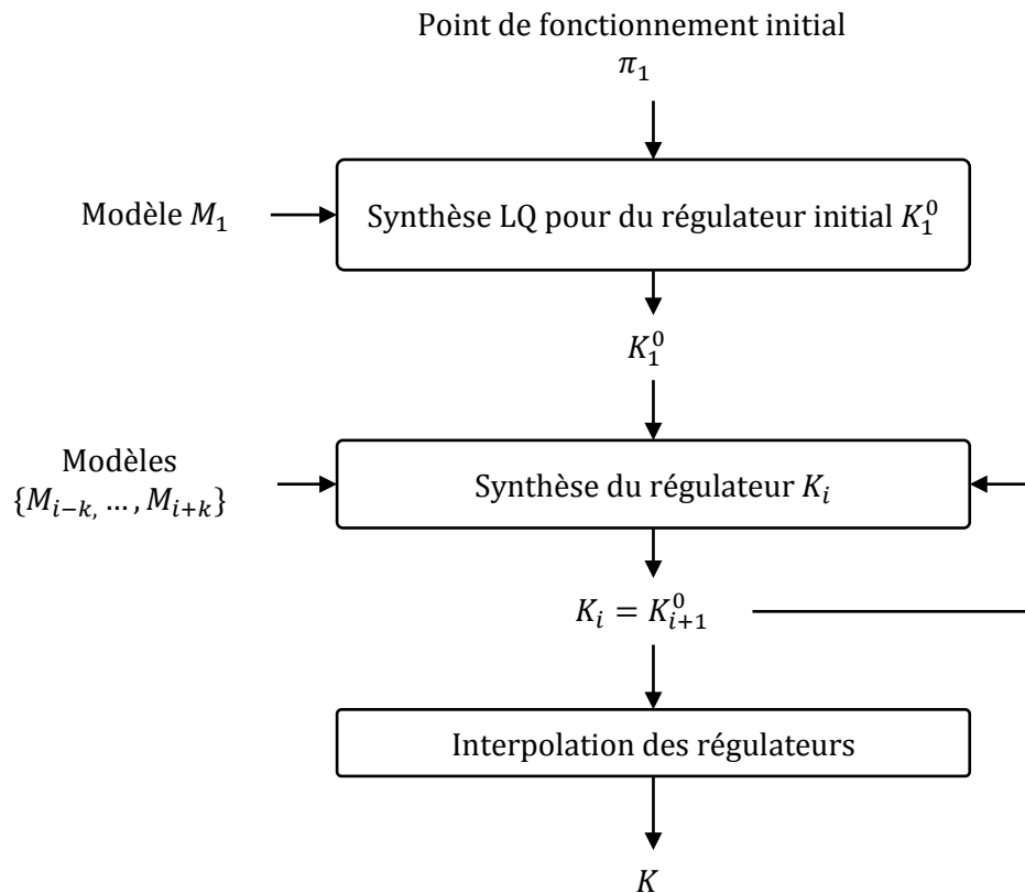
Figure 93: Séquences pour la synthèse LPV
