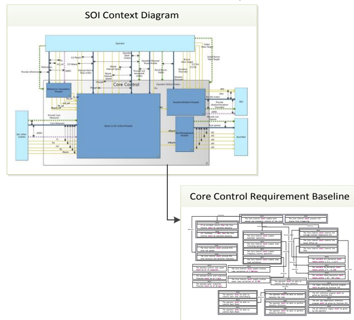
Figure 56: Référentiel d'exigences et SOI
