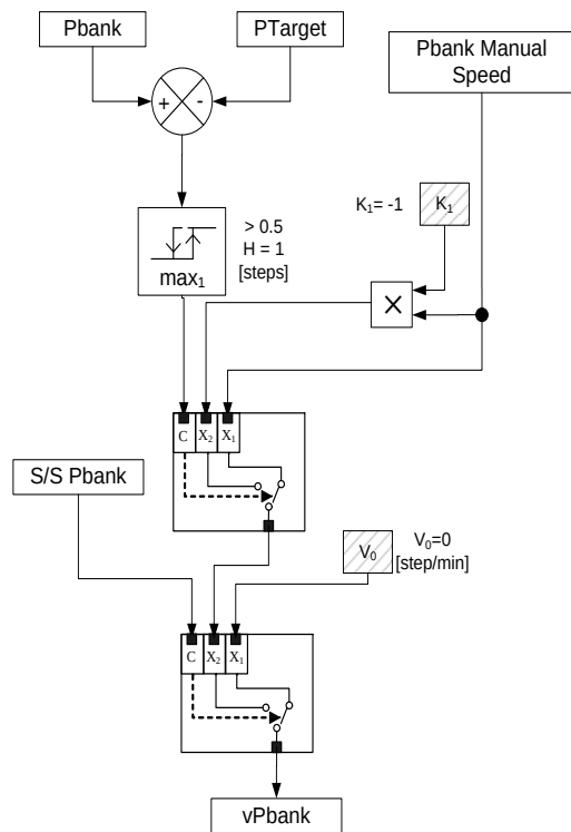
Figure 144 : Diagrammes de Spécification fonctionnelle des fonctions F0002 et F0003
