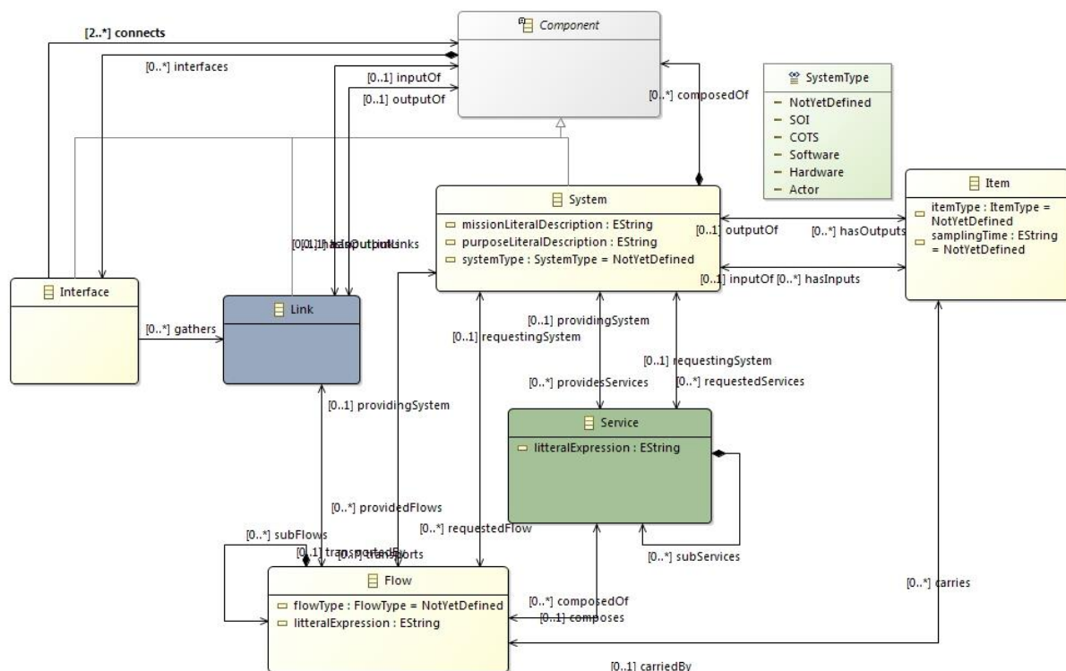
Figure 30: Méta modèle de la vue contextuelle
