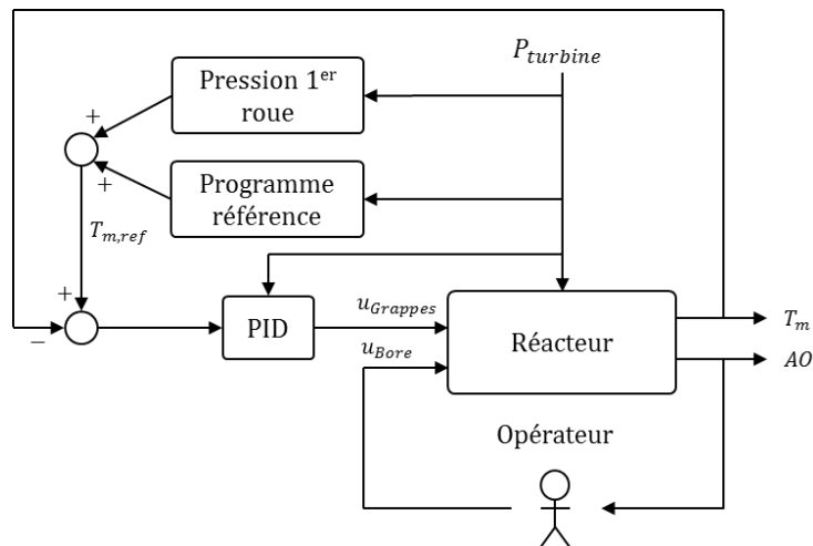
Figure 7: Principe de la régulation du mode A
