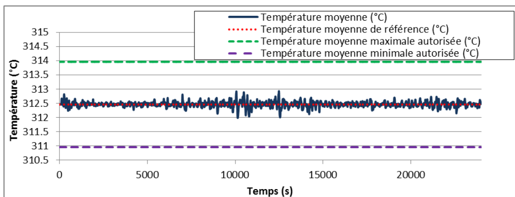
Figure 116: Tracé de la température moyenne - Rampe 100%PN à 70%PN & Réglage de fréquence
