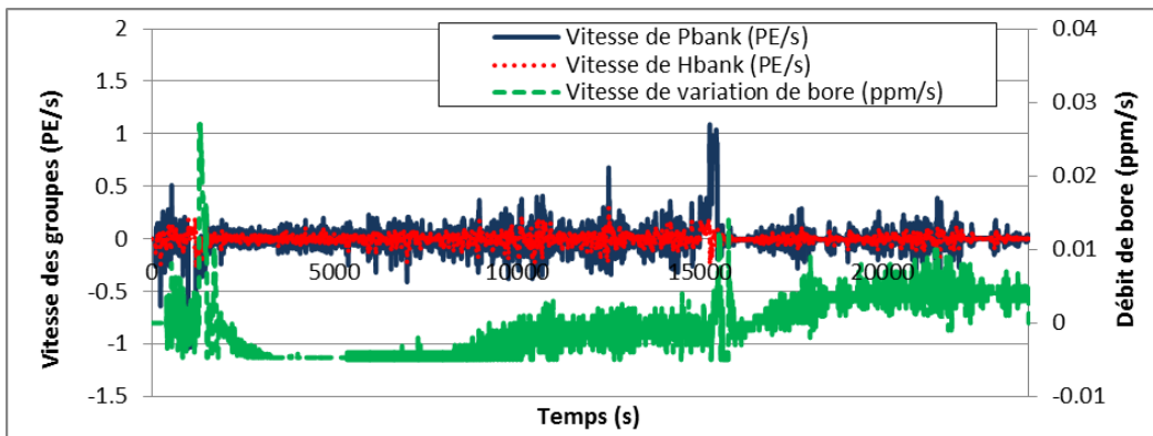
Figure 132: Tracé des vitesses et débit des actionneurs - Rampe de puissance 100%PN à 60%PN à 5%PN/min
