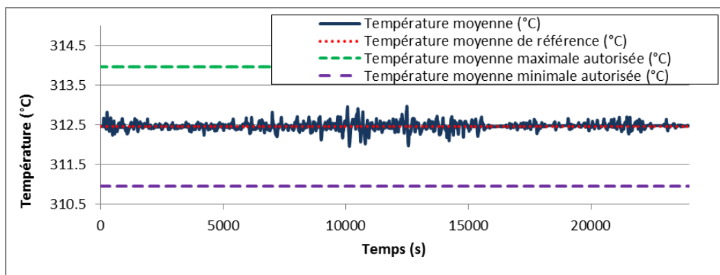
Figure 128: Tracé de la température moyenne - Rampe de puissance 100%PN à 60%PN à 5%PN/min
