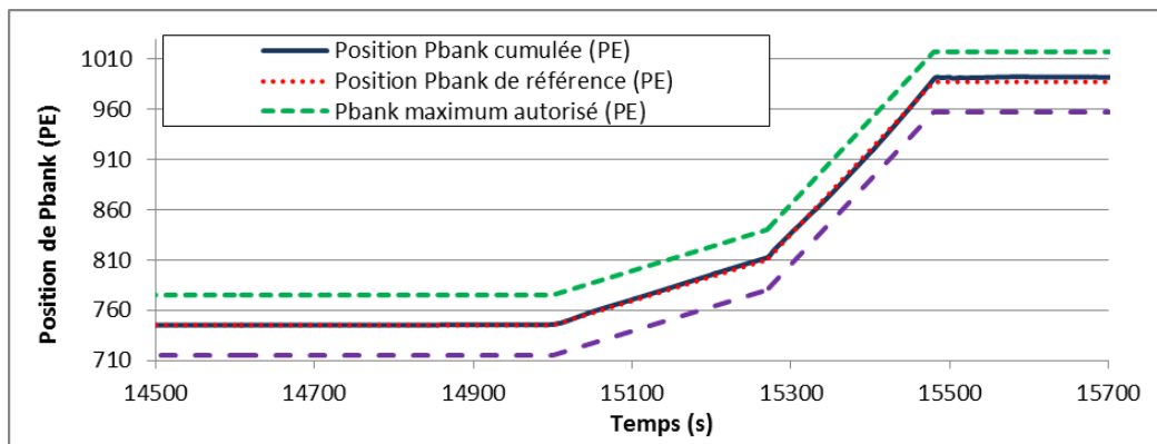
Figure 104: Tracé de la position de Pbank - Rampe de puissance 100%PN à 60%PN – Remontée en charge
