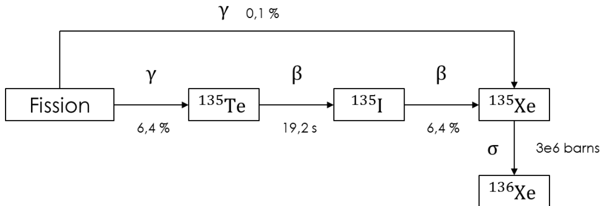
Figure 77: Chaîne de réaction produisant le xénon 135 (les rendements sont relatifs aux fissions de l' ^{235}\text{U} et les durées sont les périodes radioactives)
