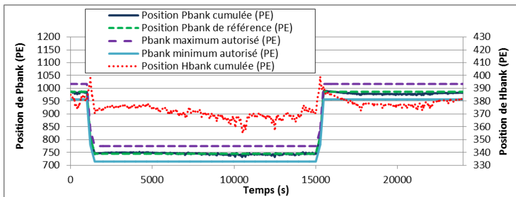
Figure 131: Tracé de la position des groupes - Rampe de puissance 100%PN à 60%PN à 5%PN/min
