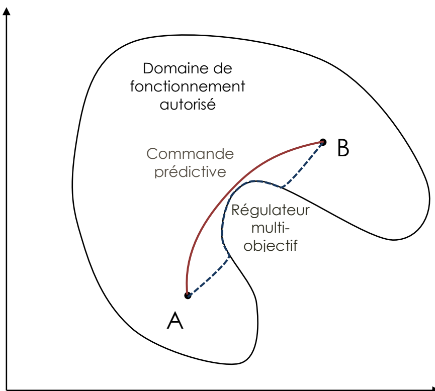
Figure 71: Illustration de la différence de trajectoire régulateur prédictif et multi-objectif
