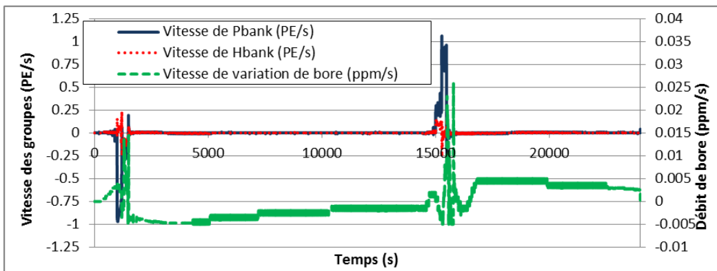
Figure 106: Tracé des vitesses et débit des actionneurs - Rampe de puissance 100%PN à 60%PN
