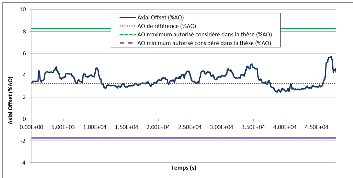
Figure 157: Simulation Mode T – Axial Offset - Réglage de fréquence
