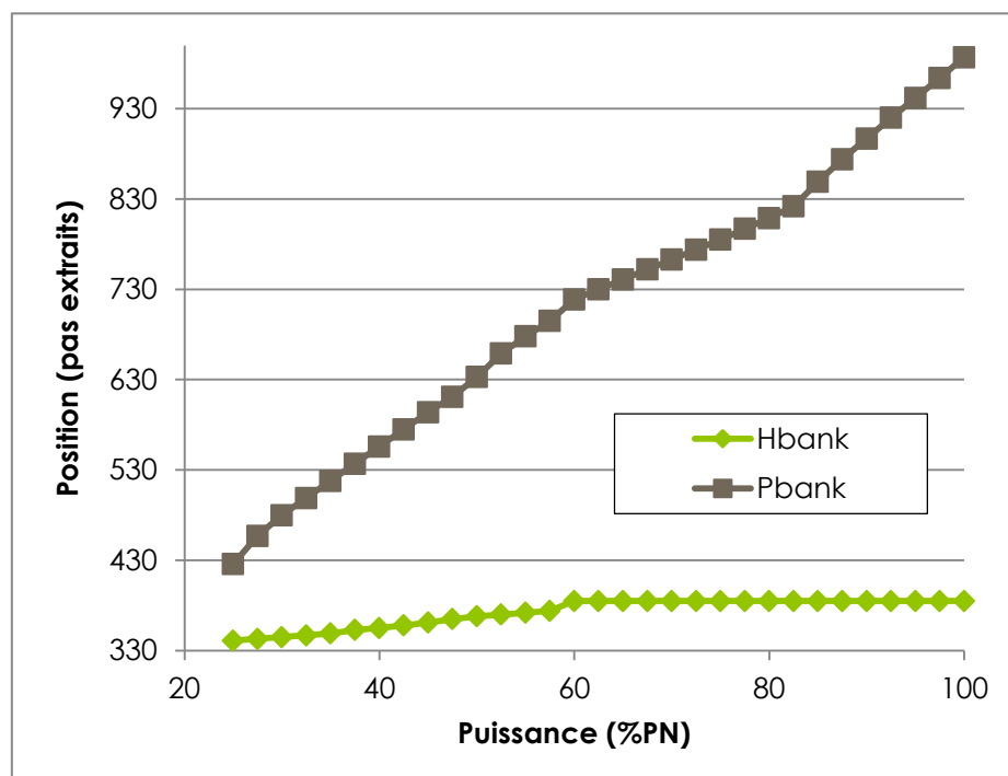
Figure 91: Position de référence des barres Pbank et Hbank pour le séquençage du modèle quasi-LPV
