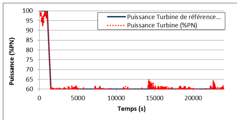
Figure 98: Tracé de la puissance turbine – Rampe de puissance 100%PN à 60%PN et réglage de fréquence
