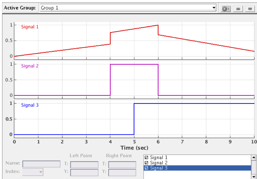
Figure 44: Exemple de diagramme de dépendance (temporel) n°2. Diagramme réalisé avec l'outil Matlab Simulink : Signal Builder
