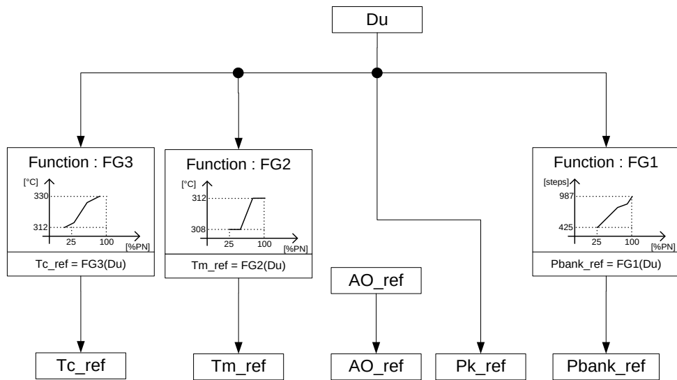
Figure 146: Diagramme de spécification fonctionnelle de la fonction F0020
