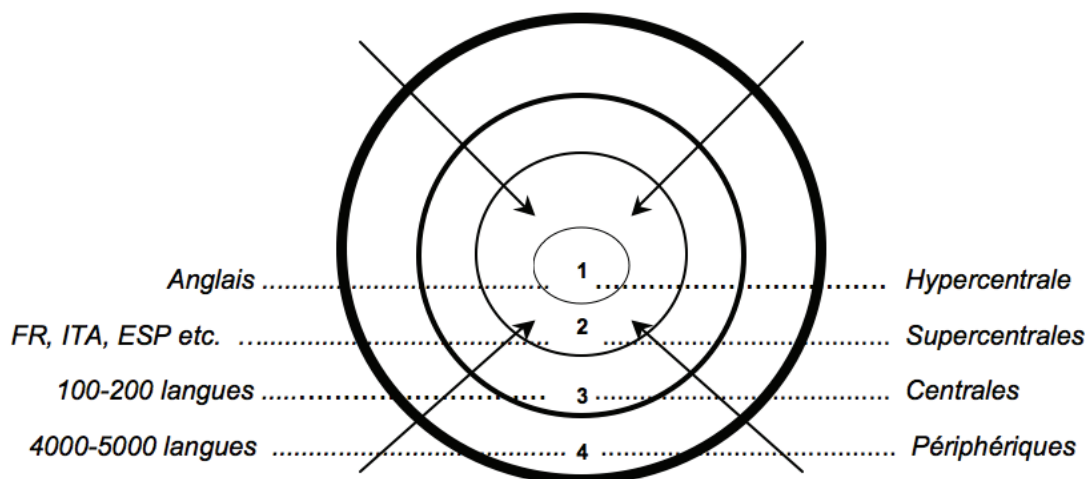
Figure 19: Modèle Gravitationnel
