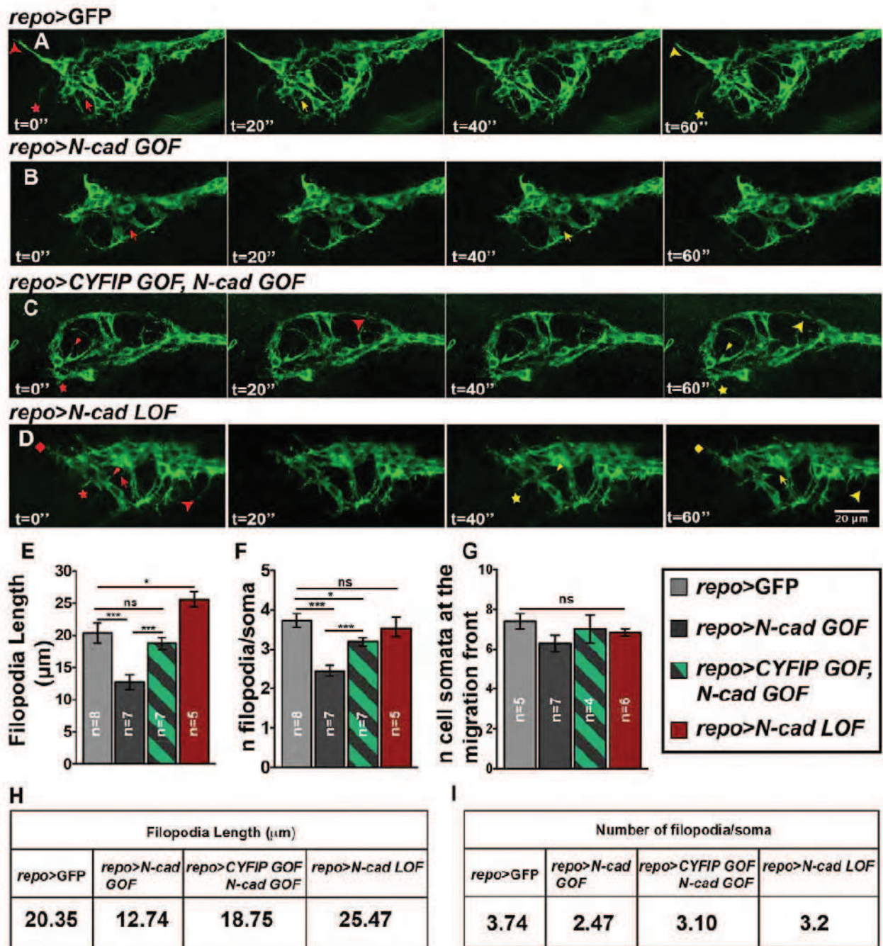
Figure 2: Impact de la N-cad sur la dynamique du cytosquelette d'actine. (A-D)
