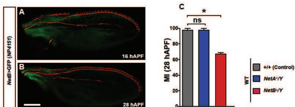
Figure 5: expression et rôle des Netrines. (A,B) Expression de NetB dans des ailes de Drosophile à 16 h et 28 h après formation de la pupa. NetB (GFP, vert) s'accumule en position proximale. Les neurones sont indiqués en rouge (anti-22C10). (C) Indice migratoire des génotypes indiqués. Le graphique représente la quantification sur des ailes de control et mutants NetA Δ , et NetB Δ .
