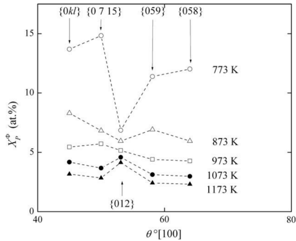
FIGURE 1.12 – Variation de la fraction atomique de phosphore X_P^\phi dans des JG symétriques de flexion d'axe [100] dans un alliage Fe-3.55\%at Si-0.0089\%at P-0.014\%at C en fonction de l'angle de désorientation \theta pour différentes températures [35].
