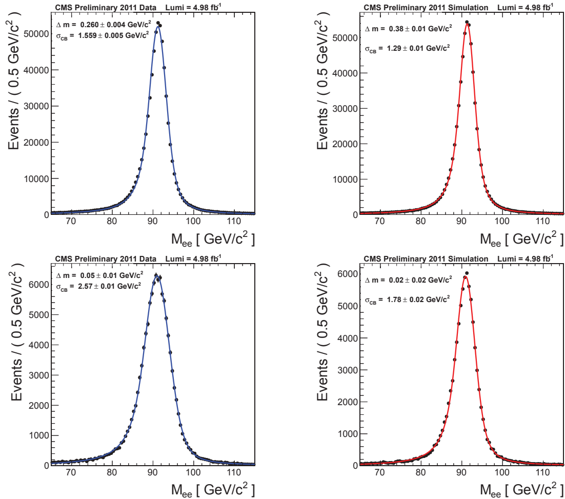
FIGURE 3.22 – Distribution de la masse invariante diélectron pour les événements Z^0 \rightarrow ee sélectionnés ajustée avec une convolution entre une fonction de Crystal-Ball et une fonction de Breit-Wigner, pour le tonneau (haut) et les bouchons (bas), dans les données (gauche) et la simulation (droite). \Delta m est la différence en GeV entre la moyenne de la fonction de Crystal Ball et la masse du boson Z^0 , et \sigma_{CB} est la largeur de la fonction de Crystal-Ball. La moyenne et la largeur de la fonction de Breit-Wigner sont fixées aux paramètres réportés dans [9]. Figure tirée de [68].
