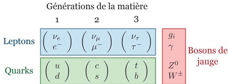
FIGURE 1.1 – Les particules du Modèle Standard. Les fermions (de spin 1/2 ) sont regroupés en trois générations (ou familles), et en deux ensembles : les leptons, soumis aux interactions faible et électromagnétique, et les quarks, soumis aux interactions faible, électromagnétique et forte. Les bosons de jauge (de spin 1) sont les particules agissant comme porteurs des interactions. Les gluons g_i portent l'interaction forte, le photon \gamma porte l'interaction électromagnétique et les bosons W^\pm et Z^0 portent l'interaction faible.
