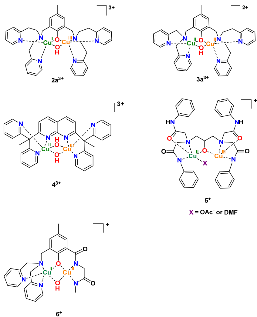
Figure VI.21. Complexes à valence mixte \text{Cu}_2^{\text{III,II}} caractérisés dans ces études.
