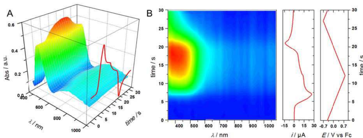
Figure VI.20. A) Représentation 3D du suivi spectroélectrochimique à T = 213 \text{ K} de l'oxydation du complexe 6 dans DMF/ \text{NBu}_4\text{ClO}_4 (0,1 M) (trajet optique 0,2 mm) ; courbe rouge: voltammogramme cyclique en couche mince ( \nu = 0.1 \text{ V/s} ). B) Représentation 2D du spectre différentiel obtenu par rapport au spectre initial pour l'oxydation électrochimique du complexe 6 . Les courbes rouges sur les panneaux de droite représentent la variation de l'intensité du courant ( i ) et du potentiel appliqué ( E ) avec le temps.
