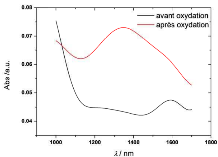
Figure VI.14. Spectre proche-infrarouge ( T = 223 K, trajet optique 0,2 mm) du complexe 4^{2+} dans \text{CH}_3\text{CN}/\text{NBu}_4\text{PF}_6 avant (noir) et après (rouge) oxydation à E = 1,6 V vs Fc.
