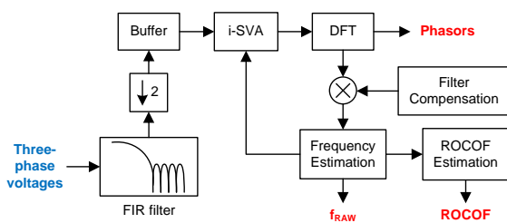
FIGURE E.5 – Méthode i-SVA pour estimer les phaseurs, fréquences et dérivées de fréquence
