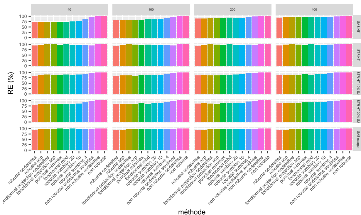
FIGURE 3.10 – Efficacités relatives (RE en %), voir (3.82) ) des différents estimateurs pour les différents plans de sondage en fonction des tailles d'échantillon
