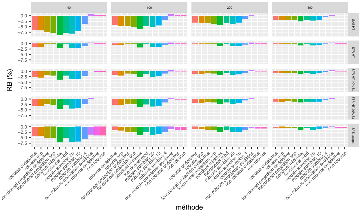
FIGURE 3.8 – Biais relatifs (RB en %), voir (3.80) ) des différents estimateurs pour les différents plans de sondage en fonction des tailles d'échantillon
