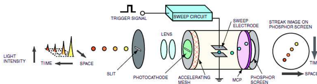
Figure F1. Schéma d'une caméra à balayage de fente. 86 Les photons sont transformés en électrons et sont déviés par un champ électrique vertical généré par un balayage rapide. Selon leur temps d'arrivée, différentes tensions sont appliquées. Ainsi, la fluorescence générée se répand spectralement et temporellement sur les axes horizontaux et verticaux de la caméra CCD, respectivement.
