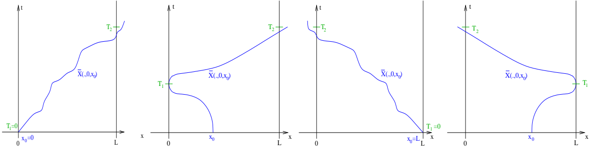
FIGURE 1 : Trajectoires possibles pour t \mapsto \bar{X}(\cdot, 0, x_0) .
