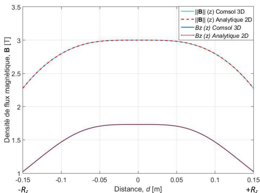
Figure III-25. Valeurs de B_z(z) et \|\mathbf{B}\|(z) obtenues avec R_z = 15 cm et I = 110 A. C3D et parc calcul analytique 2D.
