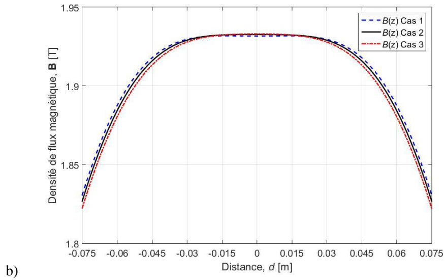
Figure III-3. Densité de flux magnétique produite par différentes sections rectangulaires de bobine de Helmholtz.
