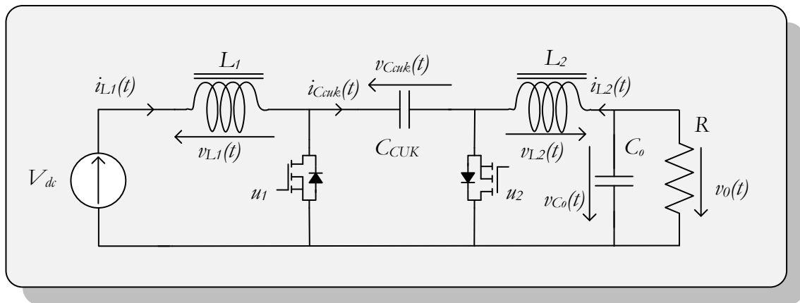
Figure 2-50 Convertisseur CUK
