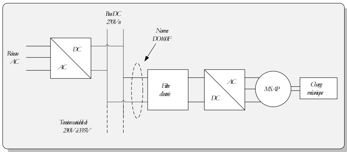
Figure 2-1 - Architecture d'alimentation classique d'une Machine Synchrone à Aimants Permanents
