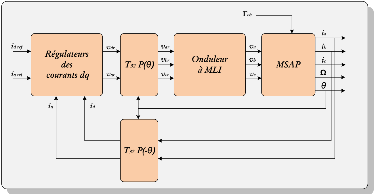
Figure 1-17 Schéma d'une commande vectorielle de MSAP
