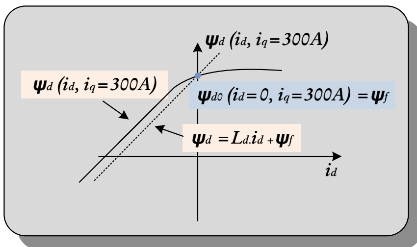
Figure 3-31 Evolution schématique du flux statorique d'axe d pour un courant i_q donné
