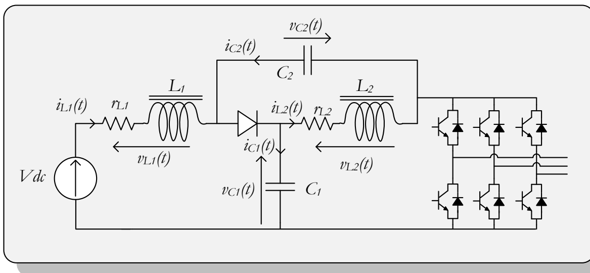
Figure 2-12 - Onduleur à Quasi Z-source avec couplage des inductances
