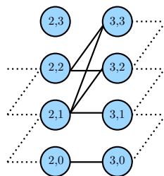
FIGURE 8.3: Représentation d'une colonne d'un diagramme sans trou.
