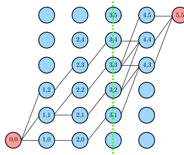
FIGURE 3.11: Diagramme K = 5 , M = 5 et \mathbf{C} = (2, 2, 1, 2, 2) vérifiant la propriété d'arbre \mathcal{T}_3 .
