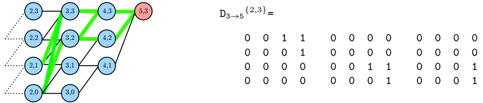
FIGURE 8.5: Matrice D_{3 \rightarrow 5}^{\{2,3\}} correspondant aux arcs en gras et vert.
