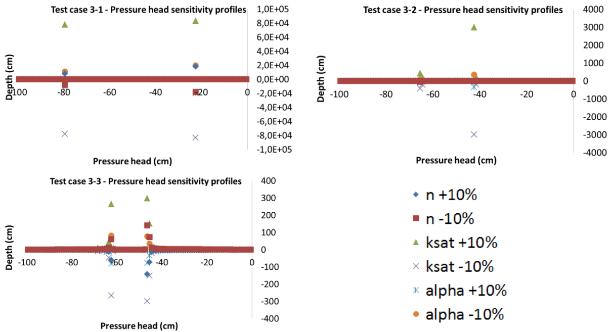
FIGURE 111 : ANALYSE DE LA SENSIBILITE DE LA PRESSION EN EAU A UNE VARIATION DE \pm 10\% DE KS ( \partial H/(\partial K_S) ), ALPHA ( \partial H/\partial \alpha ) ET N ( \partial H/\partial N ) LE LONG DU DOMAINE POUR LES CAS 3-1 A 3-3)
