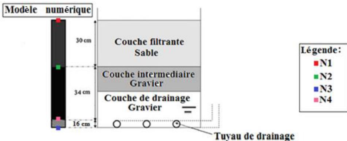
FIGURE 67: DISCRETISATION SPATIALE DU FPR EN 1D
