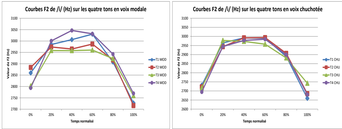
Figure 92 : Courbes F2 (Hz) de /i/ sur les quatre tons, définies à partir des moyennes interindividuelles de F2 : voix modale (à gauche) vs voix chuchotée (à droite).
