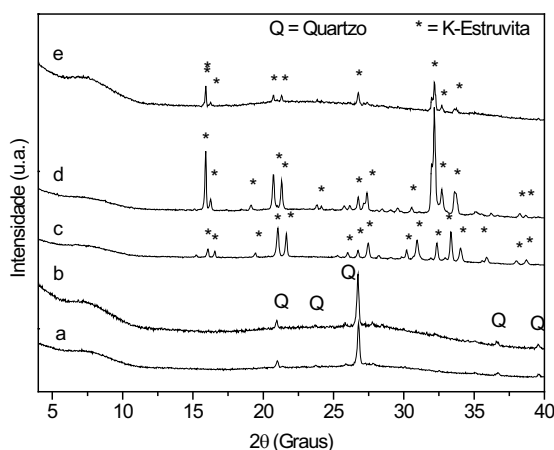
Figura 29- Difractogramas de raios X dos resíduos sólidos resultantes das amostras: MMT/K 2 HPO 4 após 30 min (a), MMT/K 2 HPO 4 após 31 dias (b), Talco/K 2 HPO 4 após 30 min (c), Talco/K 2 HPO 4 após 7 dias (d) e Talco/K 2 HPO 4 após 31 dias (e).
