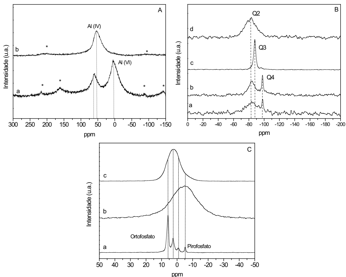
Figura 25- Espectros de ^{27}\text{Al} RMN MAS da MMT (Aa) e MMT/ \text{K}_2\text{HPO}_4 moídos (Ab); (B) ^{29}\text{Si} RMN MAS para a MMT (Ba), MMT/ \text{K}_2\text{HPO}_4 moído (Bb), talco (Bc) e talco/ \text{K}_2\text{HPO}_4 moído (Bd); (C) ^{31}\text{P} RMN MAS para o \text{K}_2\text{HPO}_4 (Ca), MMT/ \text{K}_2\text{HPO}_4 moído (Cb) e talco/ \text{K}_2\text{HPO}_4 moído (Cc).
