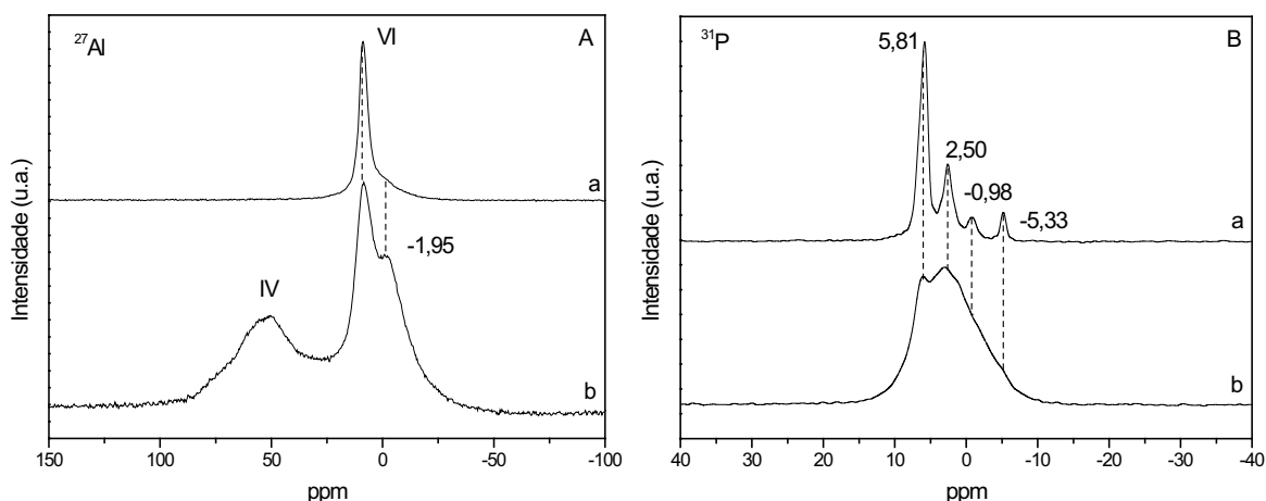
Figura 51- Espectros de RMN do ^{27}\text{Al} nas amostras MgAl (Aa), MgAl - calcinado/ \text{K}_2\text{HPO}_4 (Ab) e espectros de RMN do ^{31}\text{P} nas amostras \text{K}_2\text{HPO}_4 (Ba), MgAl - calcinado/ \text{K}_2\text{HPO}_4 (Bb).
