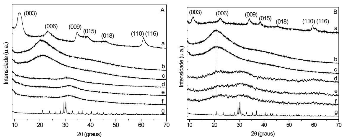
Figura 62- Difratogramas de raios x dos materiais resultantes dos experimentos envolvendo CMC.
