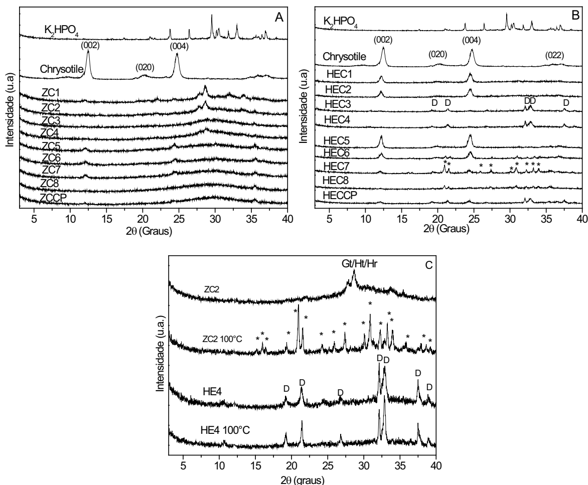
Figura 36- Difratomogramas de raios X dos materiais resultantes do sistema crisotila/ K_2HPO_4 , moídos no moinho Z (A), moinho HE (B) e ZC2 ou HEC4 tratados a 100 °C (C). * - K estruvita; Gt - Goetita; Ht - Hematita; Hr - Hornblenda; D - Dittmarita.
