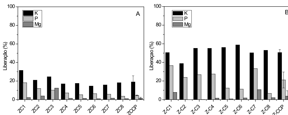
Figura 40- Liberação de nutrientes após 1 h (A) e 168 h (B) dos materiais resultantes do sistema crisotila/ \text{K}_2\text{HPO}_4 , moídos no moinho Z.
