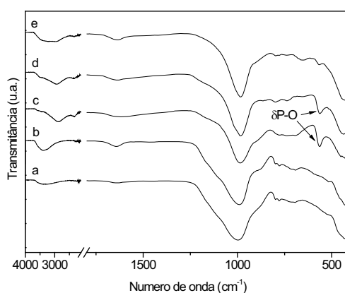
Figura 30- Espectros de FTIR dos resíduos sólidos resultantes das amostras: da MMT/ K_2HPO_4 após 30 min (a), MMT/ K_2HPO_4 após 31 dias (b), Talco/ K_2HPO_4 após 30 min (c), Talco/ K_2HPO_4 após 7 dias (d) e Talco/ K_2HPO_4 após 31 dias (e).
