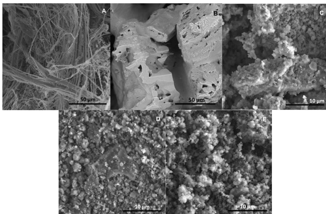
Figura 37- Imagens de MEV dos materiais: crisotila (A), K_2HPO_4 (B), ZC1 (C), ZC2 (D) e ZC3 (E).
