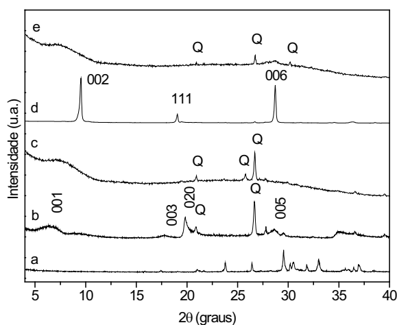
Figura 22- Difratomogramas de raios X do K 2 HPO 4 (a), MMT (b), MMT/K 2 HPO 4 moído (c), talco (d), talco/K 2 HPO 4 moído (e).
