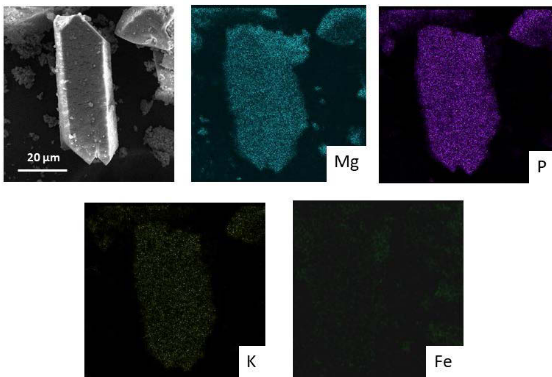
Figura 59- Mapas de EDS do resíduo MgFe - calcinado/ K_2HPO_4 após 30 minutos.
