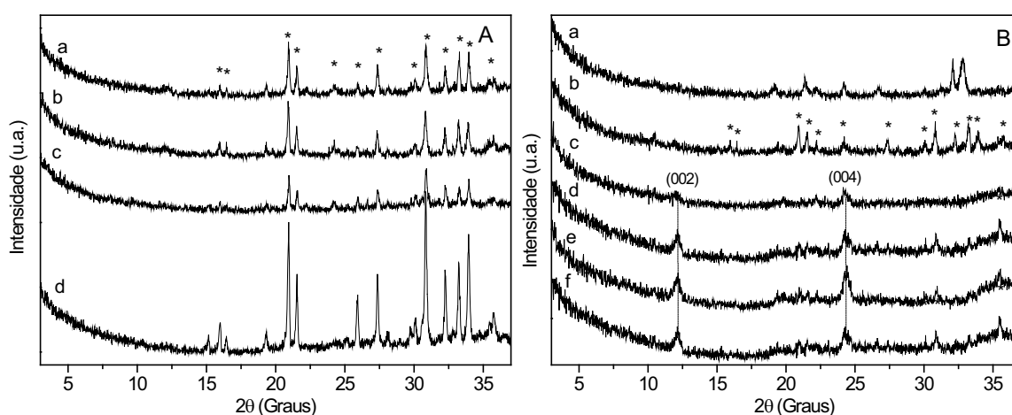
Figura 42- Difratogramas de raios X dos resíduos sólidos dos materiais resultantes do sistema crisotila/ K_2HPO_4 , moídos no moinho Z (A) após liberação: ZC1 1 h (Aa) e 168 h (Ab); ZC2 1 h (Ac) e 168 h (Ad); moinho HE (B) após liberação: HEC4 1h (Ba) e 168h (Bc), HEC7 1h (Bc) e 168h (Bd); HEC8 1 h ( Be) e 168 h ( Bf). Estruvita de potássio indicada por (*).
