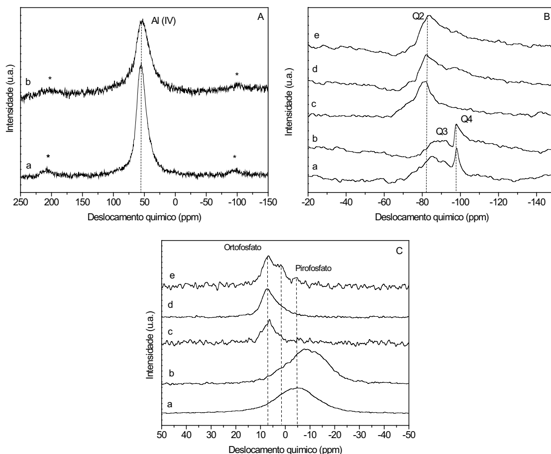
Figura 31- Espectros de RMN MAS dos resíduos sólidos derivados das amostras: ^{27}Al MMT/ K_2HPO_4 após 30 min (Aa) e após 31 dias (Ab); ^{29}Si MMT/ K_2HPO_4 após 30 min (Ba) e após 31 dias (Bb), Talco/ K_2HPO_4 após 30 min (Bc), após 7 dias (Bd) e após 31 dias (Be). ^{31}P MMT/ K_2HPO_4 após 30 min (Ca) após 31 dias (Cb), Talco/ K_2HPO_4 após 30 min (Cc), após 7 dias (Cd) e após 31 dias (Ce).
