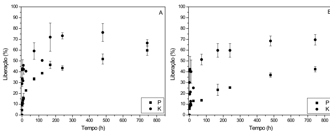
Figura 28- Curvas de liberação de P e K para os sistemas: MMT/ K_2HPO_4 (A) e talco/ K_2HPO_4 (B).
