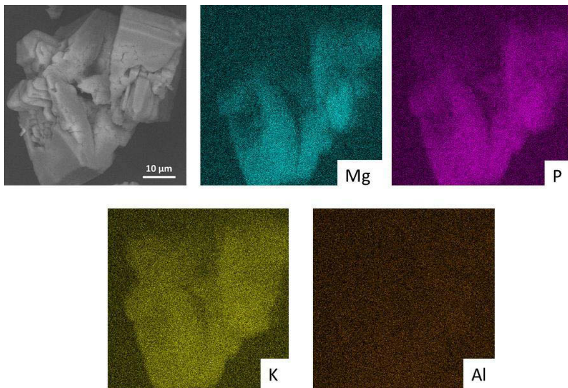
Figura 58- Mapas de EDS do resíduo MgAl - calcinado/ K_2HPO_4 após 30 minutos.
