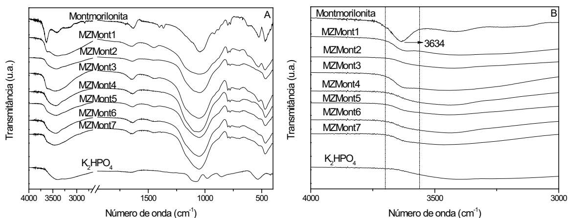
Figura 16- Espectros de FTIR dos materiais resultantes do planejamento fatorial 2 2 envolvendo MMT e K 2 HPO 4 .
