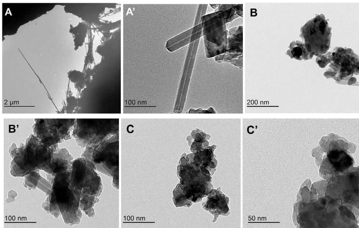
Figura 47- Imagens de MET para: telha sem tratamento (A,A'); telha moída por 4 min (B,B'); telha moída por 16 min (C,C').
