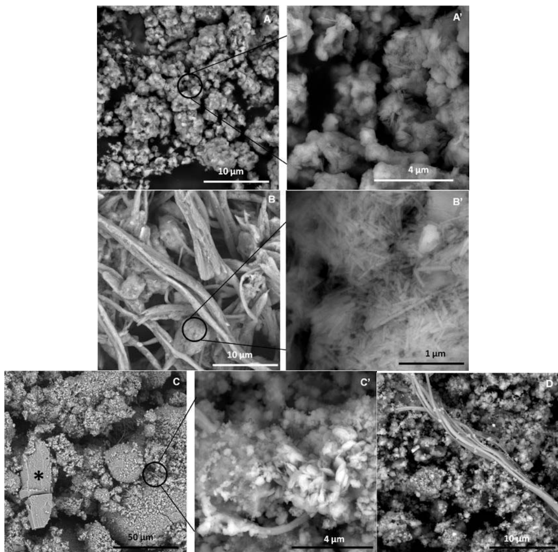
Figura 38- Imagens de MEV das amostras HEC4 (A,A'), HEC6 (B,B'), HEC7 (C,C') e HEC8 (D), respectivamente. Estruvita potássica indicada por um *.
