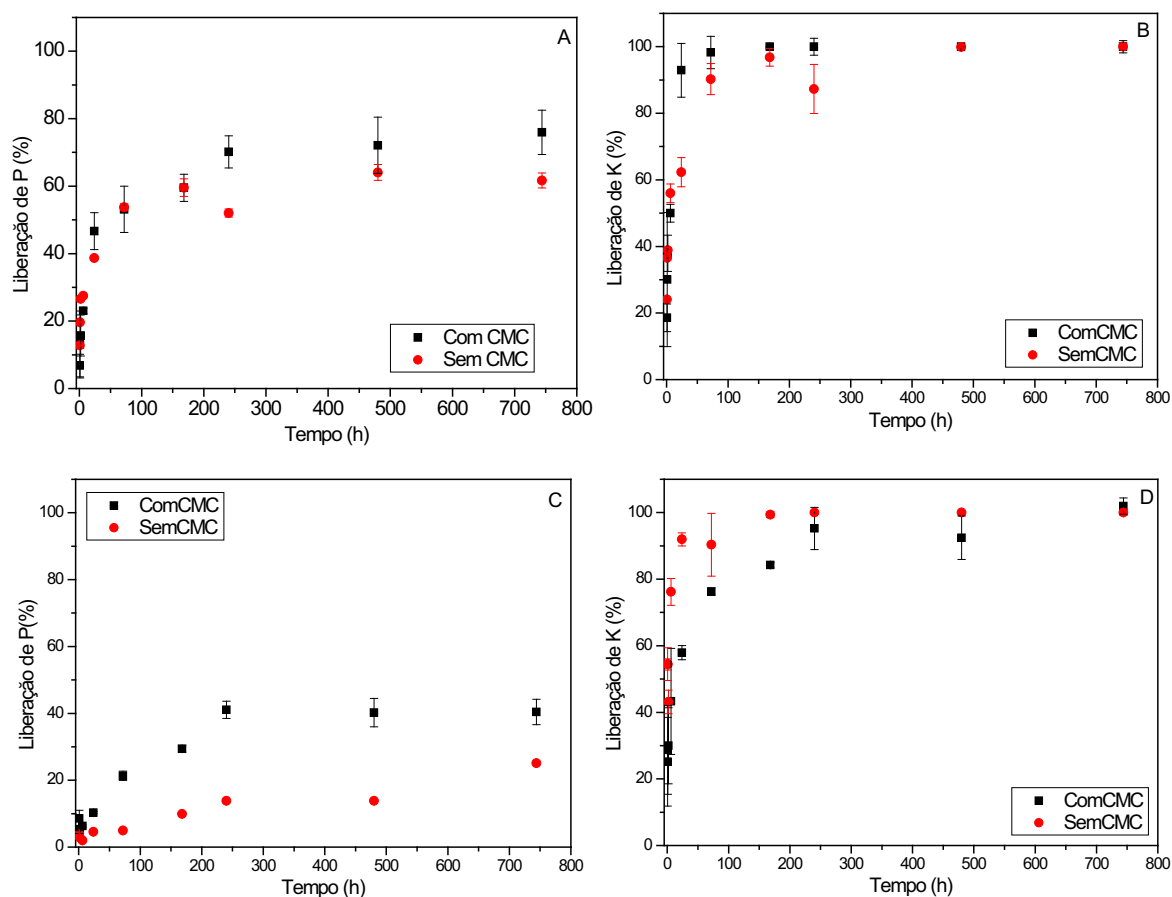
Figura 64 – Curvas de liberação para P e K da amostra HFC2 (a,b) e da amostra HFC4 (c,d).
