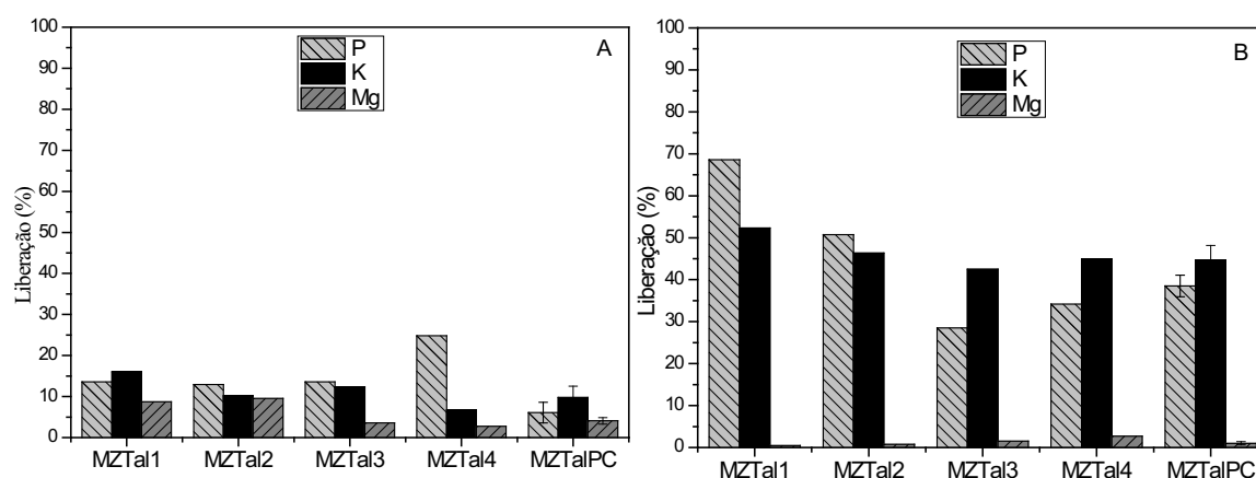
Figura 19- Ensaios de liberação dos materiais resultantes do sistema talco/K 2 HPO 4 em 1 hora (A) e 168 horas (B).
