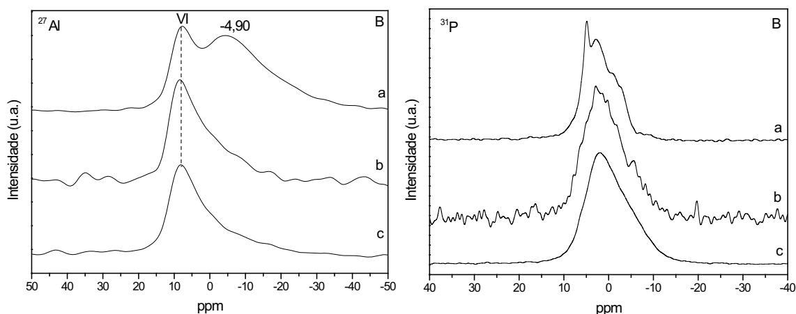
Figura 60- Espectros de RMN de ^{27}\text{Al} dos resíduos sólidos resultantes dos sistemas MgAl - calcinado/ \text{K}_2\text{HPO}_4 após 30 min (Aa), 7 dias (Ab) e após 31 dias (Ac) e espectros de RMN de ^{31}\text{P} dos sistemas MgAl - calcinado/ \text{K}_2\text{HPO}_4 após 30 min (Ba), 7 dias (Bb) e após 31 dias (Bc).
