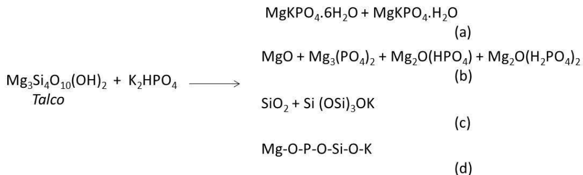
Figura 35-Possíveis produtos gerados na ativação mecanoquímica do sistema Talco /K 2 HPO 4 .
