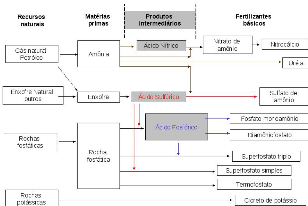
Figura 2- ilustração de produção de alguns fertilizantes (adaptado de: http://www.ebah.com.br/content/ABAAAA3-AAH/aula-fertilizantes ).
