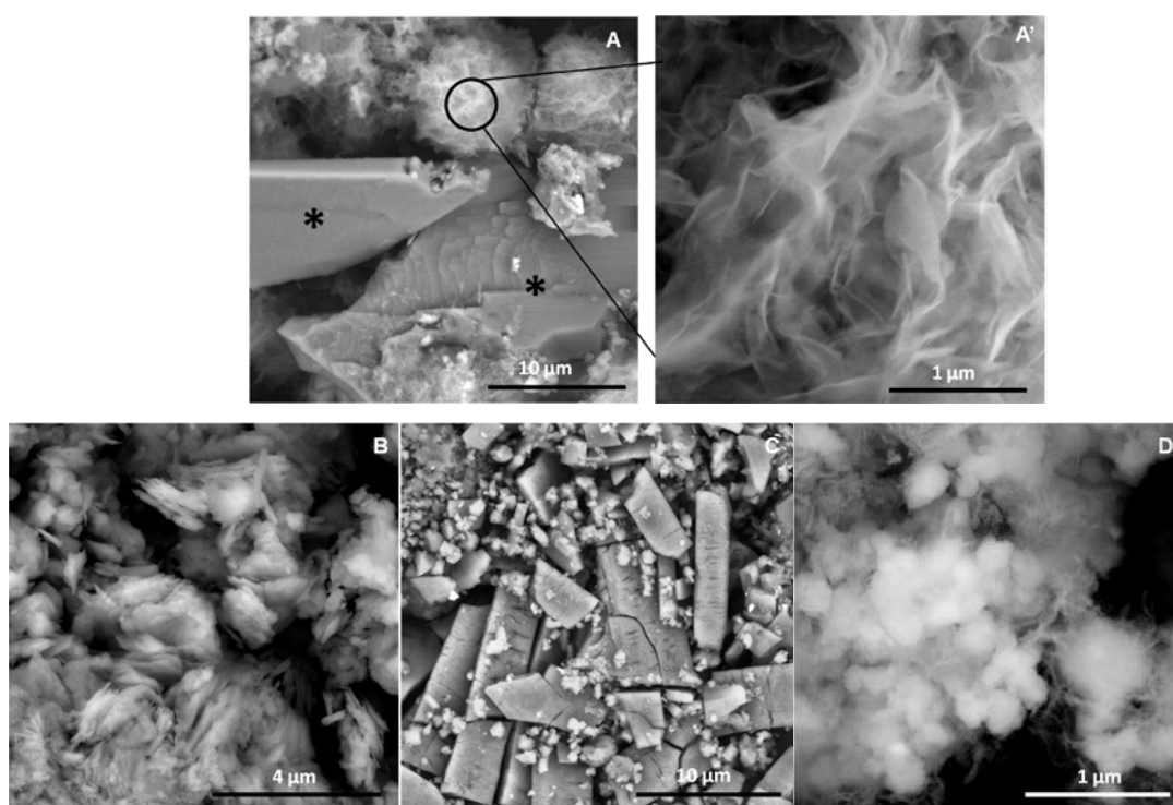
Figure 43- Imagens de MEV dos resíduos sólidos das amostras derivadas do sistema crisotila/ K_2HPO_4 : ZC2 após 168 h de liberação (A, A'), HEC4 após 1 h (B) e depois de 168 h de liberação (C) e HEC8 após 168 h de liberação (D). Estruvita de potássio indicada por (*).
