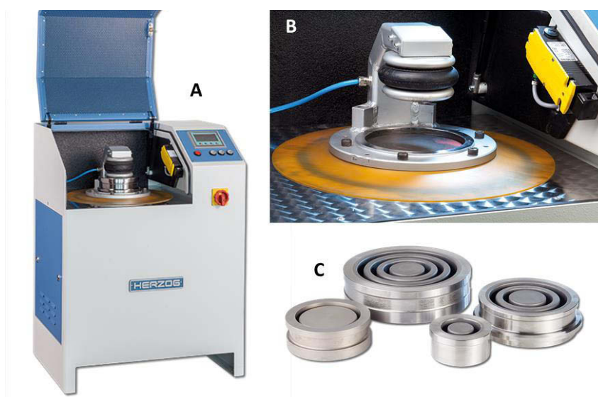
Figura 12- Fotografia do moinho Herzog: visão geral do equipamento (A), câmara interna do moinho (B) e vasos compatíveis com o moinho (C). adaptado de: http://www.herzog-maschinenfabrik.de/us/produkte/muehlen/hsm-100-hsm-250/ .
