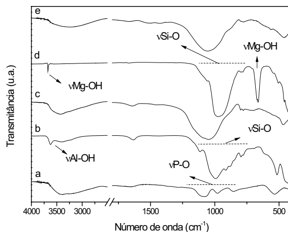
Figura 24- Espectros de FTIR do \text{K}_2\text{HPO}_4 (a), MMT (b), MMT/ \text{K}_2\text{HPO}_4 moído (c), talco (d), talco/ \text{K}_2\text{HPO}_4 moído (e).
