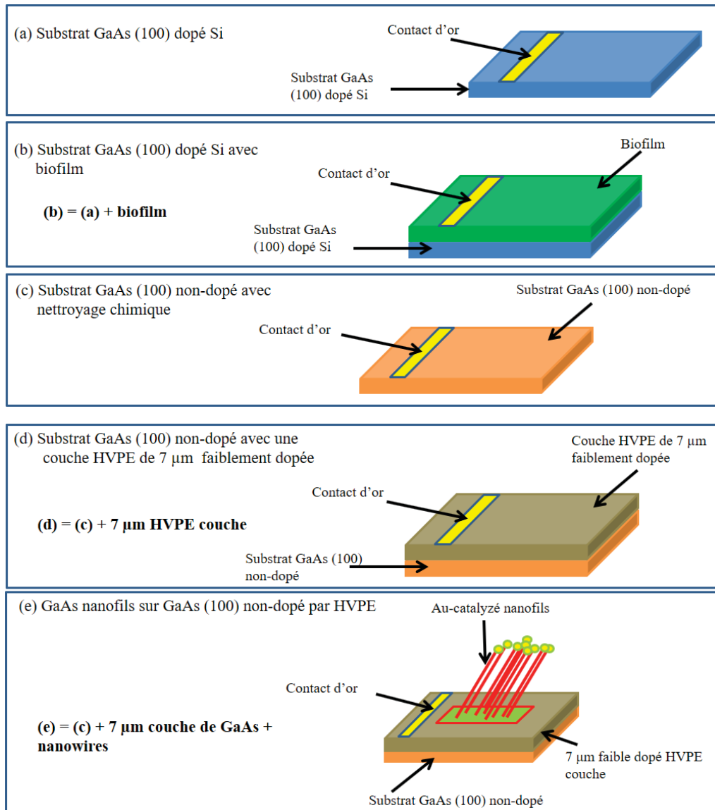
Figure. 8: Résumé des cinq électrodes GaAs testées pour leur compatibilité électrochimique.
