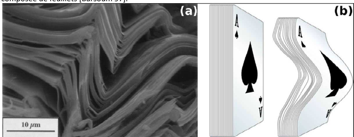
Figure I.16 : Structure nanolamellaire de \text{Ti}_3\text{SiC}_2 : (a) Déformation des lamelles en kink-band observée sur une face fracturée [Bar99b] ; (b) Analogie avec un jeu de carte déformé par une sollicitation parallèle aux plans des cartes [Barsoum 97]
