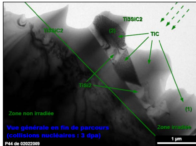
Figure I.19 : Zone proche de la fin de parcours dans \text{Ti}_3\text{SiC}_2 irradié au Xe 92 MeV, 1.10^{15} \text{ cm}^{-2}
