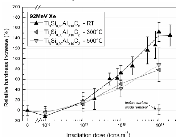
Figure I.23 : durcissement relatif de \text{Ti}_3\text{SiC}_2 irradié aux ions Xe de 92 MeV, pour différente température, en fonction de la fluence.
