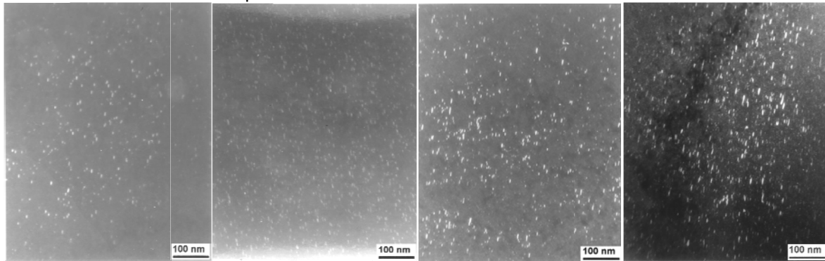
Figure I.10: Visualisation des fautes d'empilement dans les boucles de Frank pour les échantillons irradiés à a) 1.3 dpa, b) 2.4 dpa, c) 3.2 dpa et d) > 7 dpa
