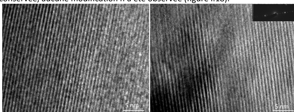
Figure I.18 : Image haute résolution montrant la surstructure selon l'axe c dans l'échantillon non irradié (à gauche) et irradié à 4.5.10^{13} \text{ cm}^{-2} , Xe 930 MeV.
