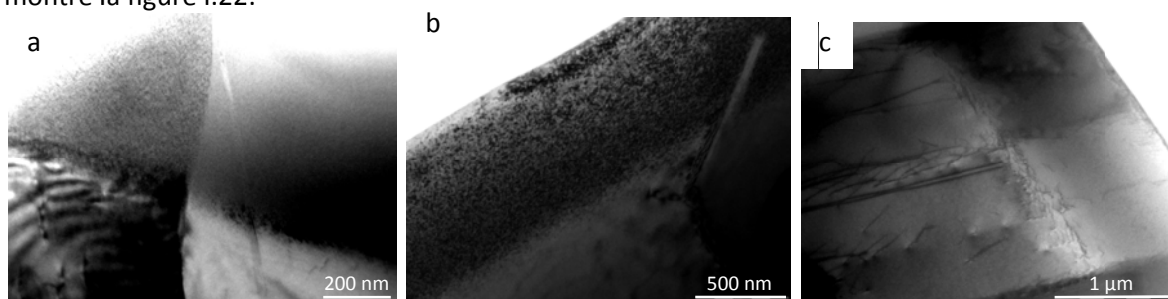
Figure I.22: evolution de la population de défauts étendus en fonction de la température a) 20°C b) 500°C et c) 900°C lors d'irradiation avec des ions Au 4 MeV à une fluence de 10^{15} / \text{cm}^2
