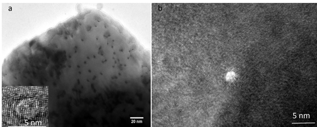
Figure II.11 : observation des traces latentes dans \text{SrTiO}_3 irradié à 10^{11} \text{ Xe } 92\text{MeV/cm}^2 a) sur poudre b) sur monocristal
