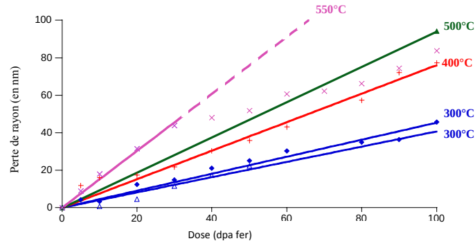
Figure II.1 : Evolution de la perte de rayon en fonction de la dose dans l'EM10+MgO irradié aux électrons de 1 MeV, pour différentes températures.
