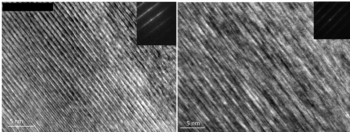
Figure I.20 : \text{Ti}_3\text{SiC}_2 a) zone non irradiée b) zone irradiée proche de la surface (<1 dpa) Xe 92 MeV 1.10^{15} \text{ cm}^{-2}
