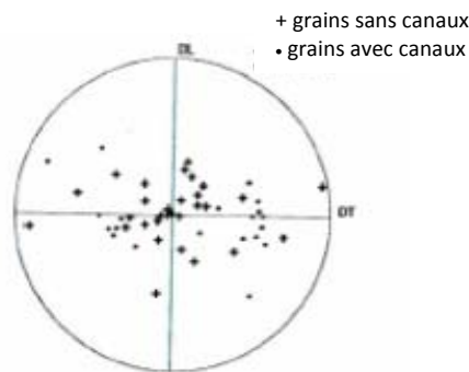
Figure I.5: figure de pôle des grains observés sur l'éprouvette A
