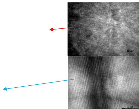
Figure I.21 : \text{Ti}_3\text{SiC}_2 irradié avec Au 4 MeV jusque 7 dpa. Le grain de gauche est orienté selon l'axe a et le grain de droite selon l'axe c. Pour le grain orienté selon a, il n'y a pas de modification de la diffraction, de nombreux défauts d'irradiation sous visibles. Pour le grain orienté selon c, les clichés de diffraction montrent la perte de la surstructure selon cet axe, ce qui est confirmé par les images en haute résolution
