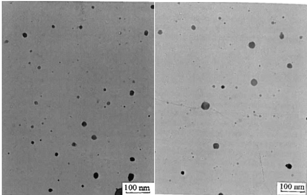
Figure II.4 Répartition des oxydes sur les répliques extractives, dans l'EM10+ \text{MgAl}_2\text{O}_4 , avant irradiation (à gauche) et après irradiation à 500°C jusque 46 dpa avec des ions krypton de 1,2 MeV (à droite).
