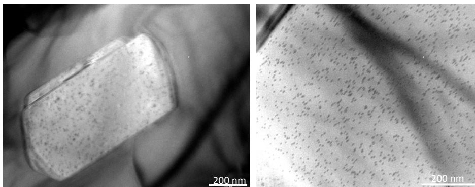
Figure I.17 : Traces latentes dans un silicure irradié aux ions Xe de 92 MeV, 2.10^{11} \text{ cm}^{-2} . On peut noter que le grain de \text{Ti}_3\text{SiC}_2 autour du silicure ne contient aucune trace.
