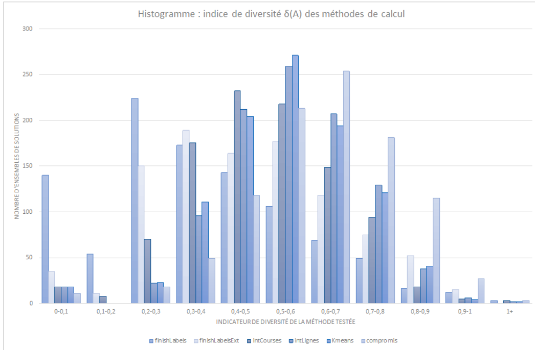
FIGURE 37 – Histogramme : \delta diversité des ensembles de résultat
