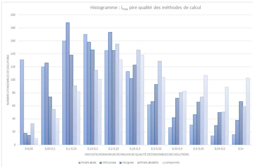
FIGURE 36 – Histogramme : i_{max} pire qualité des ensembles de résultat
