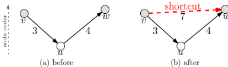
FIGURE 15 – Contraction du nœud u ([Geis2008])
