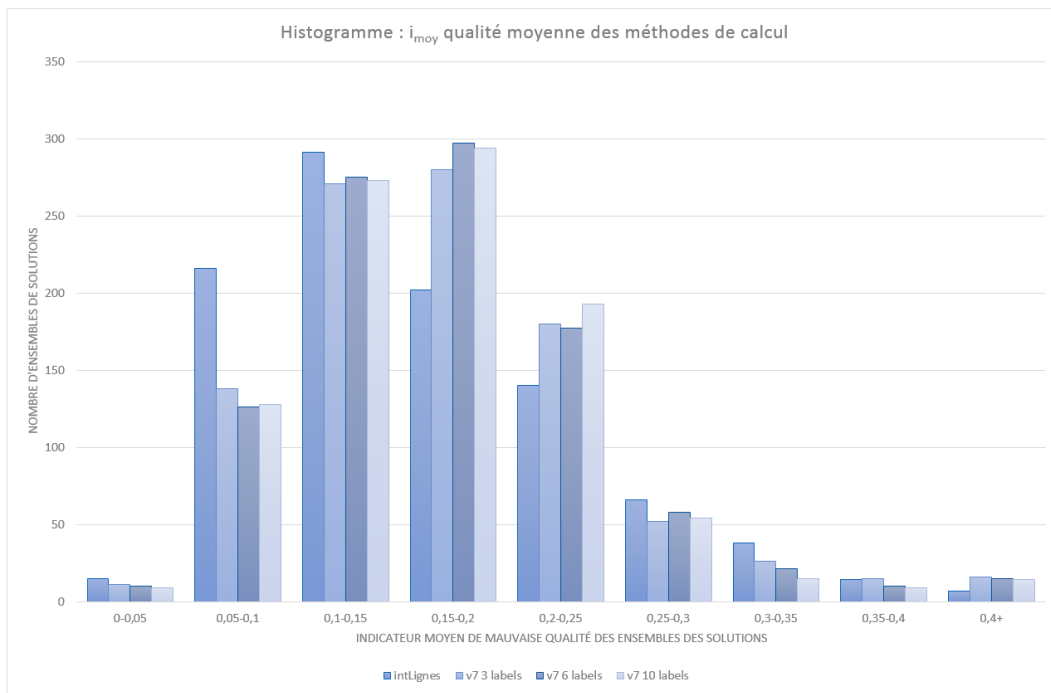
FIGURE 39 – Histogramme : i_{moy} qualité moyenne des ensembles multilabels
