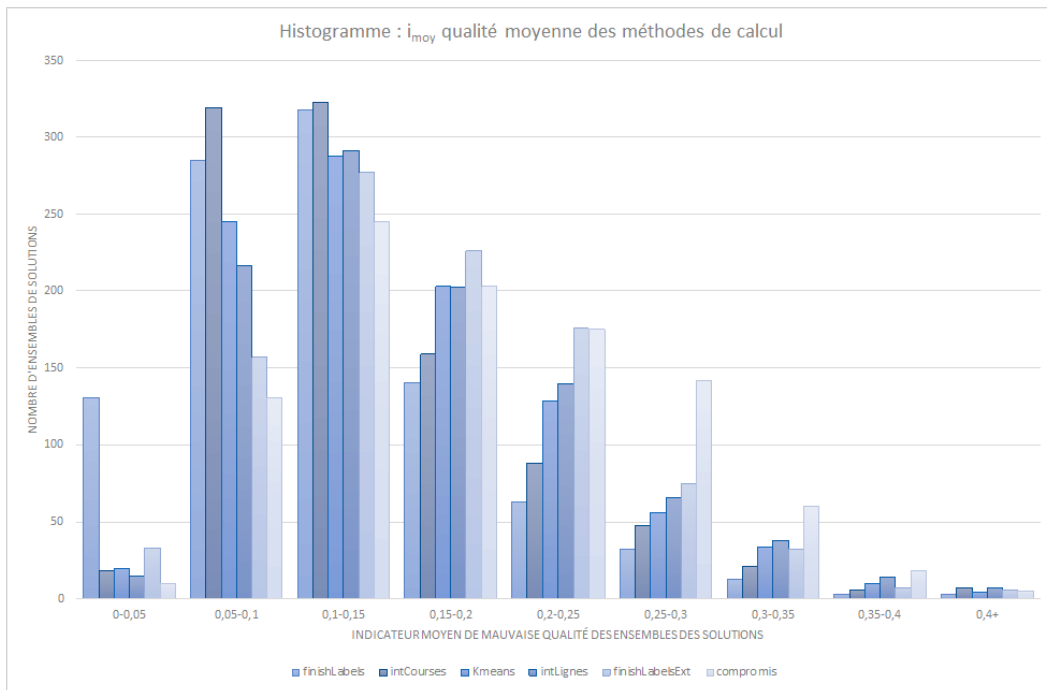
FIGURE 35 – Histogramme : i_{moy} qualité moyenne des ensembles de résultat
