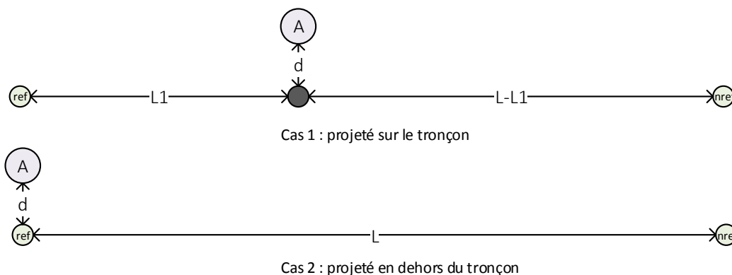
FIGURE 43 – Modélisation naturelle
