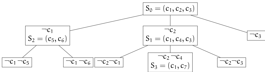
FIGURE 29 – Exemple d'arbre de recherche généré par l'algorithme 5
