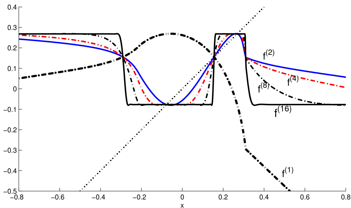
FIG. 7: Figure identique à la figure 6, avec en outre les itérées d'ordre 8 et 16. La convergence vers le régime à deux états est très rapide, quelle que soit la condition initiale (abscisse x ).
