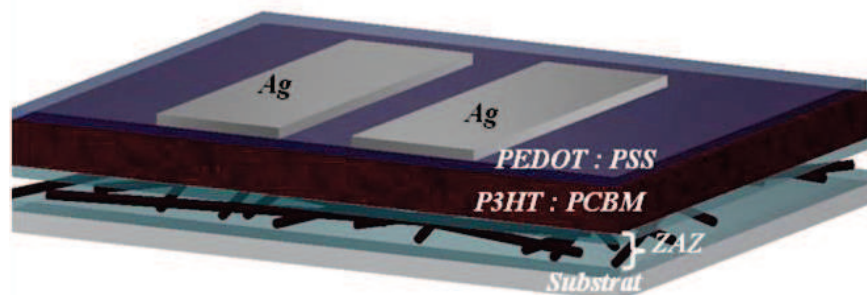
Figure III. 2 : Architecture de la cellule solaire organique à base de l'électrode ZAZ.
