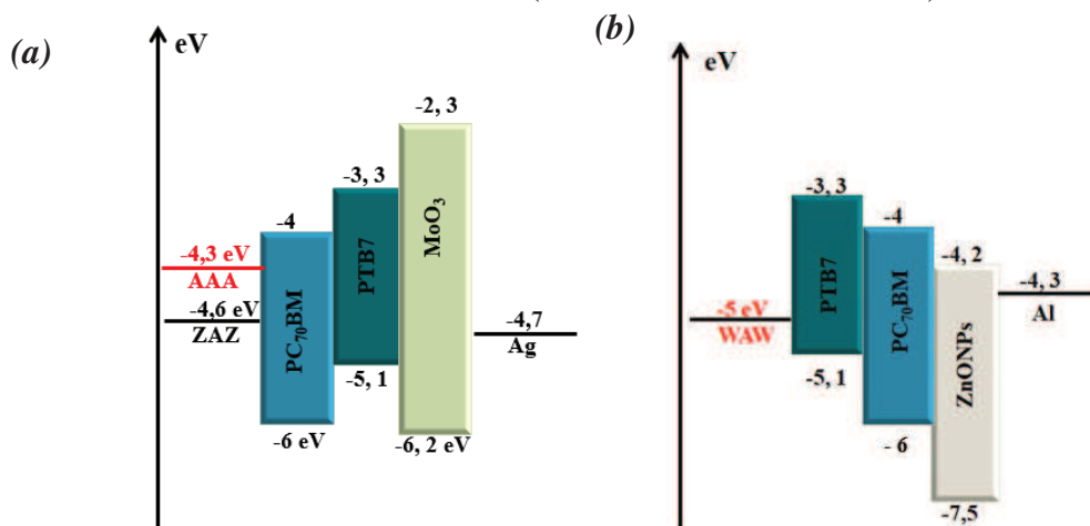
Figure II. 39 : Diagramme d'énergie pour une cellule OPV à base du PTB7:PC 70 BM utilisant les trois électrodes tricouches comme (a) cathode dans une structure inversée, (b) anode dans une conventionnelle.
