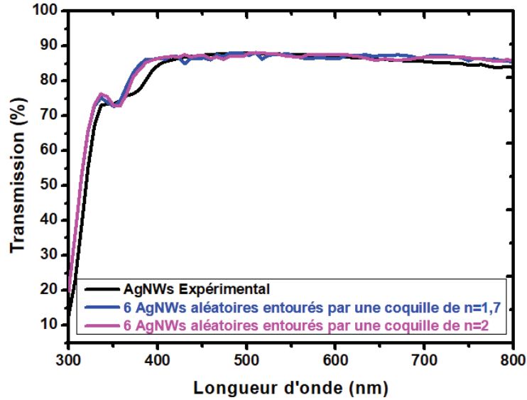
Figure IV. 34 : Comparaison entre les transmissions des AgNWs mesurée expérimentalement et 6 AgNWs semi-aléatoires entourés par des coquilles dont l'indice optique est entre 1,7 et 2.
