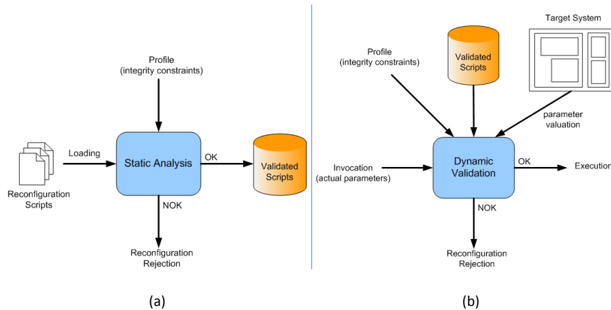
FIGURE 5.3 – Prévention des fautes : (a) Analyse statique (b) Validation dynamique
