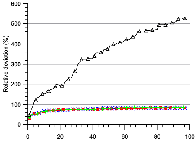
a. (m=3,n=10,d=3)
