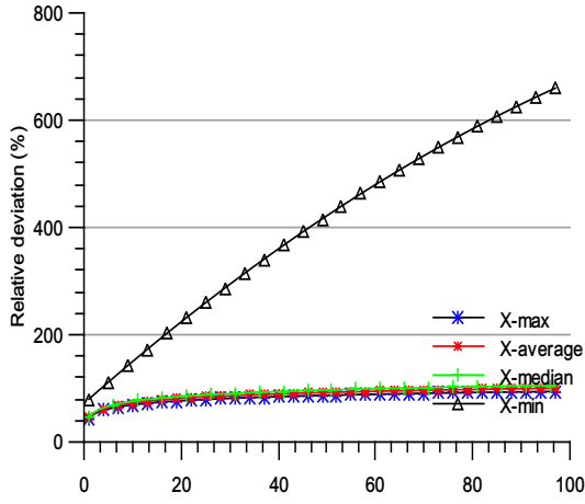
a. (m=3,n=10,d=3)
