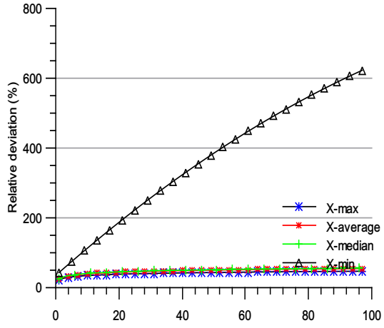
b. (m=3,n=50,d=3)
