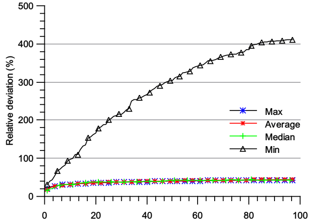
b. (m=3,n=50,d=3)
