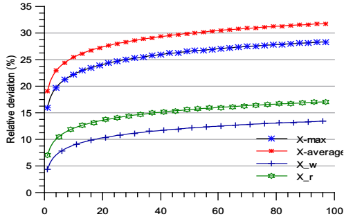
a. (m=15,n=200,d=2)
