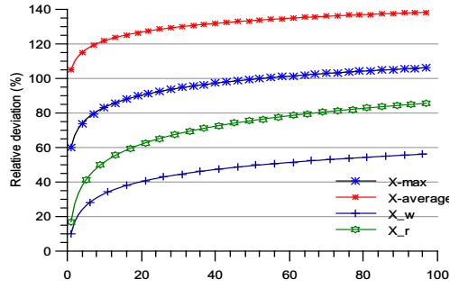
a. (m=15,n=15,d=3)
