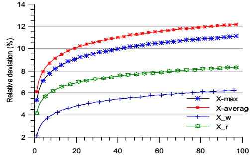
b. (m=15,n=50,d=1)
