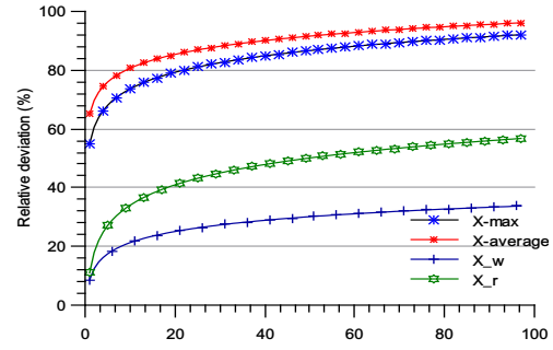
b. (m=15,n=50,d=3)
