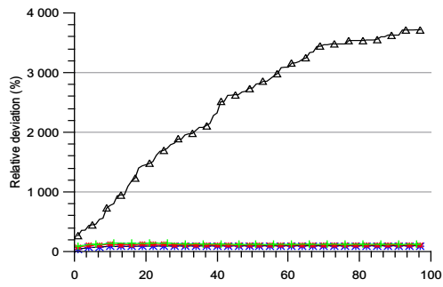
a. (m=15,n=15,d=3)
