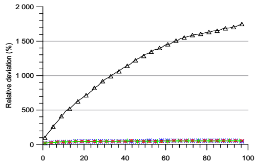
c. (m=15,n=200,d=3)
