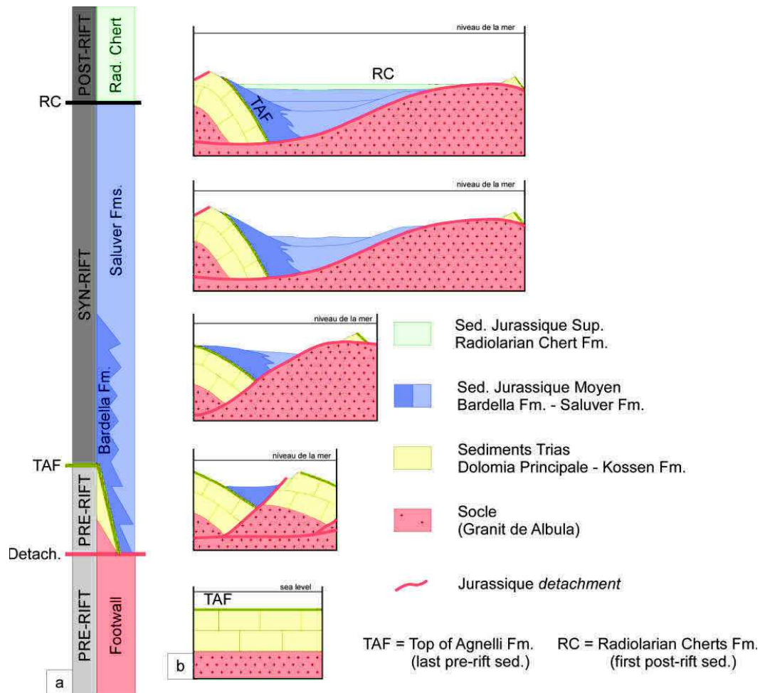
Fig. 2 - (a) Représentation schématique de la stratigraphie d'un supra-detachement basin de la marge distale Adriatique. (b) Evolution tectono-stratigraphique du bassin étudié dans cette thèse dans l'intervalle entre TAF et RC. Modifié après Masini et al. (2011, 2012).
